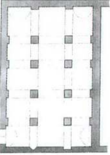
Şekil 35. Zigana Köyü Kervansaray Planı
