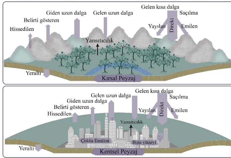
Şekil 3. Kırsal ve kentsel peyzaj üzerinde radyasyon ve enerji akıları (okların genişliği akı göreceli boyutuna yakın olarak uyarlanmıştır) (Oke 1978; Hasyim 2008'den değiştirilerek)
