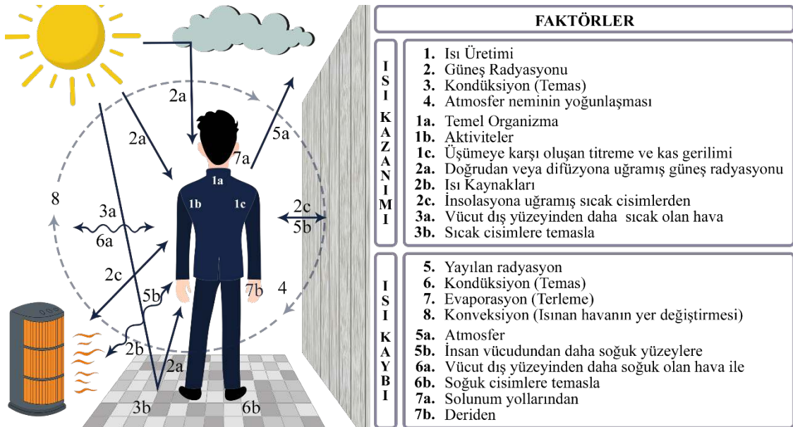
Şekil 4. İnsan vücudunda ısı kazanımı ve kaybı faktörleri (Olgyay,1973; Çınar, 1999'dan geliştirilmiştir)
