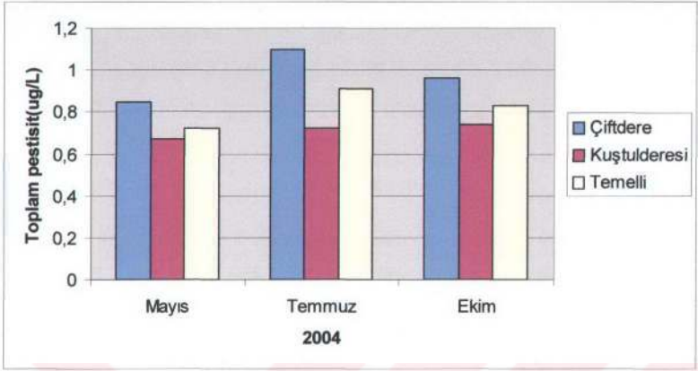
Şekil 46: İstasyonlarda aylara göre ölçülen toplam pestisit değerlerinin değişimi
