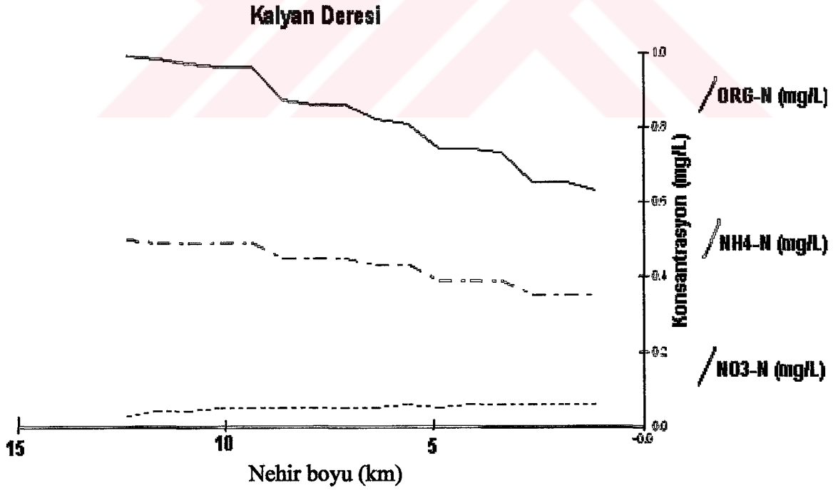
Şekil 50: Nehir boyunca NO 3 -N, NH 4 -N ve ORG-N değerlerinin değişimi
