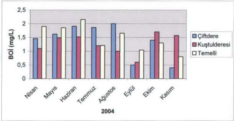
Şekil 37: İstasyonlarda aylara göre ölçülen BOİ değerlerinin değişimi
