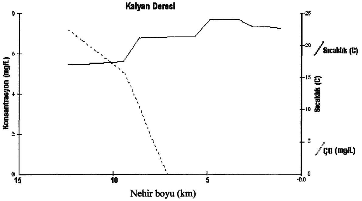
Şekil 49: Nehrin değişen sıcaklık - ÇO değerleri
