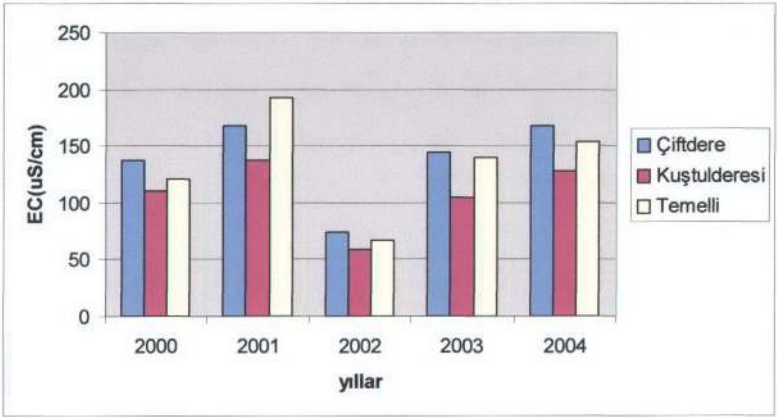
Şekil 16: Yıllara göre ortalama elektriksel iletkenlik değerlerinin karşılaştırılması
