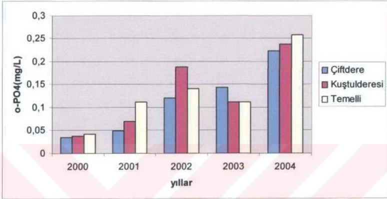
Şekil 31: Yıllara göre ortalama \text{o-PO}_4^{-3} değerlerinin karşılaştırılması
