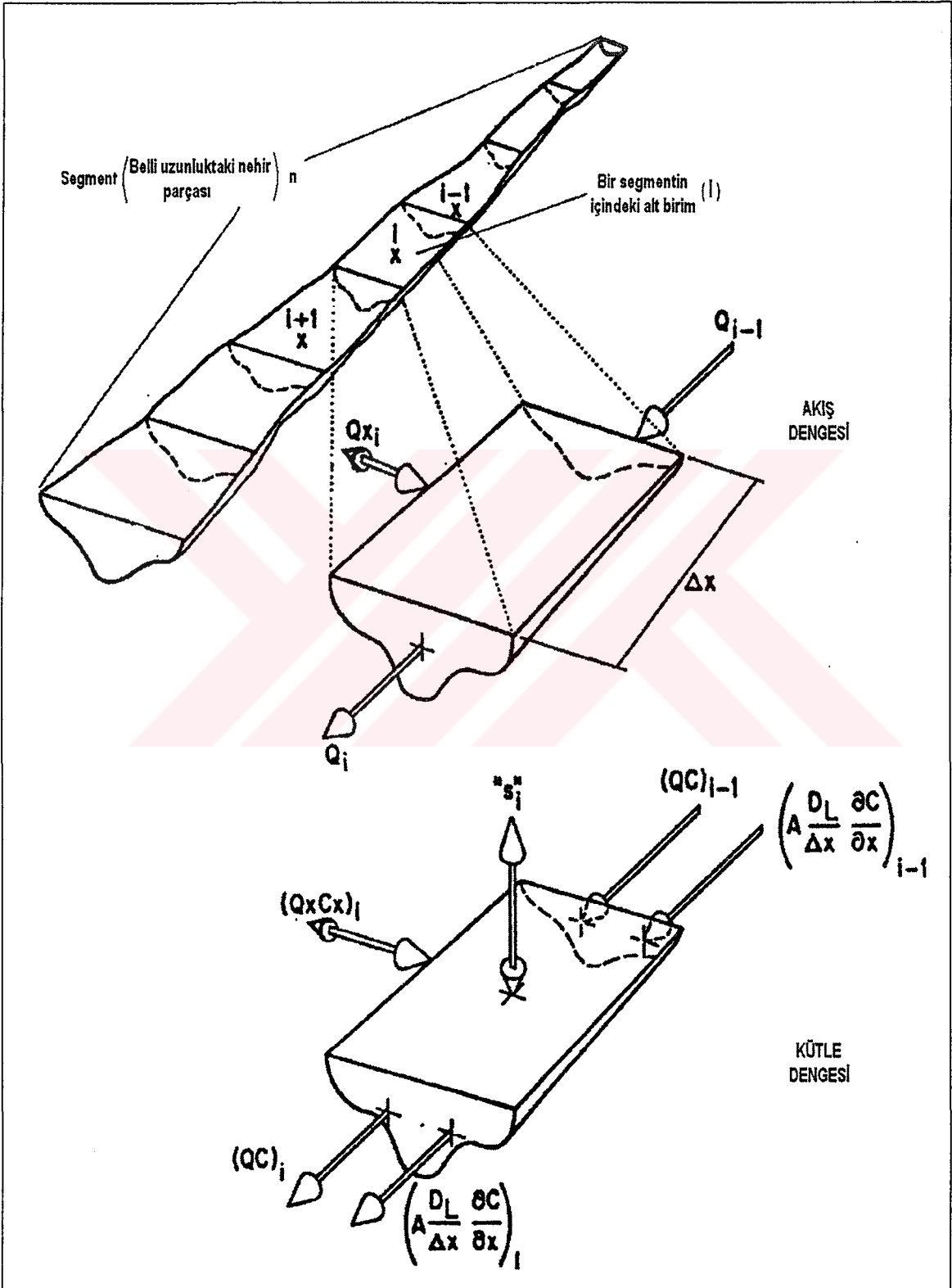
Şekil 5. Bir nehir sistemindeki akış ve kütle dengeleri
