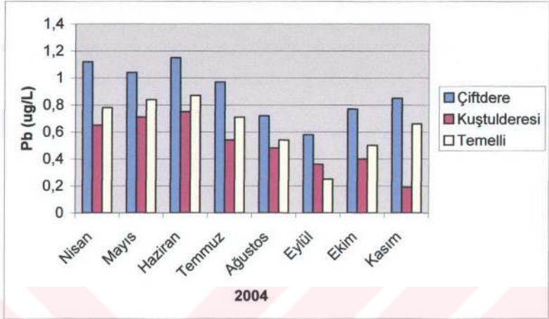
Şekil 42: İstasyonlarda aylara göre ölçülen Pb değerlerinin değişimi
