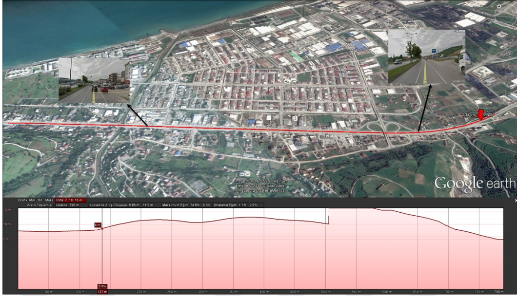
Resim 5.2 Yol kesim no 300-18, 31442, 31443, 31444 ve 31445 no'lu segmentlere ait yatay ve düşey yol geometrileri ve yol görüntüleri.
