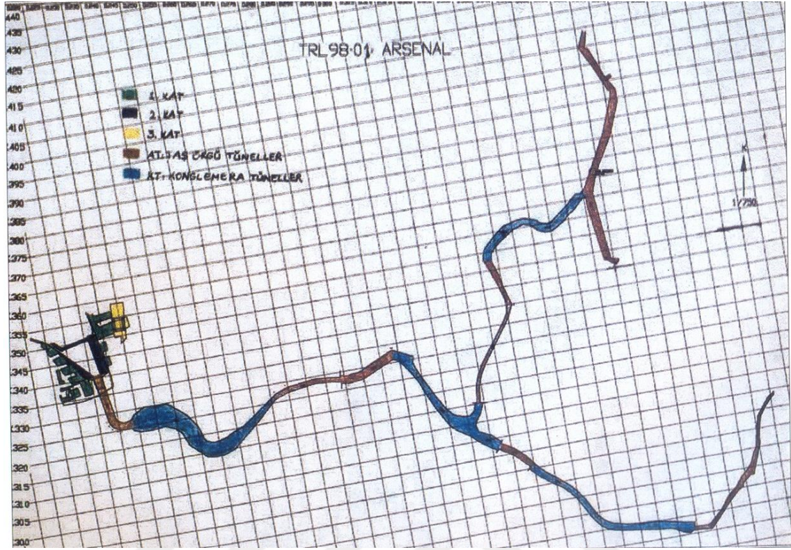
Çizim 3. Arsenel tünel ağı taban planı (Dinç, 2003c, Fig. 20, 27).
