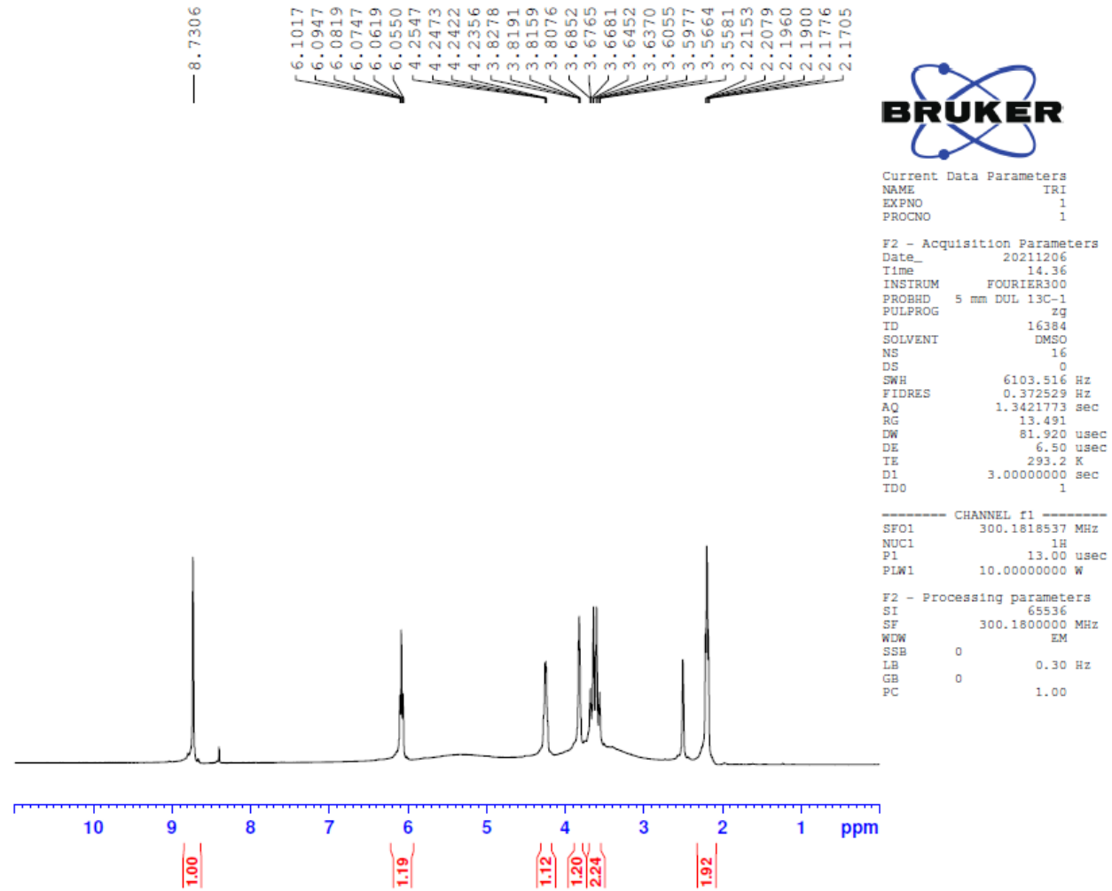
Şekil 5.3. TRI için alınmış ^1\text{H} NMR spektrumu
