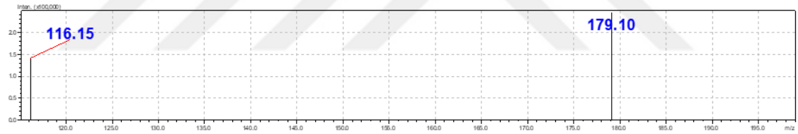
Şekil 5.14. TRI etken maddesi LC-MS/MS Spektrumu (Negatif Mod)
