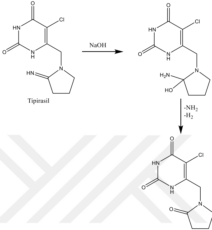
Şekil 5.29. TIP'in NaOH ortamda meydana gelen bozunma reaksiyonu
