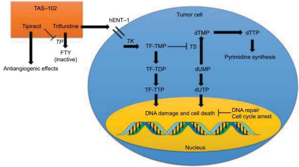
Şekil 2.3. Tipirasil HCl ve Trifluridin etki mekanizması (28)
