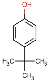
4-tert-butylphenol
