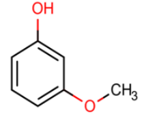
3-Methoxyphenol
