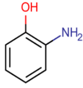
2-Aminophenol
