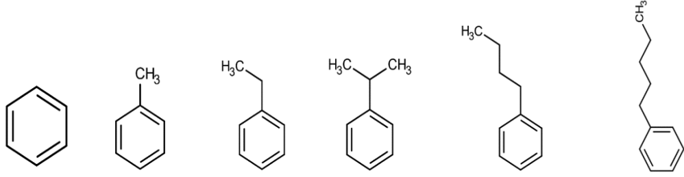
Benzene Toluene Ethylbenzene Cumene Butylbenzene Pentylbenzene
