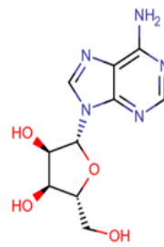
Adenosine
