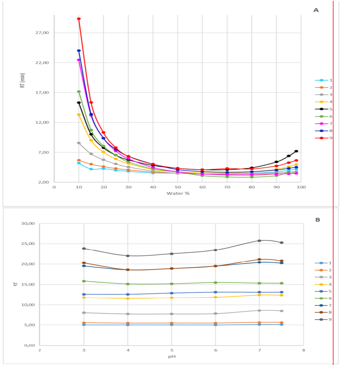
Şekil 4.5. Mobil faz içeriğinin (A) ve pH'ın (B) THMA-Mix sabit fazında nükleobazların/nükleozitlerin ayrılması üzerindeki etkisi. Koşullar: (A) ACN/su, 1,0 mL/dak, 20 °C, (B) ACN/tampon:90/10 (10 mM format, asetat veya fosfat tamponları), 1,0 mL/dak, 20 °C, 2 µL, 265 nm. Analitler: 1; timin, 2; urasil, 3; uridin, 4; adenozin, 5; adenin, 6; sitozin, 7; sitidin, 8; guanin, 9; guanozin.
