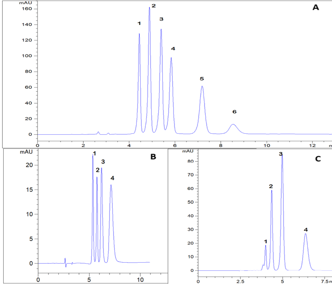
Şekil 4.6. (A) alkilbenzenlerin, (B) Sudan Boyalarının ve (C) THMA-Mix SP'de PAH'ların ayrılması. Koşullar: (A): ACN/su: 33/67, 1ml/dk, 20 0C, 1,5 µL, 210 nm. Analitler: 1; benzen, 2; toluen, 3; etilbenzen, 4; kümen, 5; bütilbenzen, 6; Pentilbenzen. (B): ACN/su gradyanı: 35/65-70/30, 0-10 dk., 1 ml/dk, 40 0C, 2 µl, 520 nm. Analitler: 1; Sudan I, 2; Sudan II, 3; Sudan III, 4; Sudan IV. (C): ACN/su: 41/59, 20 0C, 1 ml/dk, 254 nm, 1,5 µl. Analitler: 1; Naftalin, 2; Floren, 3; Antrasen, 4; Benzantrasen.
