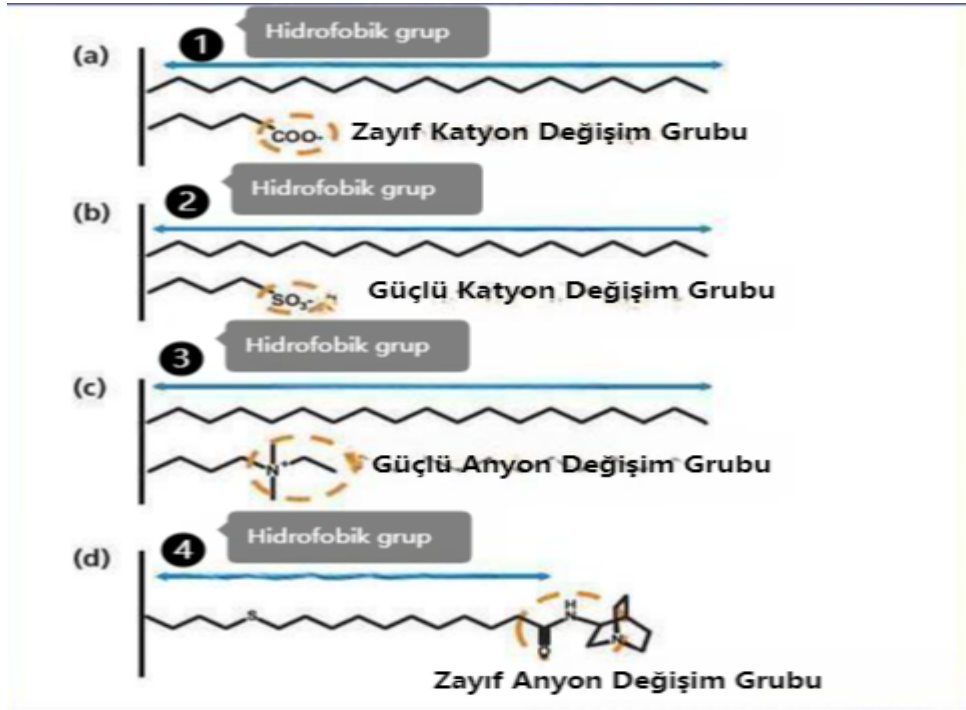
Şekil 1.2. (a) Zayıf kation değişim grubu içeren ters fazlı karma mod sabit faz, (b) güçlü kation değişim grubu içeren ters fazlı karma mod sabit faz, (c) güçlü anyon değişim grubu içeren ters fazlı karma mod sabit faz ve (d) zayıf anyon değişim grubu içeren ters fazlı karma mod sabit faz.
