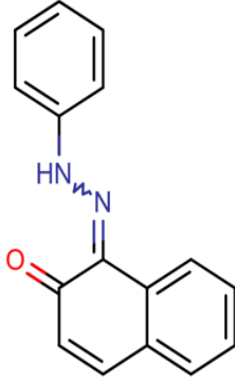
Sudan I
