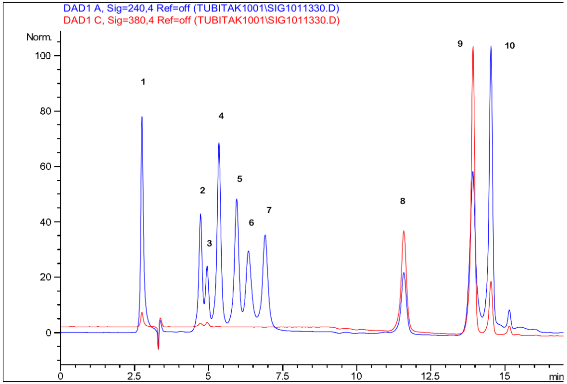
Şekil 4.8. THMA-Mix SP'de Anilinlerin Ayrılması. Koşullar: Sulu tampondaki ACN gradyanı (pH:5.00, 10 mM, Amonyum asetat): %3; 0-5 dak, %40; 5-15 dak, 1 ml/dak., 20 °C, 2 µl, 240 ve 380 nm
