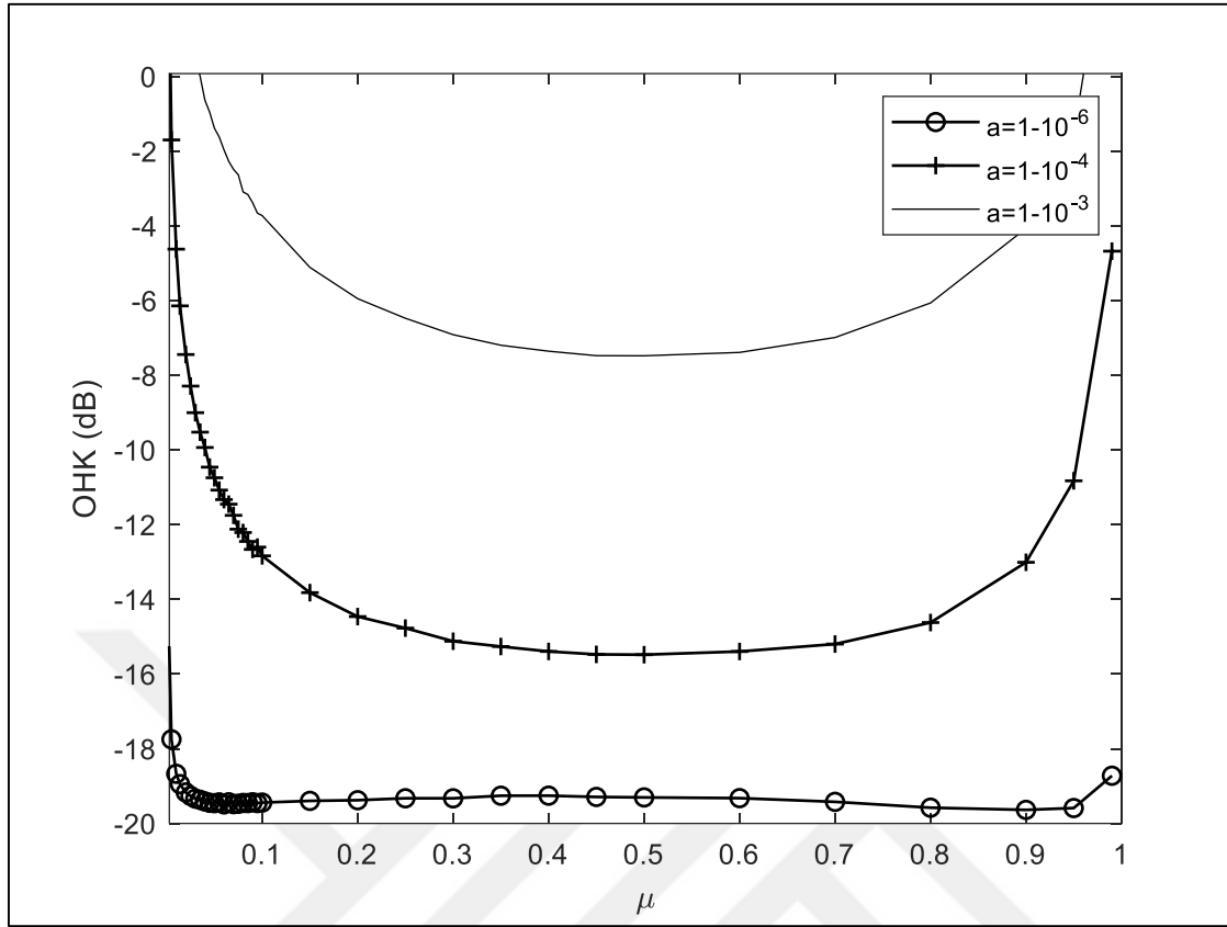
Şekil 4.7. FB-RLS kanal kestirim algoritması takip performansı
