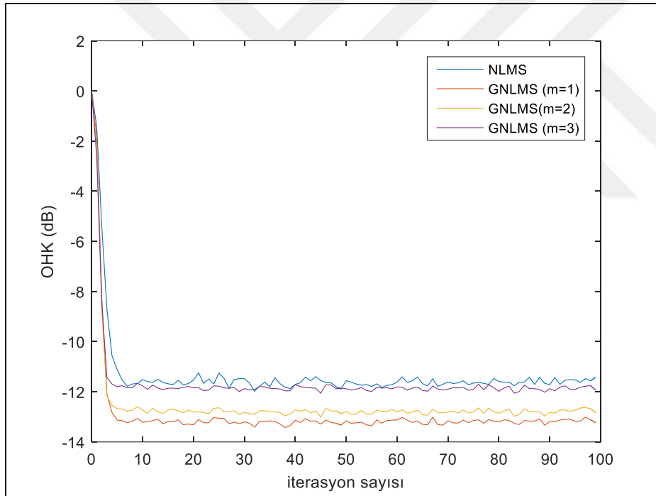
Şekil 3.11. GNLMS algoritmasında farklı projeksiyon seviyeleri için elde edilen öğrenme eğrisi performansları, f_D=5.56\text{Hz} , E_b/N_0=20\text{dB} , BPSK, N_{\text{sym}}=128 , \mu=0.9
