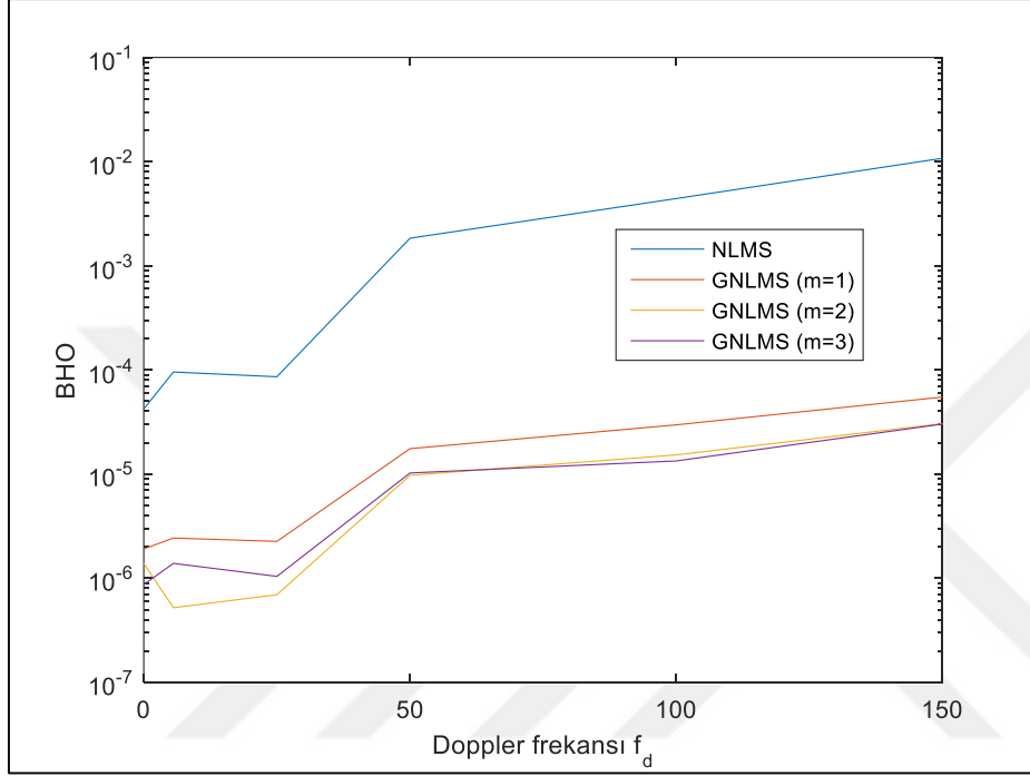
Şekil 3.12. GNLMs algoritmasında farklı projeksiyon seviyeleri için Doppler frekansına göre BER değişimi, f_D=5.56\text{Hz} , E_b/N_0=20\text{dB} , BPSK, N_{\text{sym}}=256 , \mu=0.9
