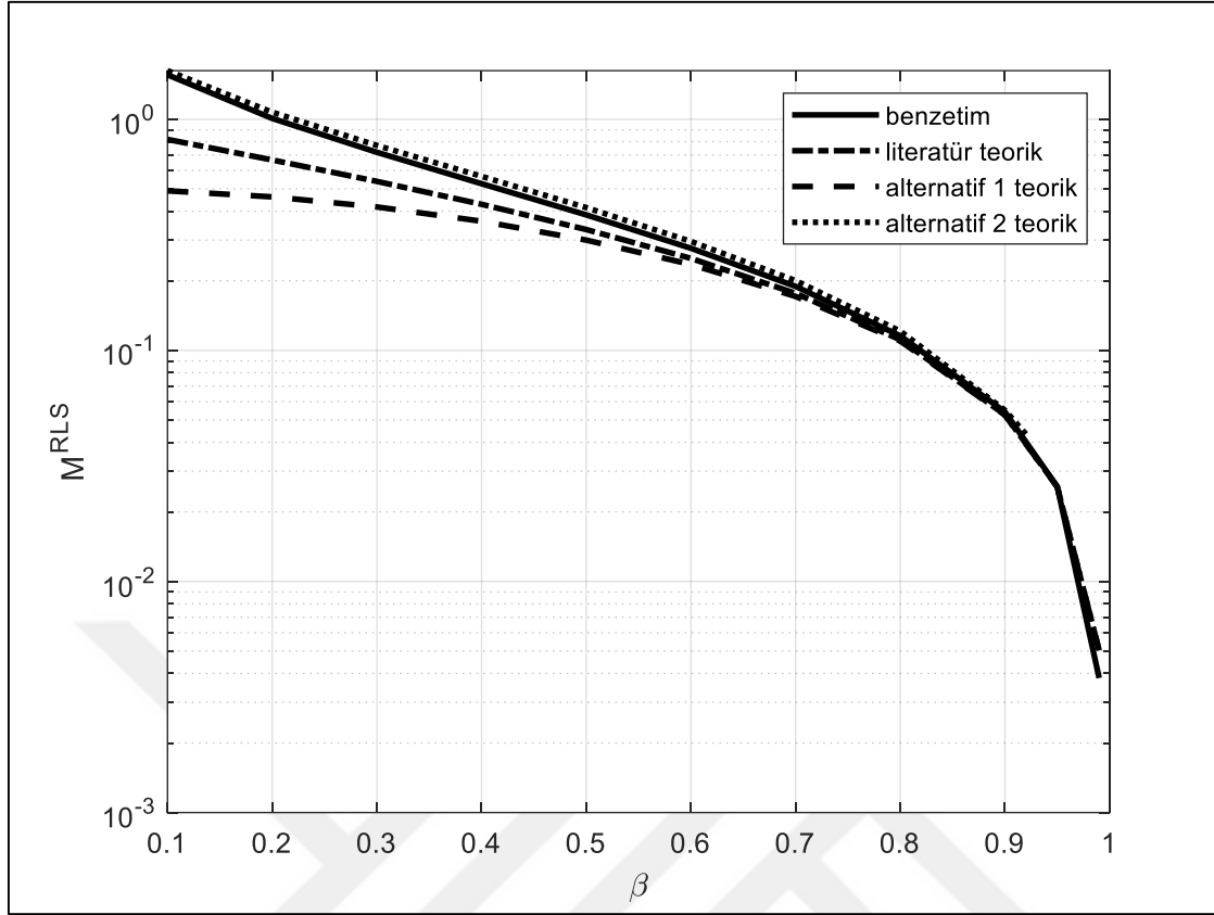
Şekil 2.8. RLS algoritması ayarsızlık değerinin unutma faktörüne göre değişimi
