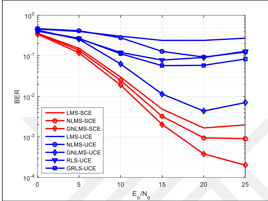
Şekil 4.2. Uyarlanabilir kanal kestirim BHO sonuçları, v=150\text{km/h}
