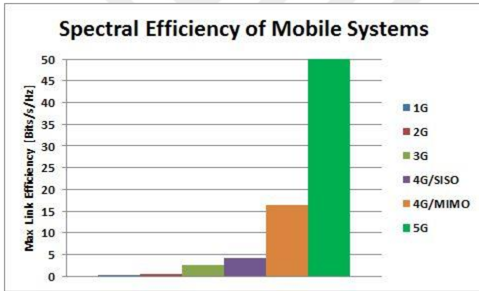
Şekil 1.1. Mobil haberleşme sistemlerinde spektrum verimliliği
