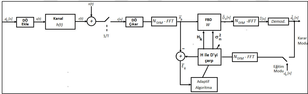
Şekil 4.1. TT-FBD uyarlanabilir kanal kestirim algoritması kullanan sistem modeli
