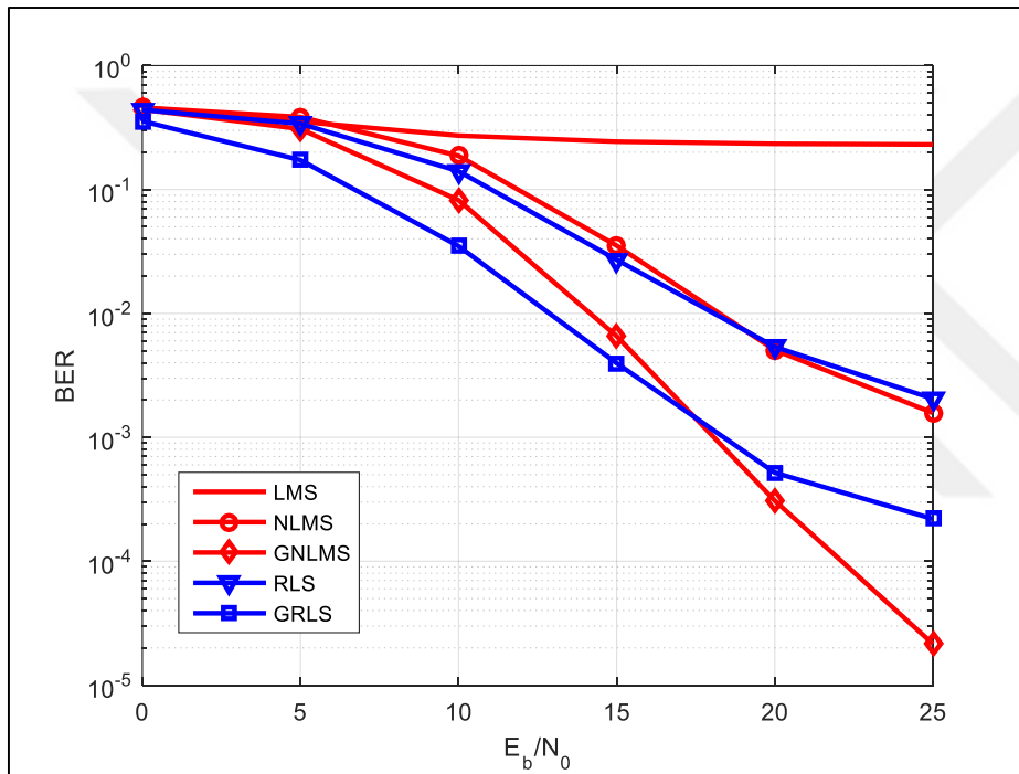
Şekil 3.5. GNLMs ve GRLS algoritmalarının BHO performansları, v=75\text{km/s}
