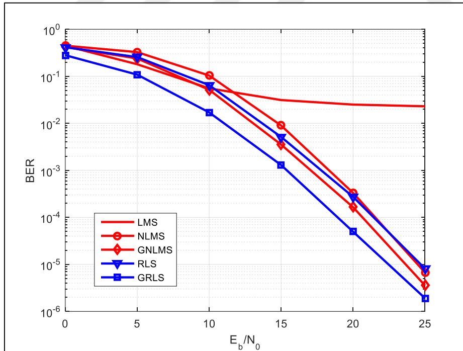
Şekil 3.4. GNLMS ve GRLS algoritmalarının BHO performansları, v=25\text{km/s}
