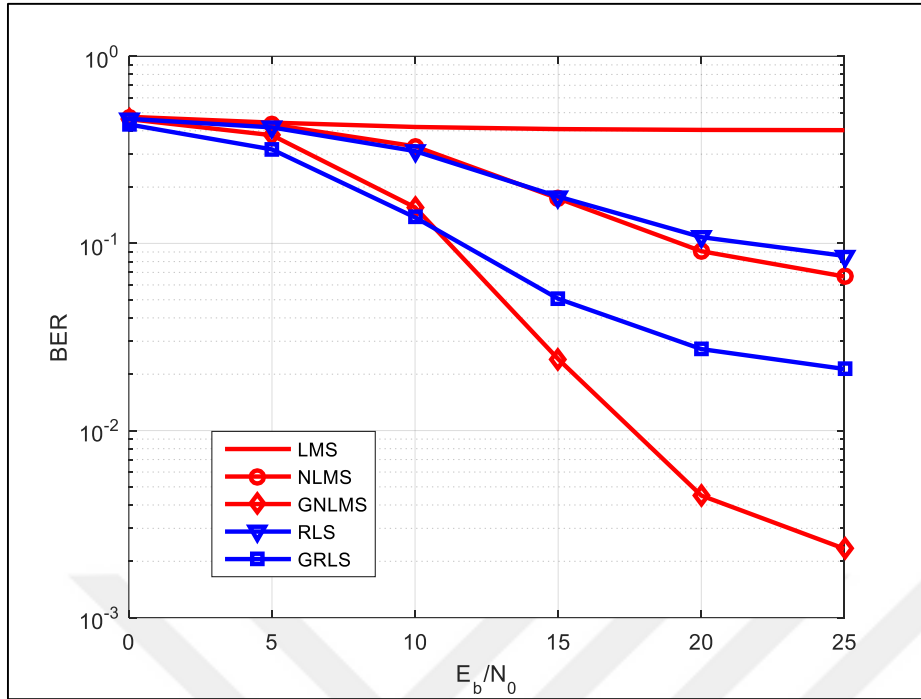
Şekil 3.6. GNLMs ve GRLS algoritmalarının BHO performansları, v = 150 \text{ km/s}
