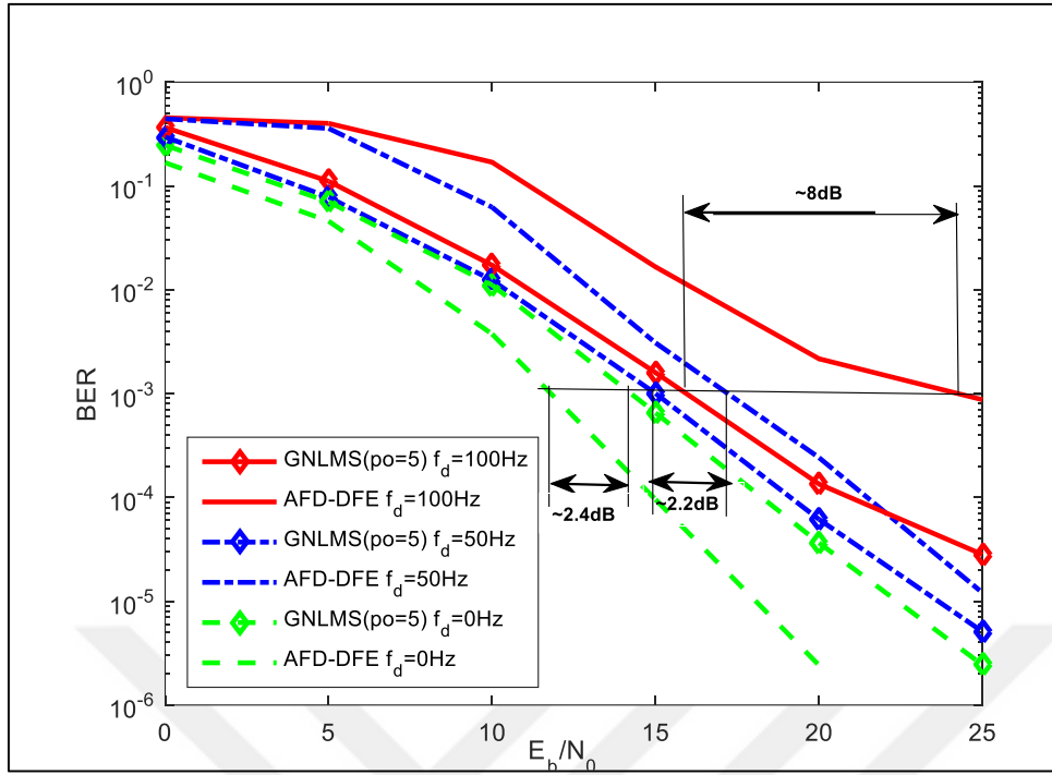
Şekil 5.2. AFD-DFE ile GNLM algoritmalarının BHO performansları
