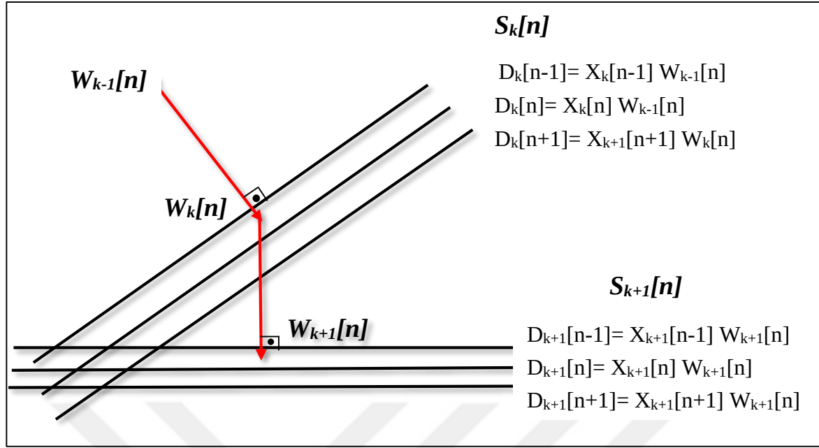
Şekil 3.2. GNLMS algoritmasında katsayı güncellemesi, GNLMS algoritması p_o=3
