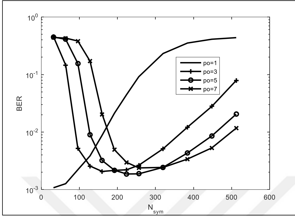
Şekil 3.9. GNLMS algoritmasında farklı projeksiyon seviyeleri için elde edilen BHO performansları, f_D=100\text{Hz} , E_b/N_0=15\text{dB}
