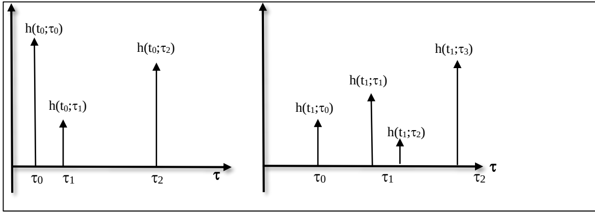
Şekil 1.6. Zamanla kanal birim dürtü tepkisinin değişimi
