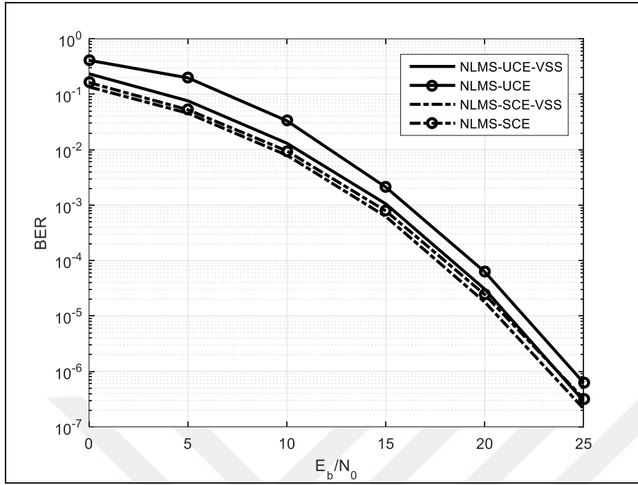
Şekil 4.3. Sabit ve değişken katsayılı uyarlamalı kanal kestirim BHO sonuçları, v=3\text{km/h}
