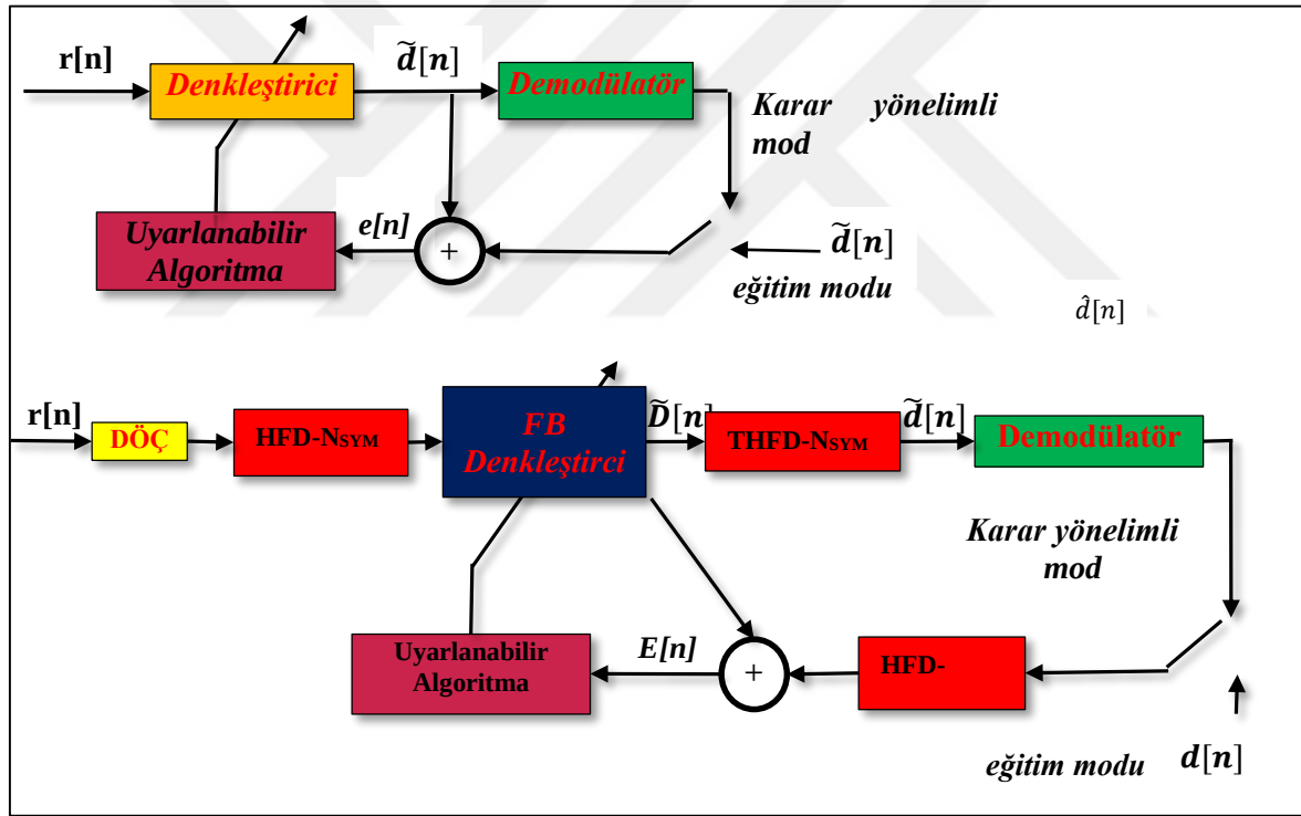
Şekil 2.1. TT-FBD için (a) ZB (b) FB'de çalışan uyarlanabilir denkleştirici yapıları
