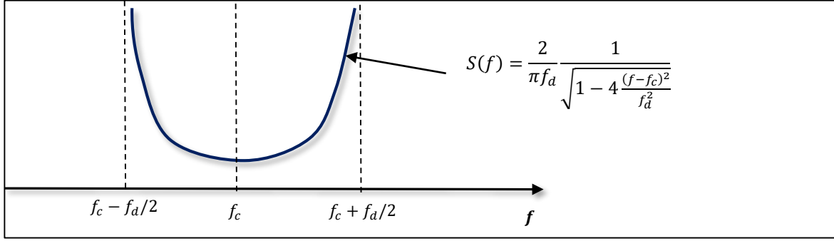
Şekil 1.5. Doppler frekans kayması
