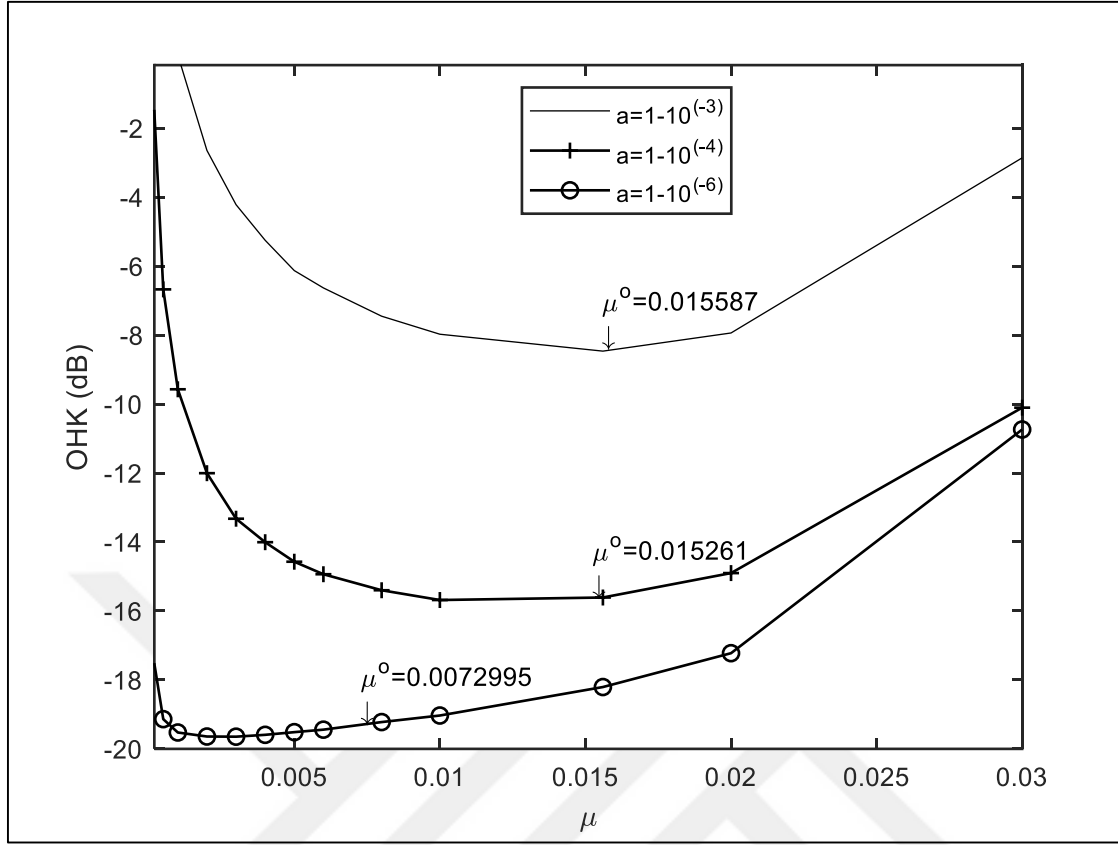
Şekil 4.5. FB-LMS kanal kestirim algoritması takip performansı
