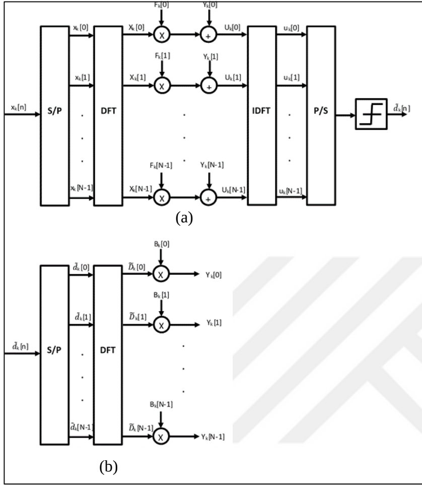
Şekil 5.1. Uyarlanabilir frekans bölgesi karar geri besleme denkleştirici sistemi (a) doğrusal, (b) geri besleme kısmı
