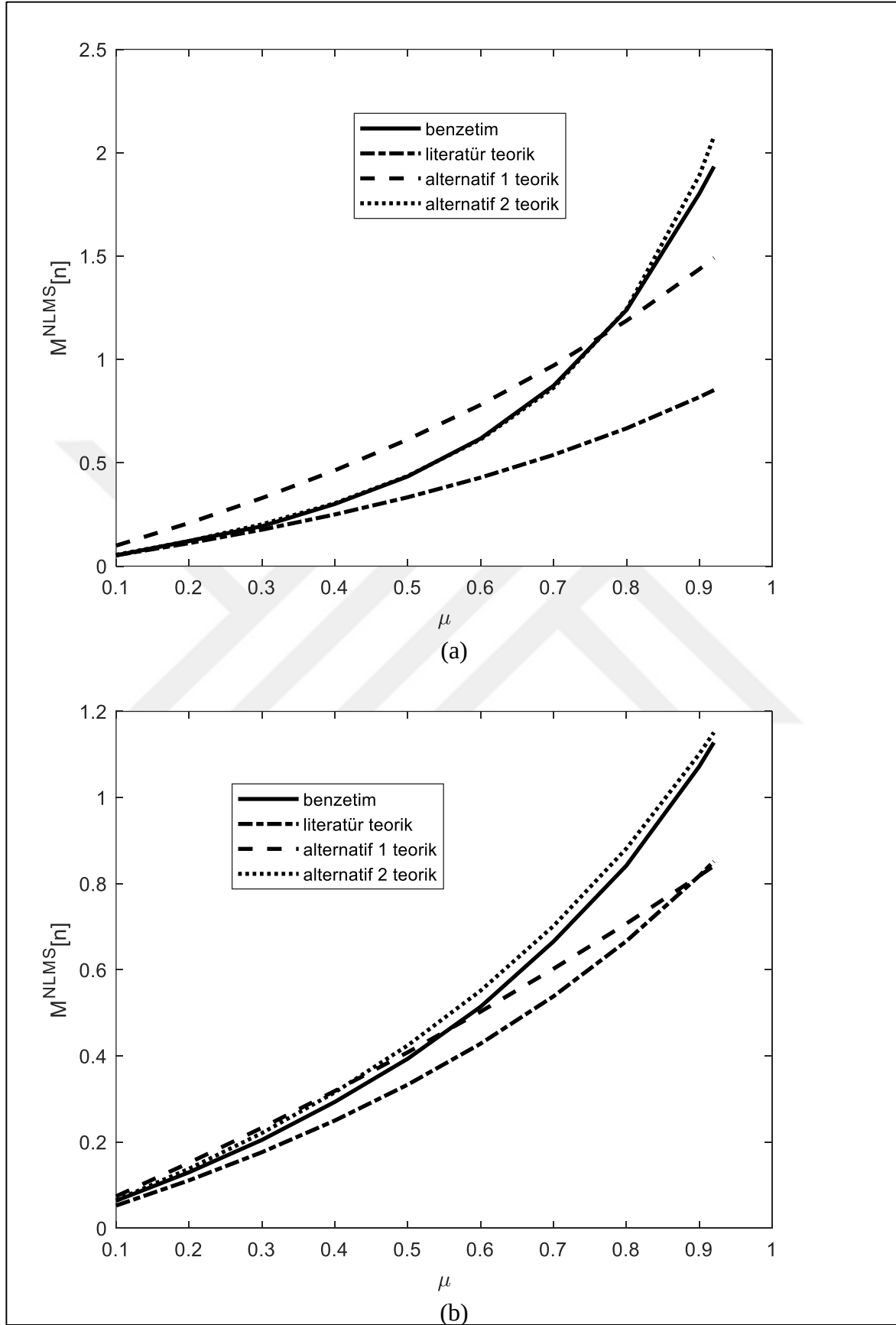
Şekil 2.6. FB-NLMS algoritması ayarsızlık değerinin \mu 'ya göre değişimi (SGO=20dB) (a) \gamma = 0.1 , (b) \gamma = 0.45 , (c) \gamma = 0.9
