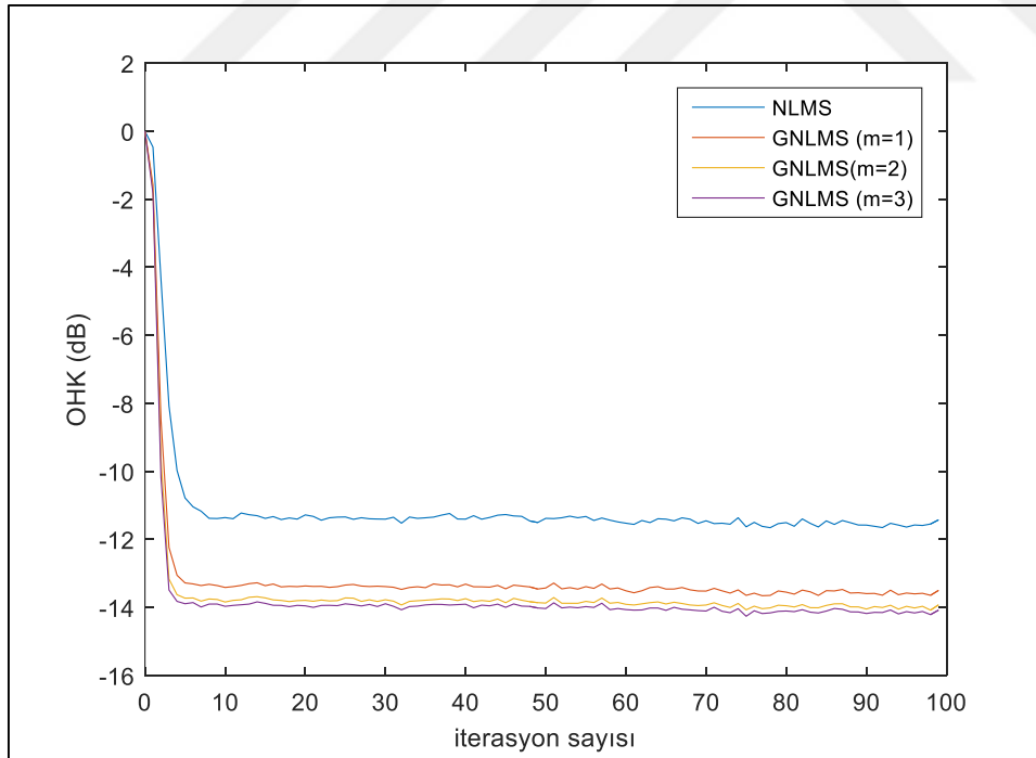
Şekil 3.10. GNLMS algoritmasında farklı projeksiyon seviyeleri için elde edilen öğrenme eğrisi performansları, f_D=5.56\text{Hz} , E_b/N_0=20\text{dB} , BPSK, N_{sym}=256 , \mu =0.9
