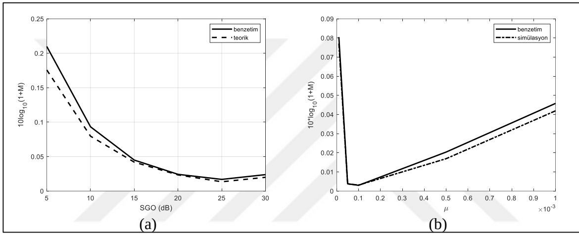
Şekil 2.4. LMS algoritması ayarsızlık değeri (a) SGO, (b) \mu 'ye bağlı değişimi
