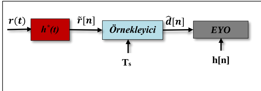
Şekil 1.10. EYO algoritması
