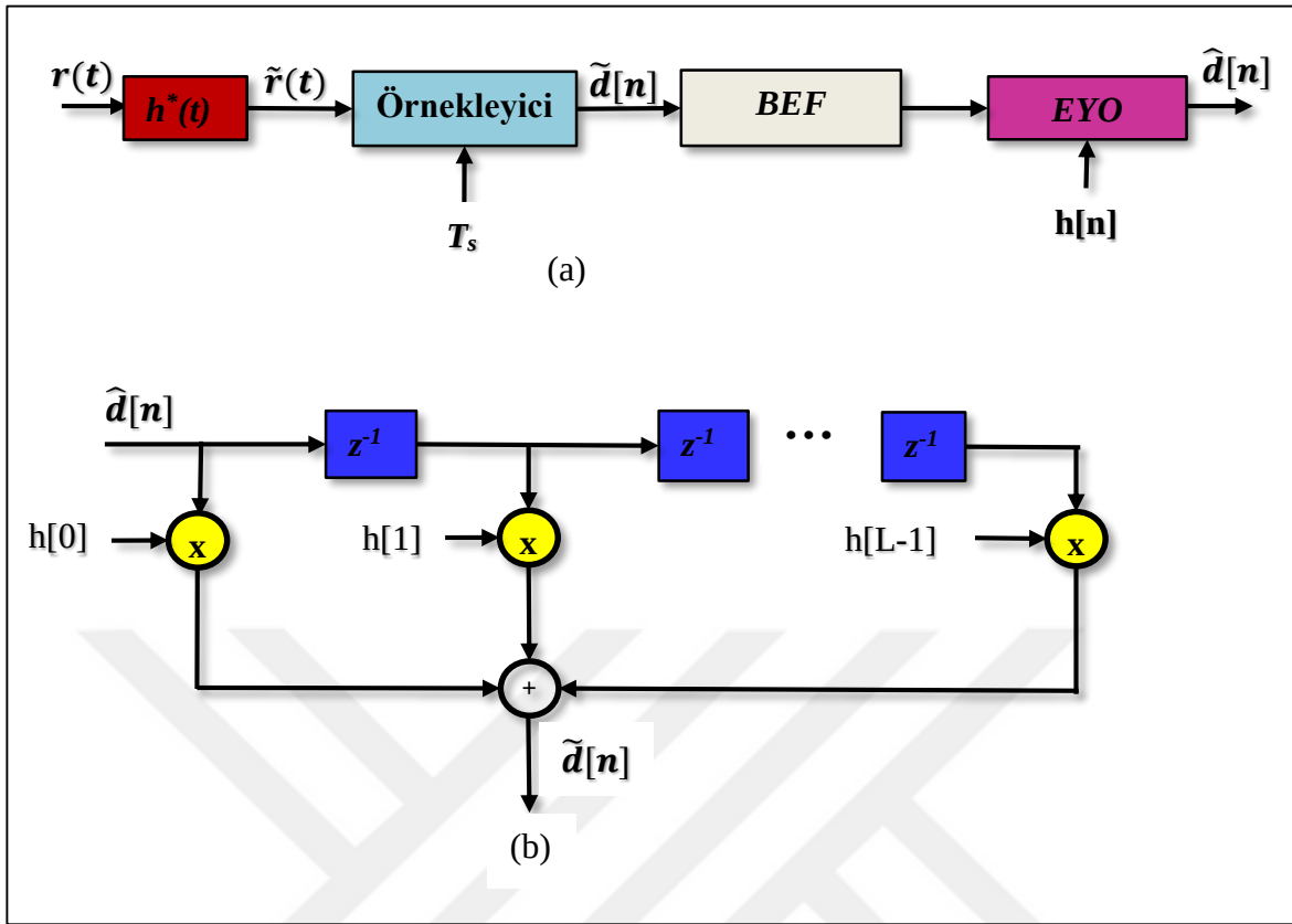
Şekil 1.11. (a) BEF kullarılan EYO alıcı yapısı (b) BEF filtre eşdeğer sayısal modeli
