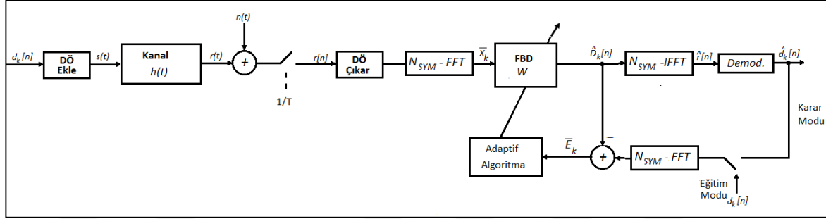
Şekil 3.1. Uyarlanabilir FBD kullanan TT-FBD alıcı-verici sistemi
