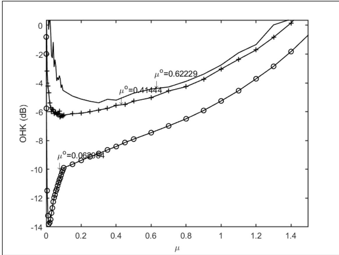
Şekil 2.9. FB-NLMS takip performansı
