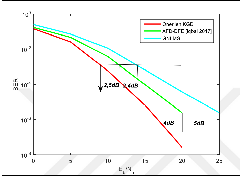
Şekil 5.4. AFD-DFE, GNLMS ve yeni önerilen KGB algoritmalarının bit hata oranı performansları
