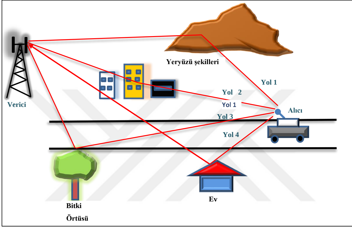
Şekil 1.2. Kablosuz haberleşme sistemlerinde çok yollu iletim
