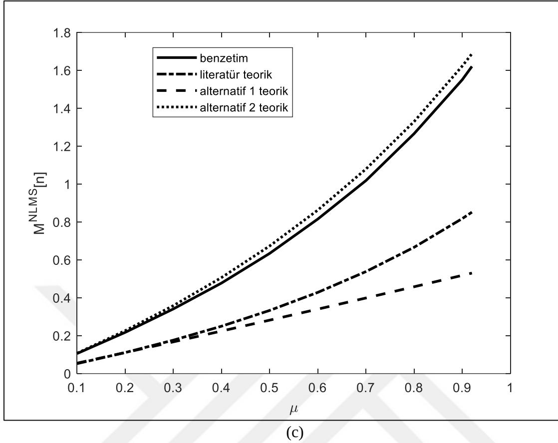
Şekil 2.6. (devam) FB-NLMS algoritması ayarsızlık değerinin \mu 'ya göre değişimi (SGO=20dB) (a) \gamma=0.1 , (b) \gamma=0.45 , (c) \gamma=0.9
