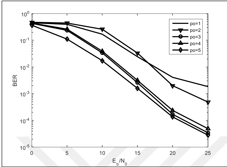
Şekil 3.8. GNLS algoritmasında farklı projeksiyon seviyeleri için elde edilen BHO performansları, f_D=100\text{Hz}
