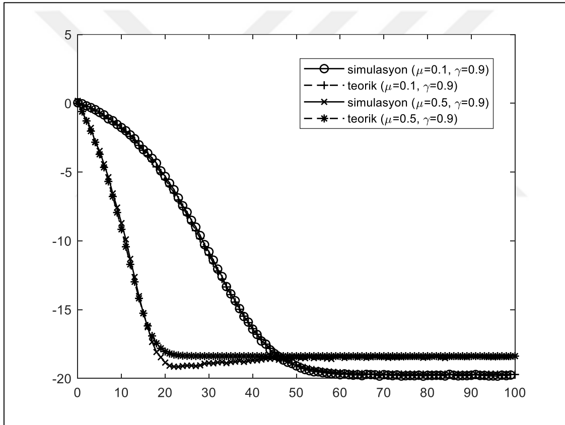
Şekil 2.7. FB-NLMS öğrenme eğrisi
