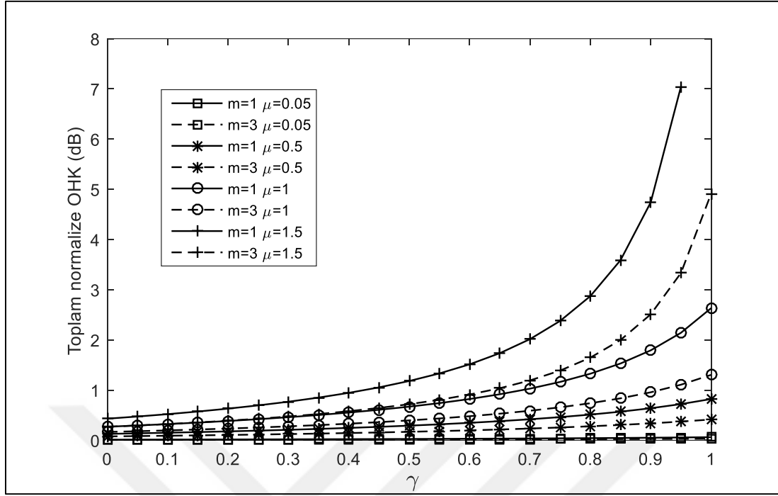
Şekil 3.3. GNLMS karalı durum normalize OHK değerin \gamma ve \mu e göre değişimi
