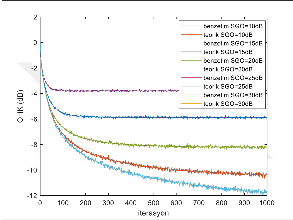
Şekil 2.3. FB-LMS öğrenme eğrileri \mu=10^{-3}
