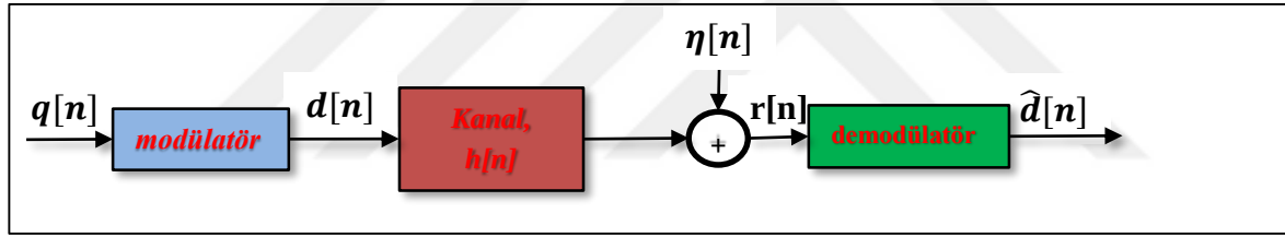
Şekil 1.3. Temel bant sayısal haberleşme sistemi
