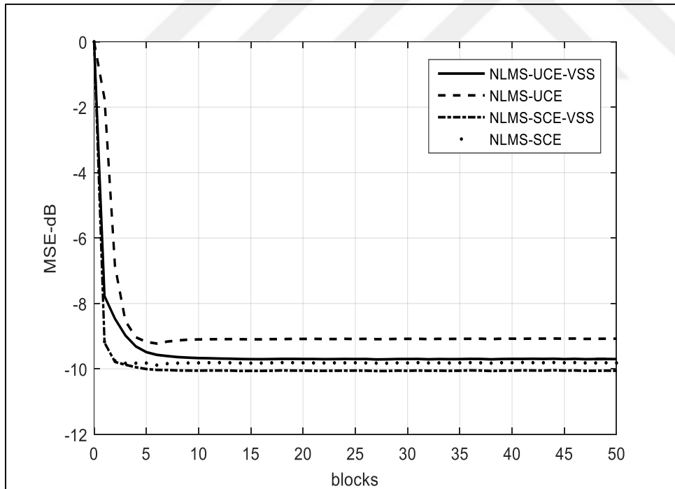
Şekil 4.4. Sabit ve değişken katsayılı uyarlamalı uyarlamalı algoritmaların öğrenme eğrisi performansları, v=3\text{km/s} , \text{SGO}=15\text{dB}
