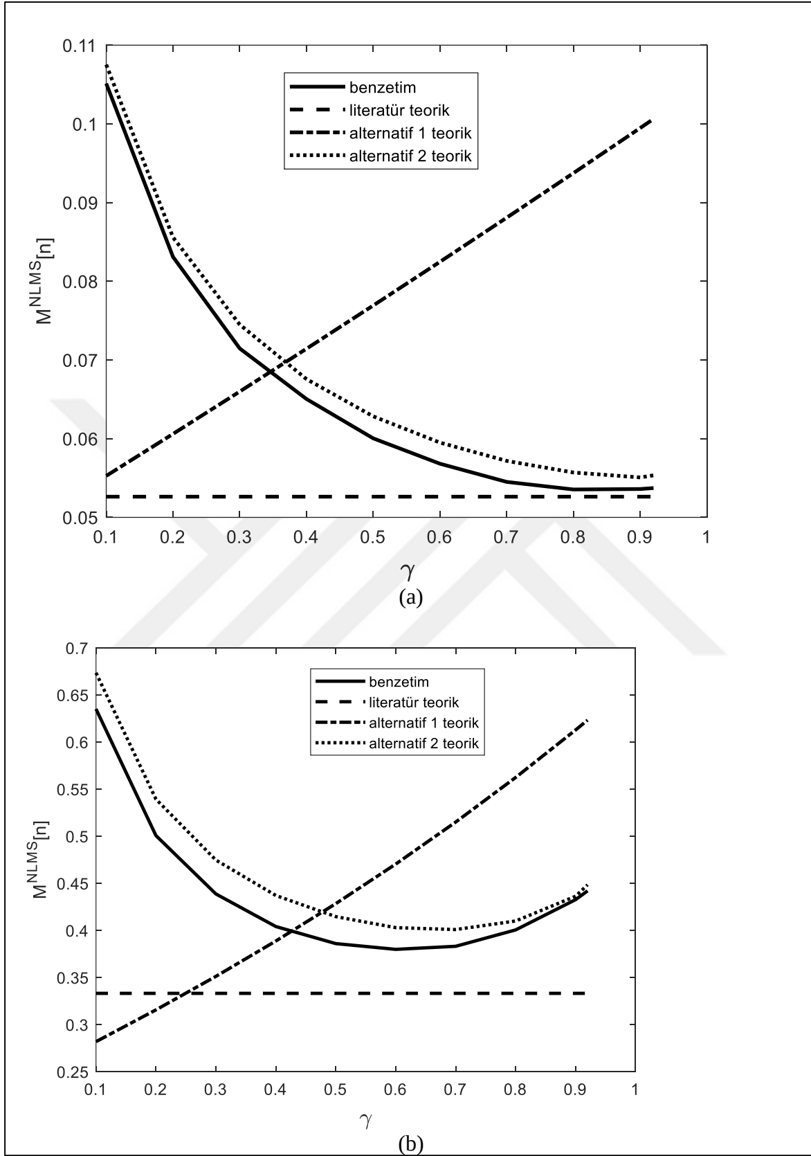
Şekil 2.5. FB-NLMS algoritması ayarsızlık değerinin unutma faktörüne göre değişimi (SGO=20dB) (a) \mu = 0.1 , (b) \mu = 0.5 , (c) \mu = 0.9
