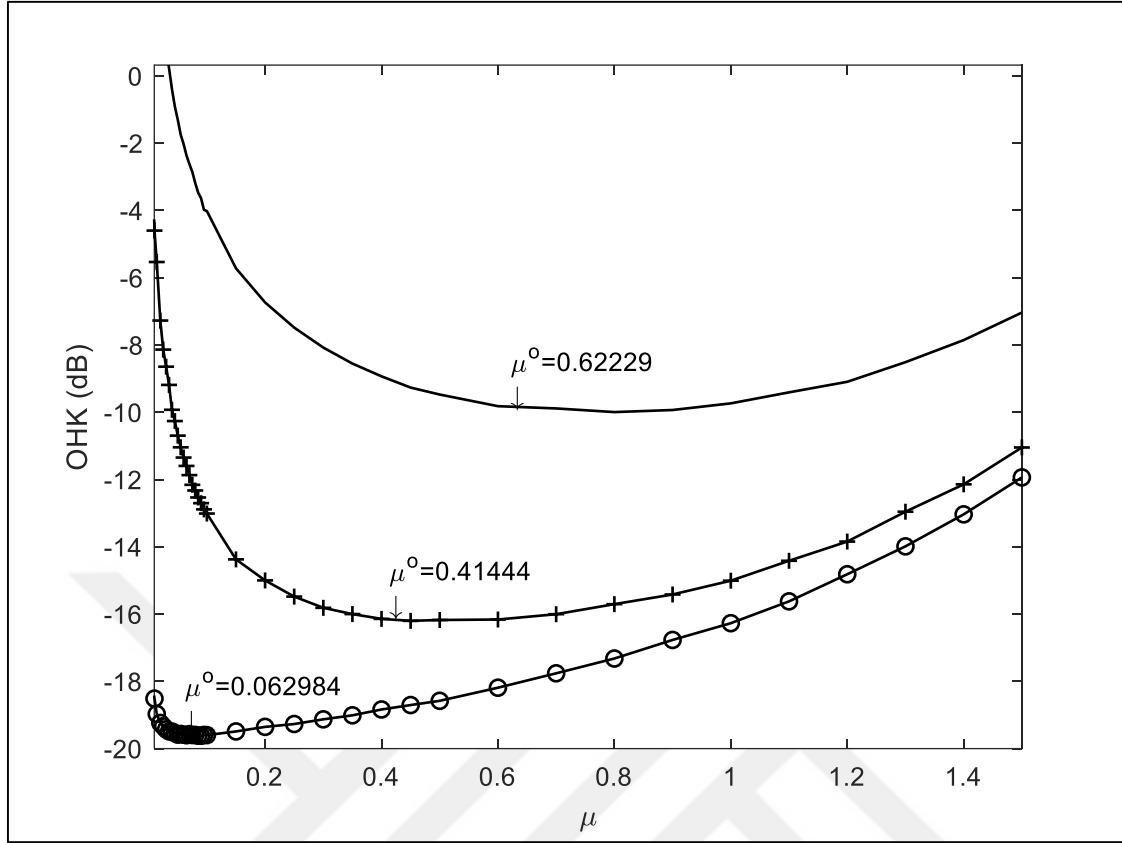
Şekil 4.6. FB-NLMS kanal kestirim takip performansı
