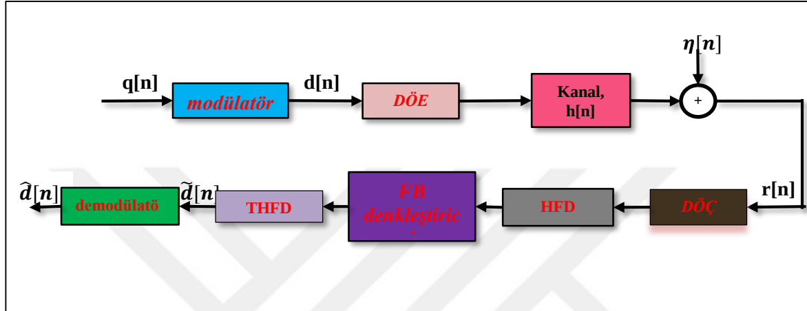
Şekil 1.13. TT-FBD alıcı verici sistemi
