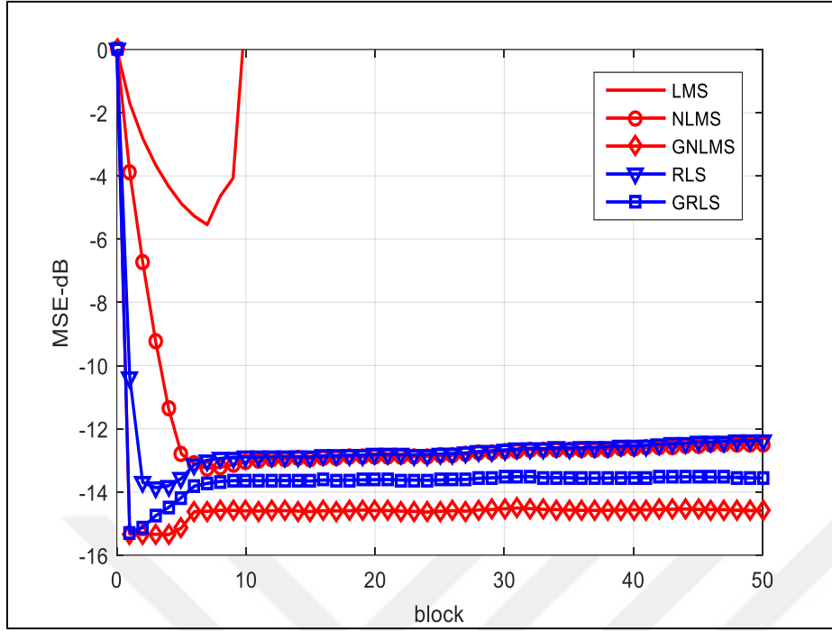
Şekil 3.7. Uyarlanabilir algoritmalarının öğrenme eğrisi performansları, v=75\text{km/h} , \text{SGO}=25\text{dB}
