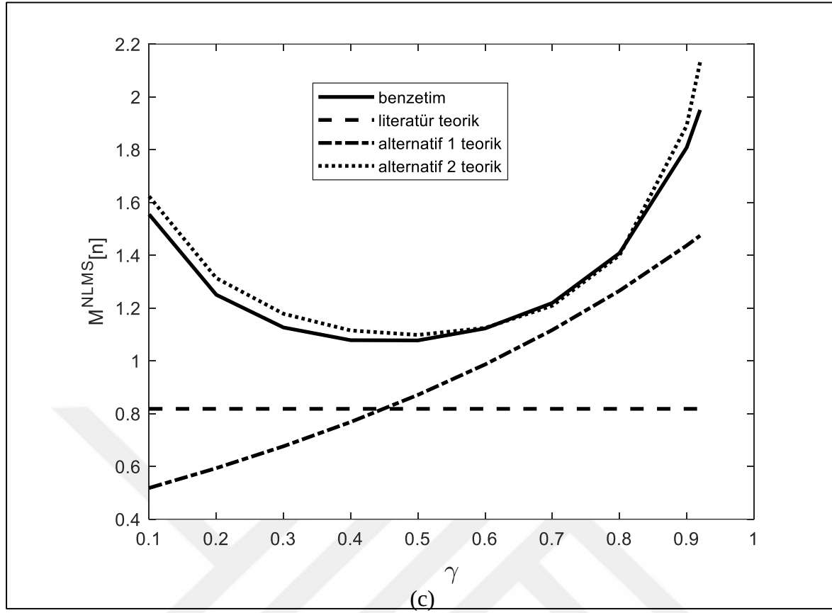
Şekil 2.5. (devam) FB-NLMS algoritması ayarsızlık değerinin unutma faktörüne göre değişimi (SGO=20dB) (a) \mu = 0.1 , (b) \mu = 0.5 , (c) \mu = 0.9
