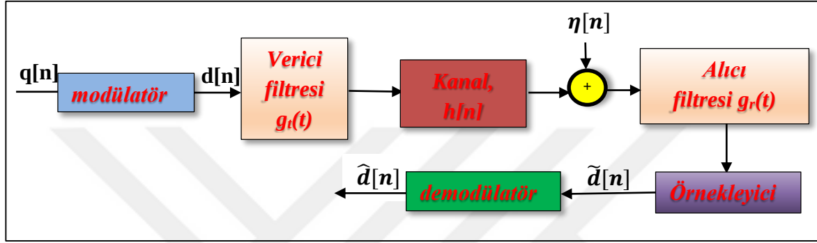
Şekil 1.9. Eşlenik filtre kullanan alıcı-verici sistemi
