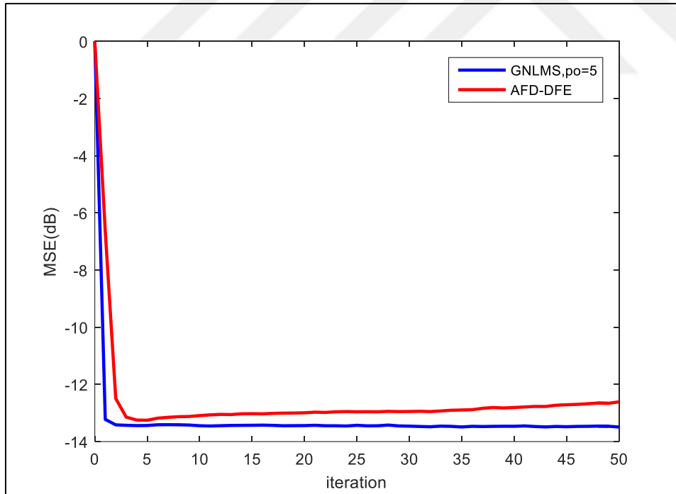
Şekil 5.3. AFD-DFE ile GNLM algoritmalarının öğrenme eğrisi performansları
