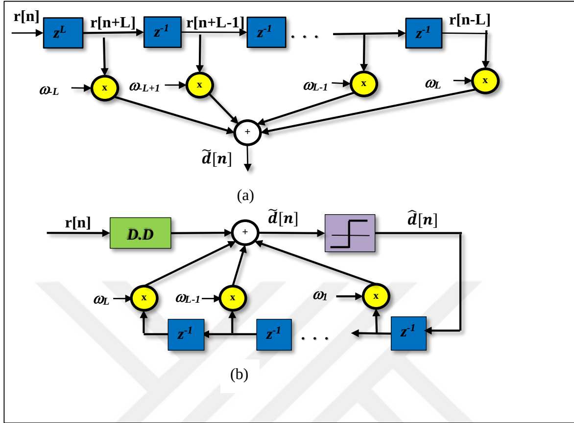
Şekil 1.12. ZB- EUAÇ denkleştirici yapıları (a) DD ve (b) KGB
