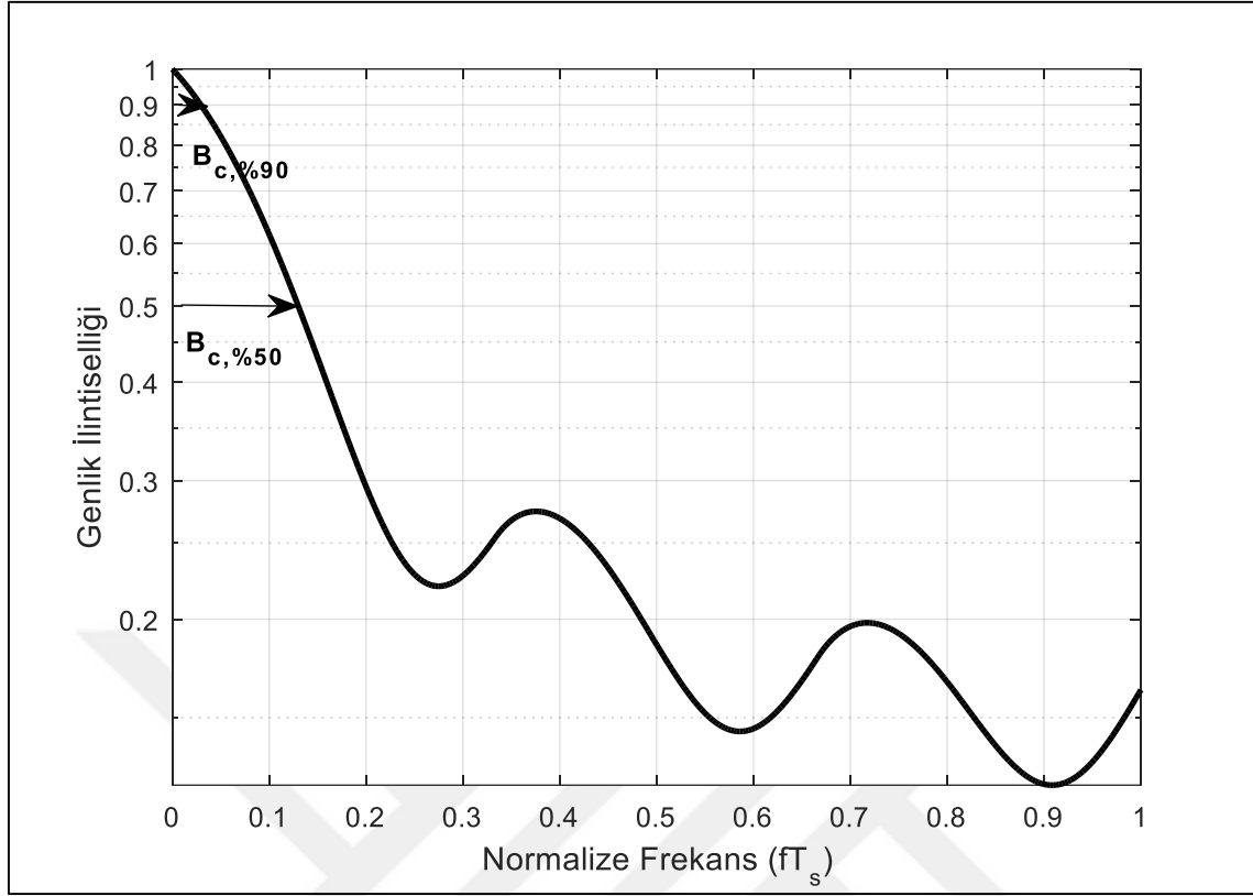
Şekil 1.8. Kablosuz haberleşme kanalı ilintiselliği
