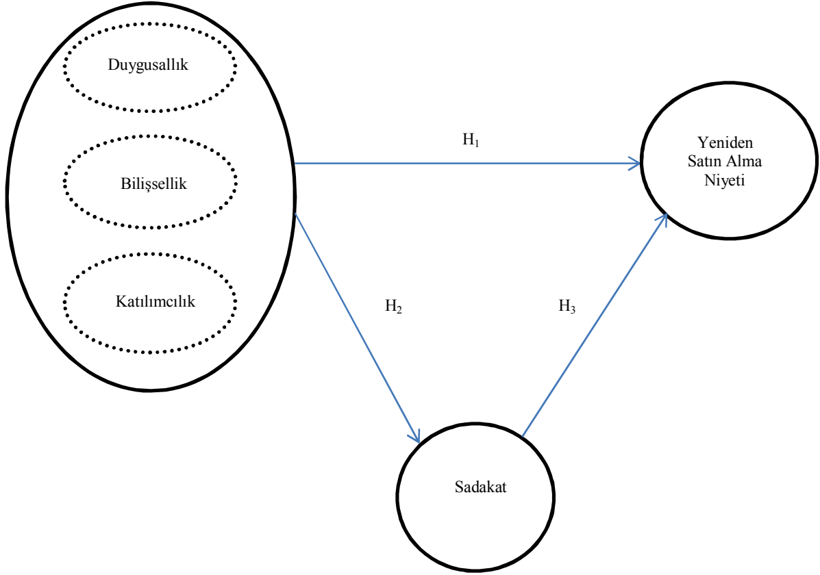
Şekil 1. Araştırma Modeli
