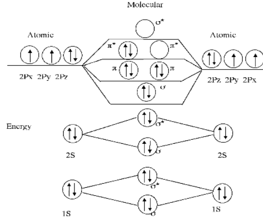
Şekil 3: Singlet oksijenin moleküler orbital şeması (42)
