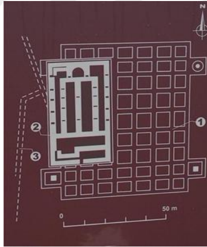
Görsel 3.17. Kurum Han İç Saray Planı
