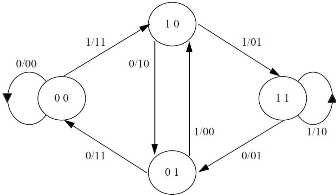
Şekil 2.2. Evrişimli Kodlayıcının Durum Gösterimi
