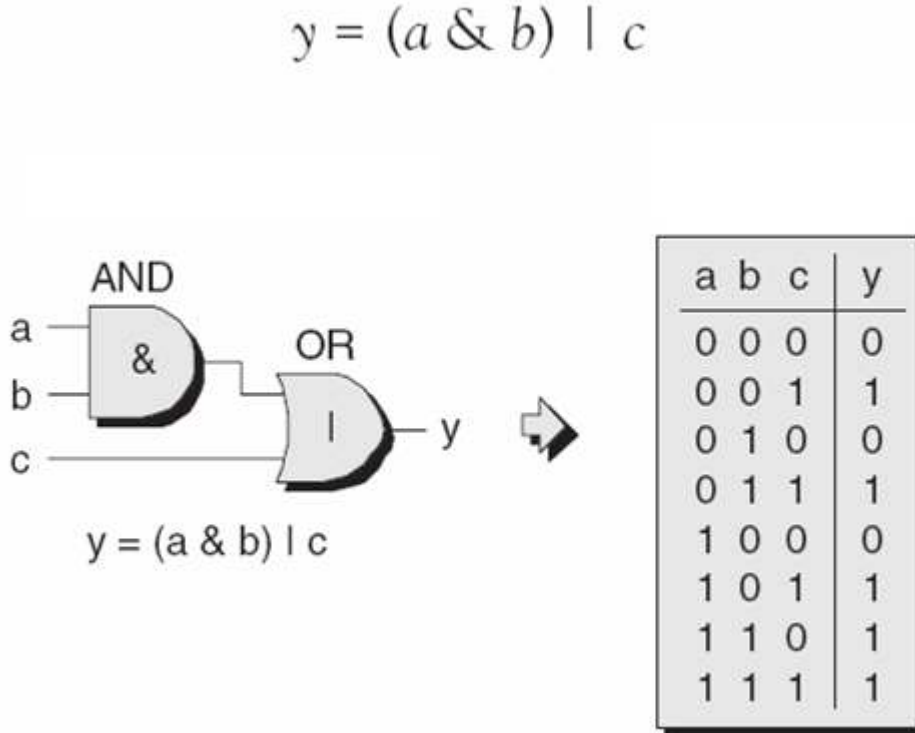
Şekil 4.6. LUT Tabanlı Hücre
