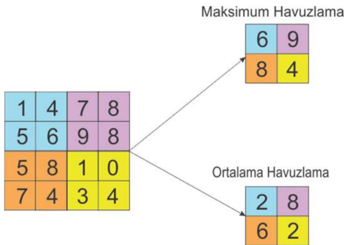
Şekil 3.17 Maksimum ve ortalama havuzlama
