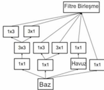
Şekil 4.3 Inception modeli-3 [43]
