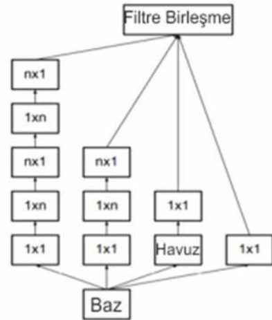
Şekil 4.2 Inception modeli-2 [43]
