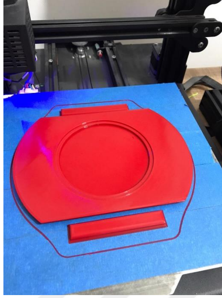
Görsel 4.13. Keskin gövdeli formun fincan tabağı, 3D baskı, Sonay Ersöyleyen fotoğraf arşivi
