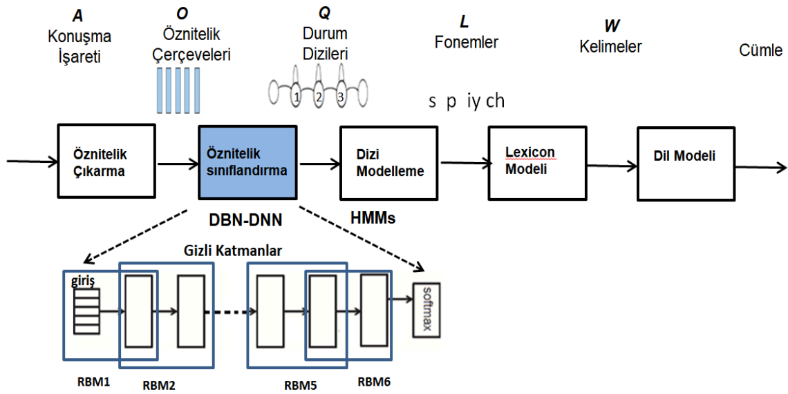
Şekil 6.8. Sistem Mimarisi
