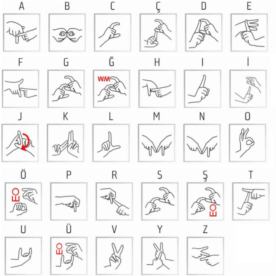
Şekil 3.1 TİD Alfabeti [50]
