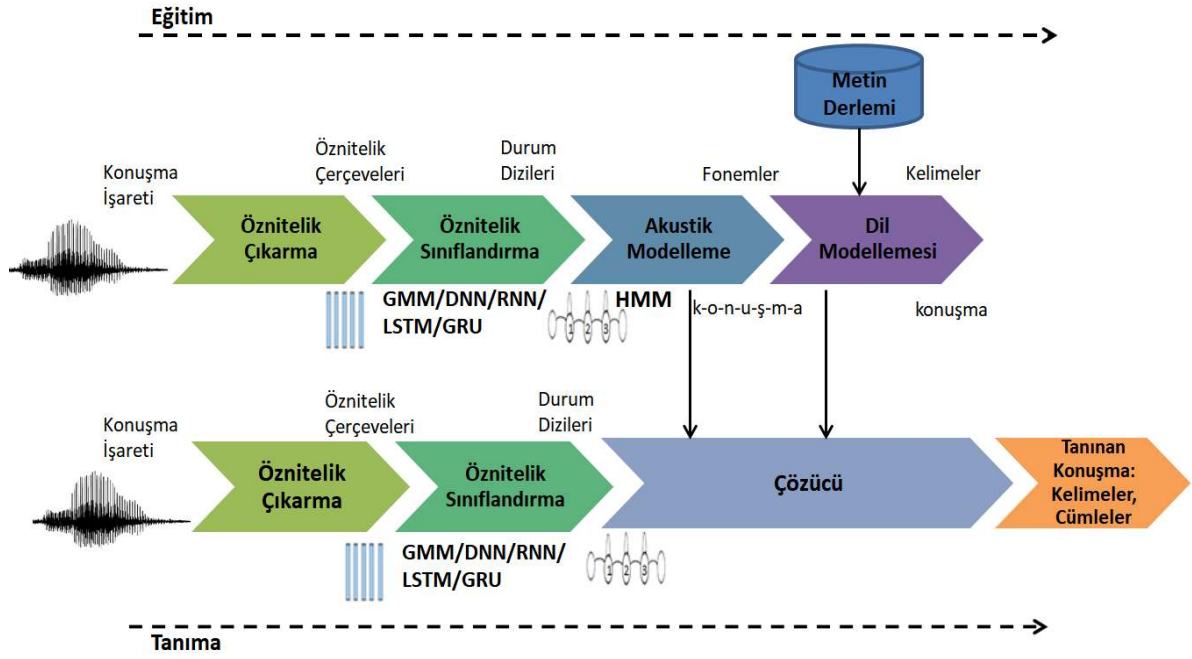
Şekil 4.3. ASR Sistemi
