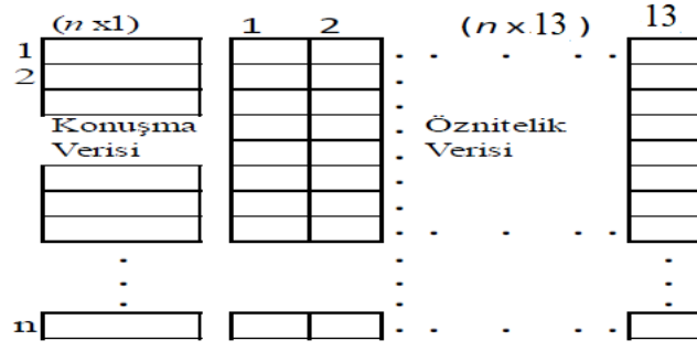
Şekil 6.4 Öznitelik matrisi
