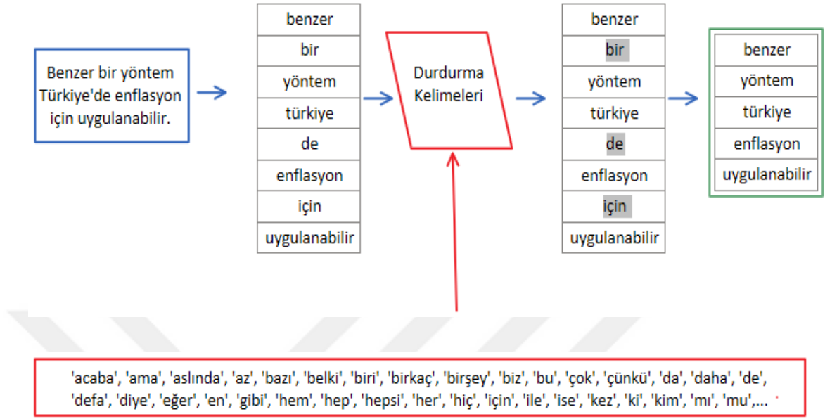
Şekil 7: Filtreleme Süreci Örneği
