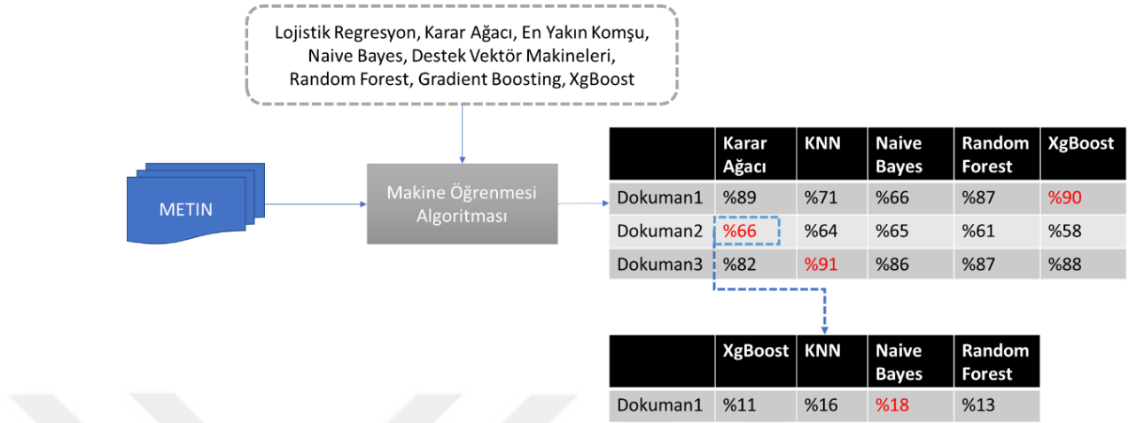
Şekil 15: Topik Modellemede Algoritmaların Sıralı Kullanımı
