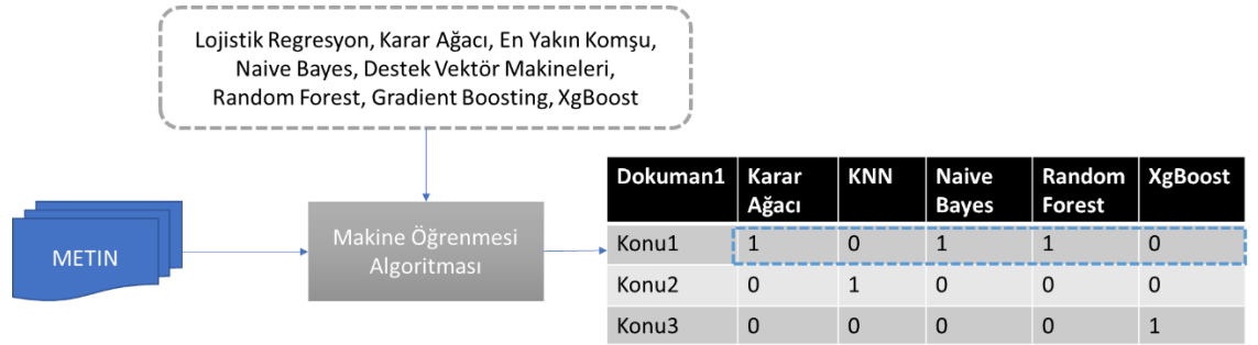
Şekil 16: Topik Modellemede Toplu Öğrenme Yöntemi
