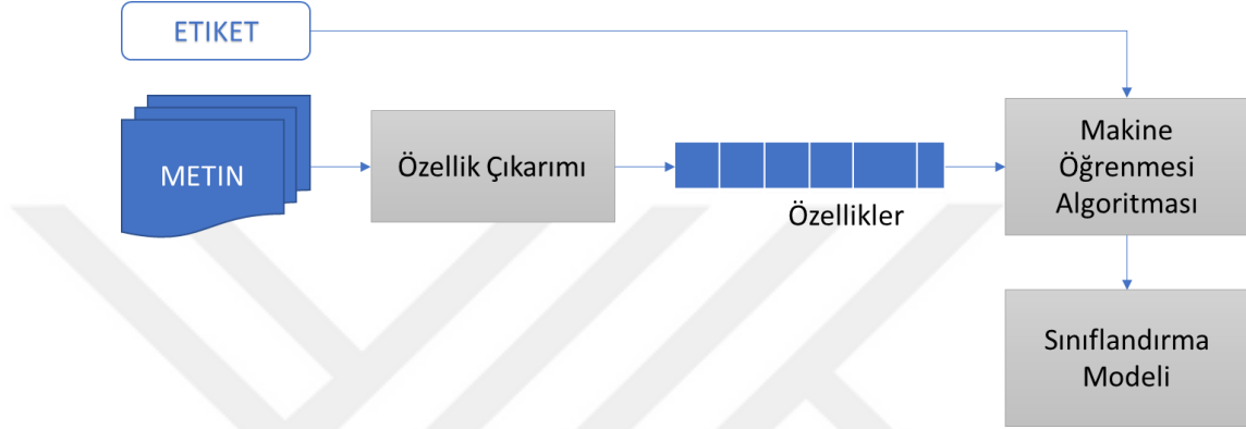
Şekil 9: Denetimli Öğrenme Süreci
