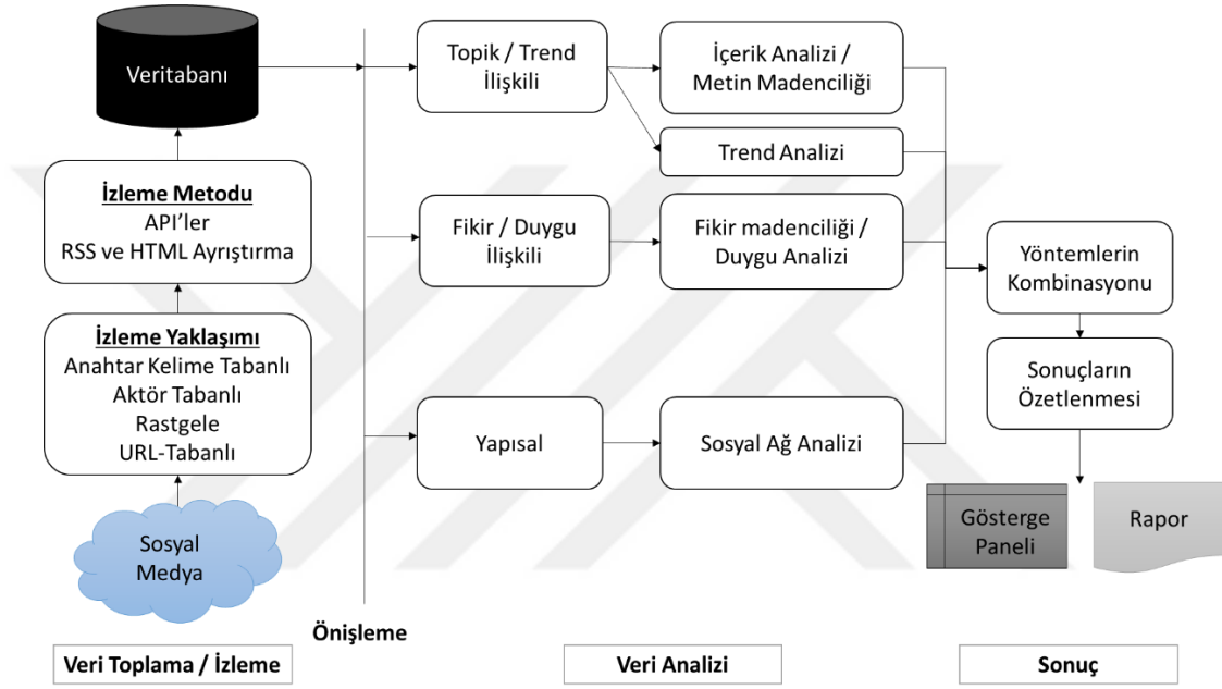
Şekil 21: Sosyal Medya Analitiği Süreci
