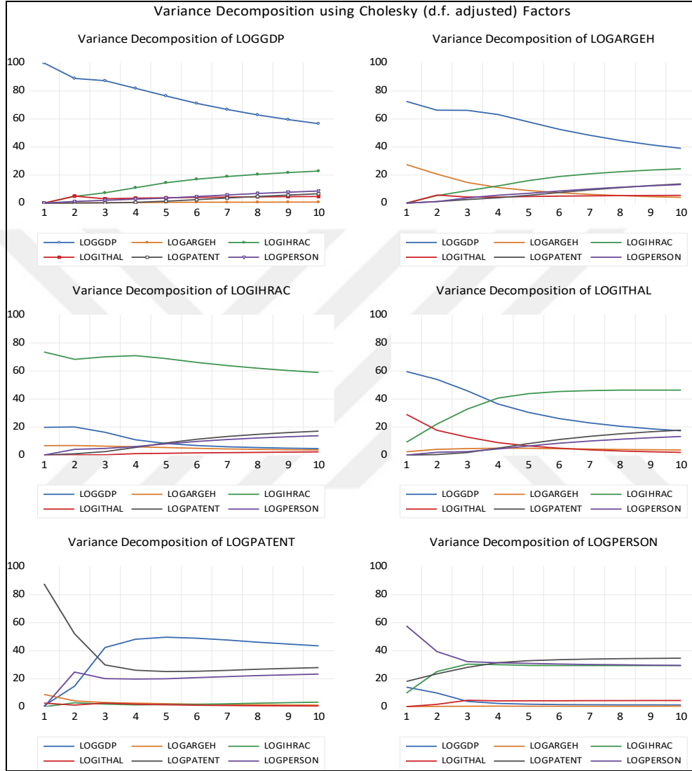
Şekil 19: Cholesky Bozulması
