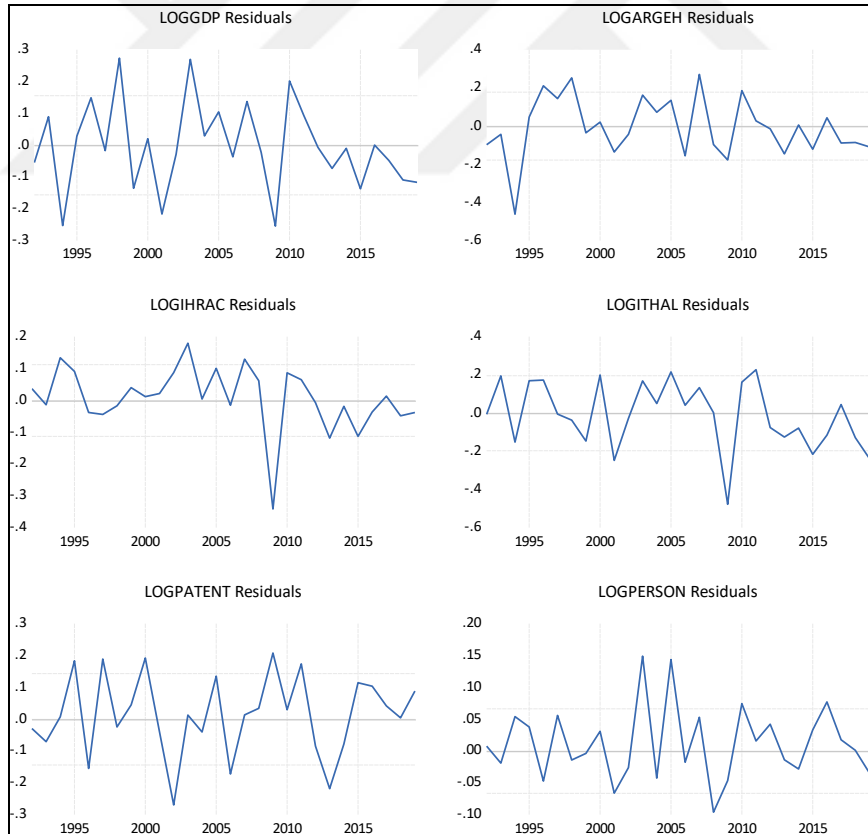
Şekil 16: Değişkenlerin Kalıntıları
