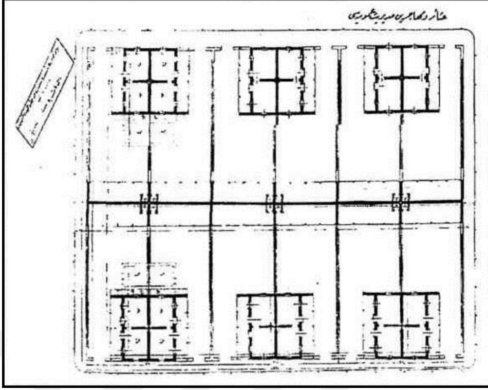
Resim 10. 1917 Tip Muhacir Köyü “12 Haneli Ada Planı” (Dündar 2000).
