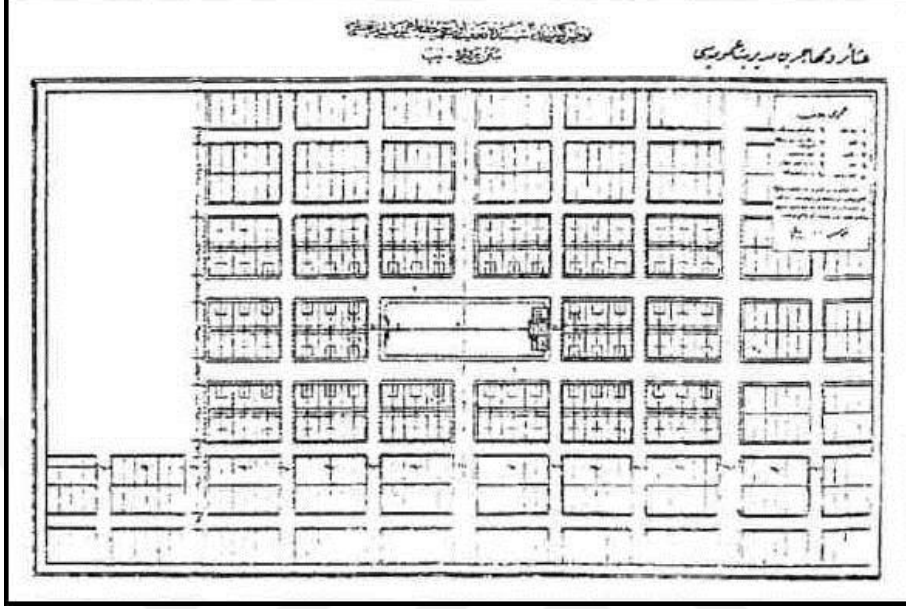
Resim 9. 1917 Tip Muhacir Köyü “Umumi Planı” (Dündar 2000).
