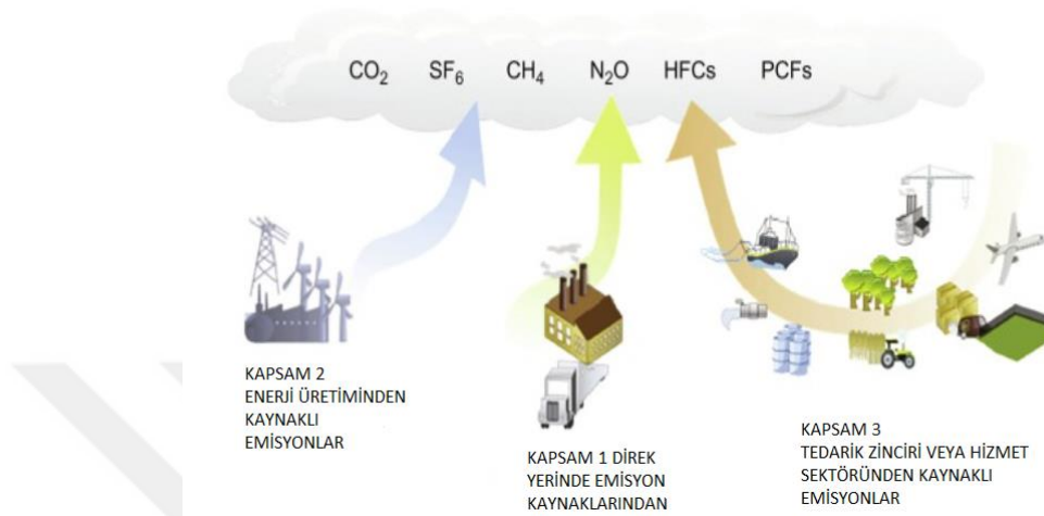
Şekil 2.9. Sera gazı emisyonlarının sınıflandırılmış kaynakları [38]
