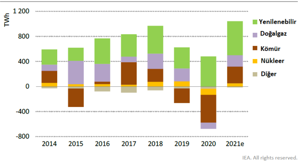
Şekil 2.2. Küresel Ölçekte elektrik üretimi değişim verileri (2014-2021) [29]
