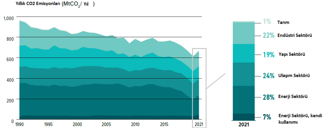
Şekil 2.7. Yıllara göre Yakıtların Yanmasından Kaynaklı CO 2 Emisyonları Değişimi ve Enerji Kaynaklarına göre Dağılımları (2022 verileri) [33]
