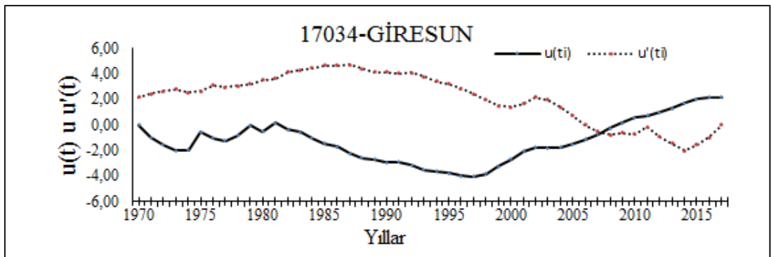
Şekil 3.8: 17034 Giresun istasyonu M-K merteye korelasyon test sonucu
