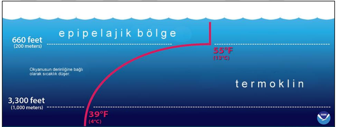
Şekil 1.2: Termoklin tabakasının katmanları
