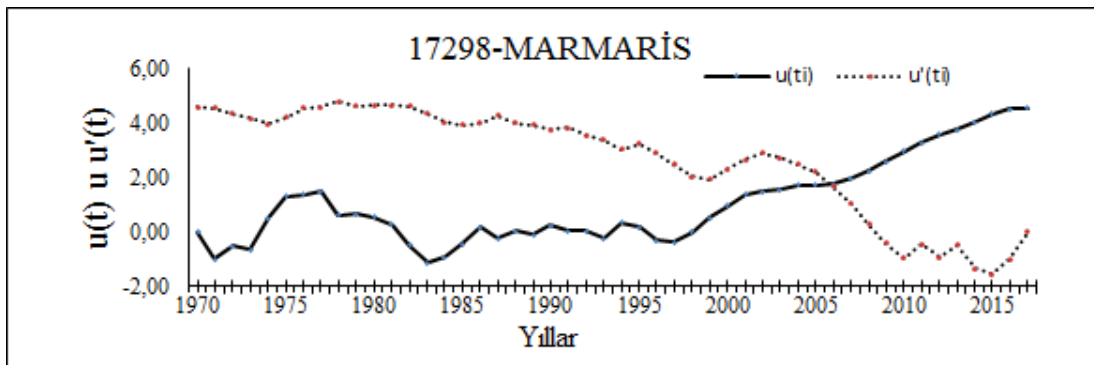
Şekil 3.20: 17298 Marmaris istasyonu M-K merteye korelasyon test sonucu
