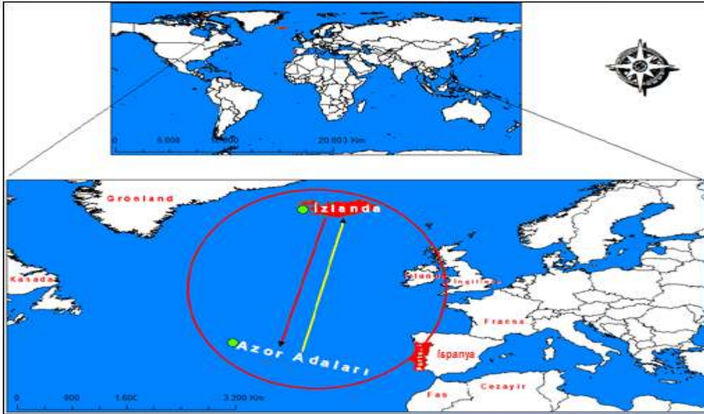
Şekil 1.5: Kuzey Atlantik salınınının haritada konumsal olarak gösterimi
