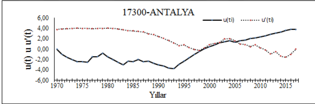
Şekil 3.22: 17300 Antalya istasyonu M-K merteye korelasyon test sonucu
