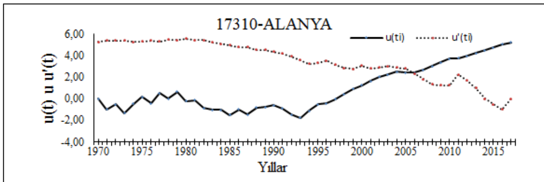
Şekil 3.23: 17310 Alanya istasyonu M-K merteye korelasyon test sonucu
