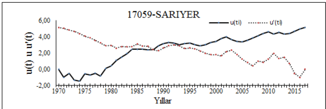
Şekil 3.11: 17059 Sarıyer istasyonu M-K mertebe korelasyon test sonucu
