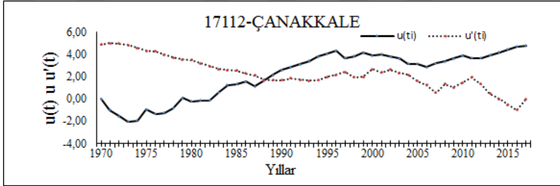
Şekil 3.13: 17112 Çanakkale istasyonu M-K merteye korelasyon test sonucu
