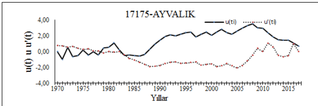
Şekil 3.14: 17175 Ayvalık istasyonu M-K merteye korelasyon test sonucu
