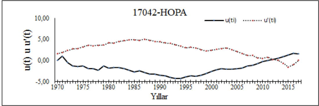
Şekil 3.9: 17042 Hopa istasyonu M-K mertebe korelasyon test sonucu
