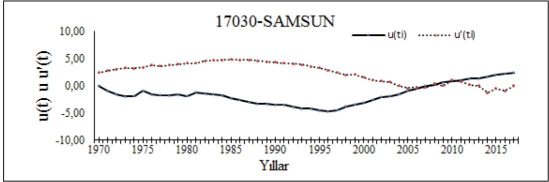
Şekil 3.6: 17030 Samsun istasyonu M-K merteye korelasyon test sonucu
