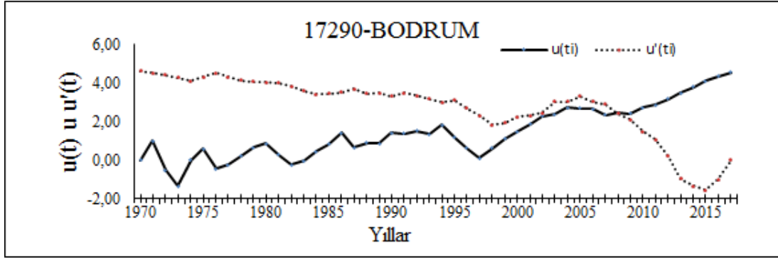
Şekil 3.18: 17290 Bodrum istasyonu M-K merteye korelasyon test sonucu
