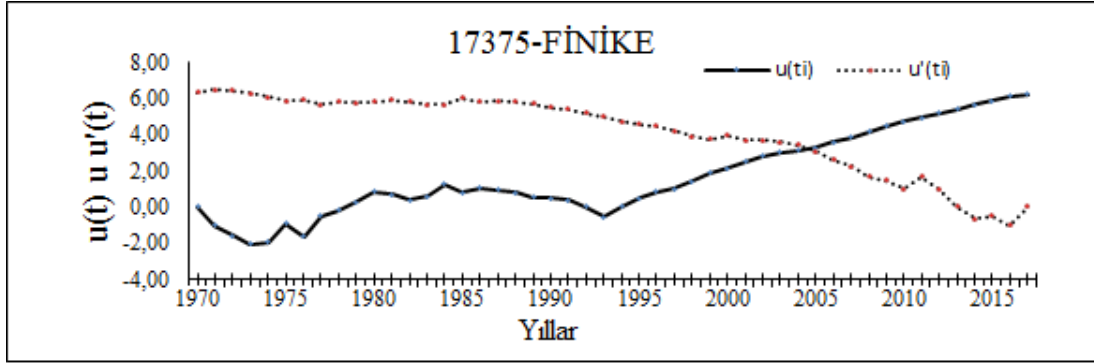
Şekil 3.21: 17375 Finike istasyonu M-K merteye korelasyon test sonucu
