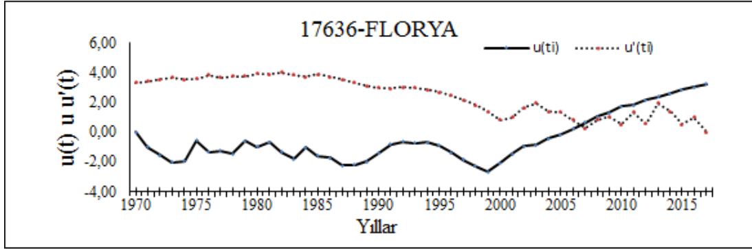
Şekil 3.12: 17636 Florya istasyonu M-K merteye korelasyon test sonucu
