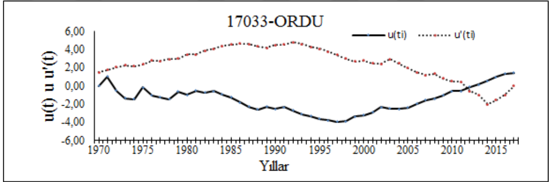
Şekil 3.7: 17033 Ordu istasyonu M-K merteye korelasyon test sonucu
