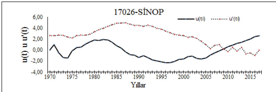
Şekil 3.5: 17026 Sinop istasyonu M-K mertebeye korelasyon test sonucu
