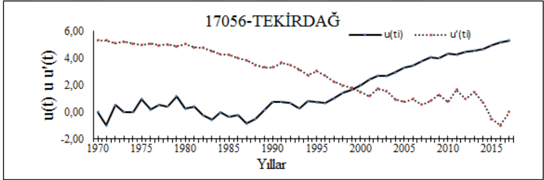
Şekil 3.10: 17056 Tekirdağ istasyonu M-K mertebe korelasyon test sonucu
