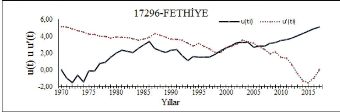
Şekil 3.19: 17296 Fethiye istasyonu M-K merteye korelasyon test sonucu
