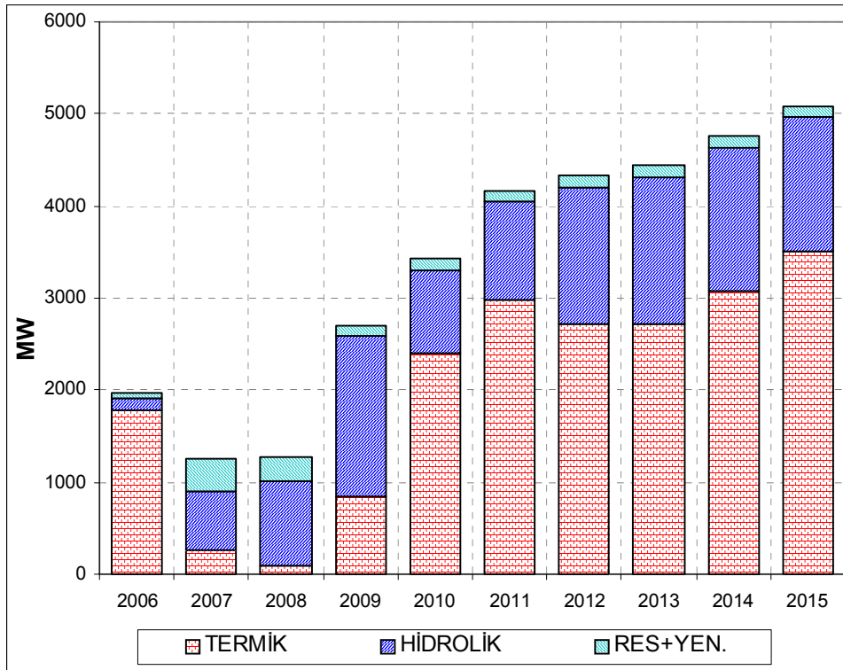
Grafik 7: Kapasite İlavesinin Termik – Hidrolik Dağılımı (Çözüm I)
