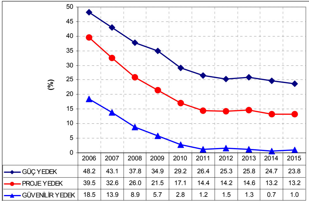
Grafik 18: Kurulu Güç, Proje Üretim ve Güvenilir Üretim Yedeği (Çözüm II)
