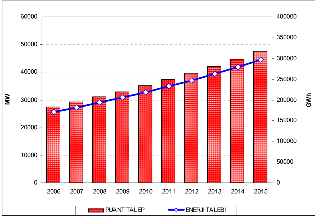
Grafik 2: Talep Tahmini (Senaryo 2, Düzenlenmiş Düşük Senaryo)
