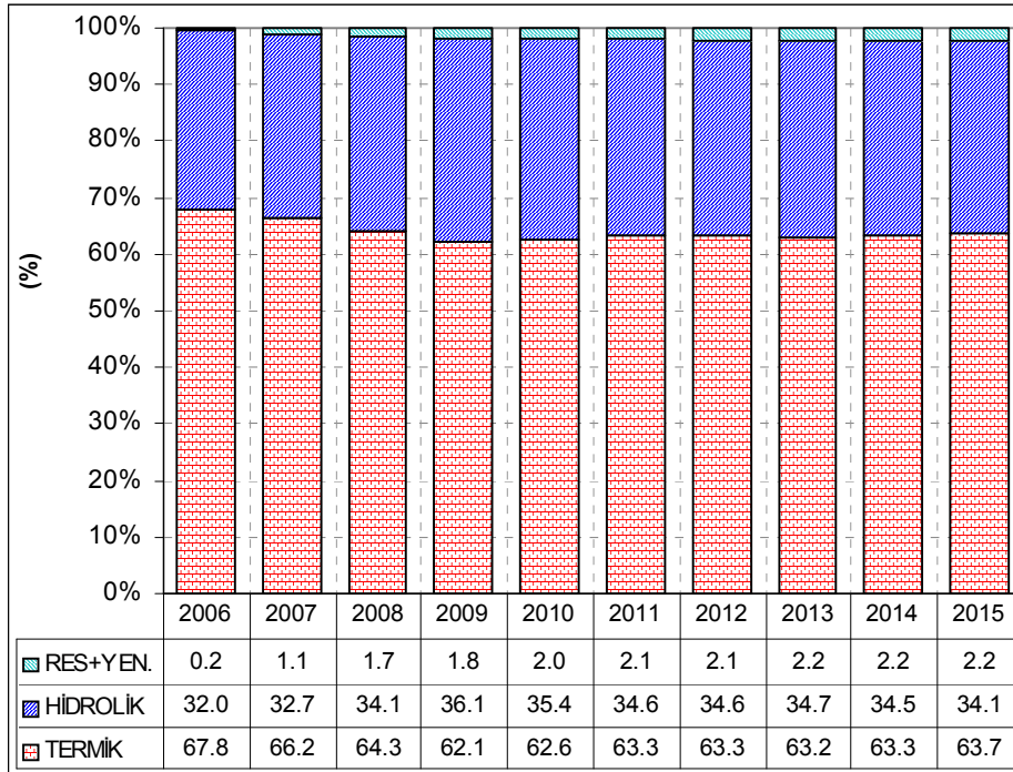
Grafik 9: Kurulu Gücün Termik Hidrolik Dağılımı (Çözüm I)
