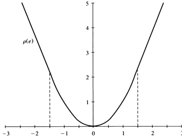
Şekil 1: k = 1.5\hat{\sigma} iken Huber 'in M-tahmini tanımında kullanılan \rho(e) fonksiyonunun grafiği.
