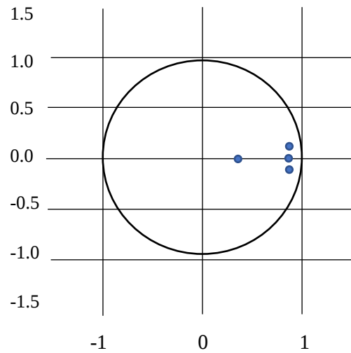
Grafik 8. AR Karakteristik Polinomun Ters Kökleri
