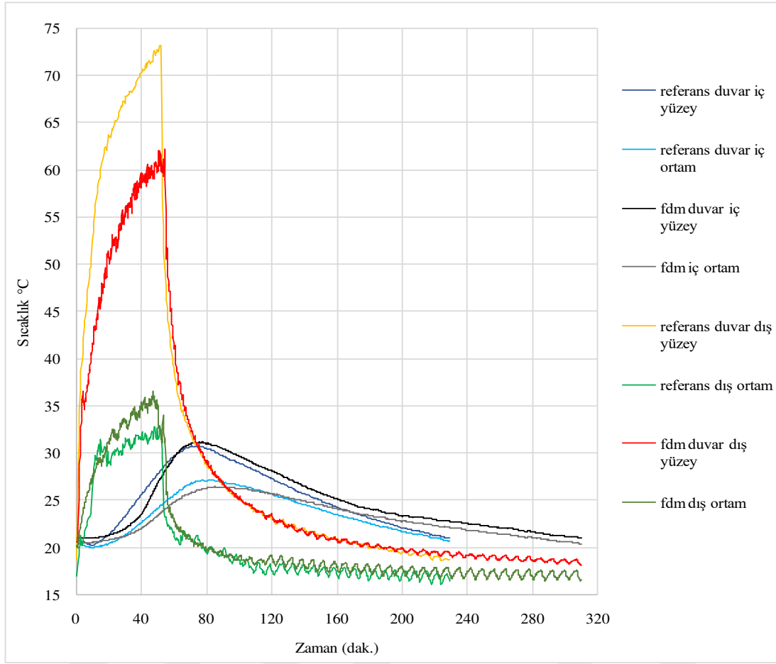
Şekil 50. 800W/m 2 'lik güneş ışınlam değeri uygulanarak yapılan uygulama bulgularının grafiksel gösterimi
