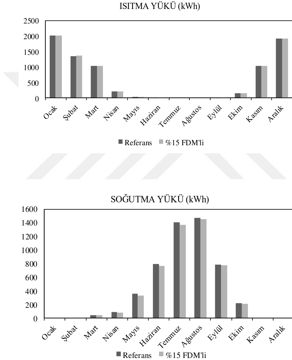
Şekil 42. Ankara ilinde %15 FDM' li örnek ile referans örneğin kullanılması durumunda elde edilen aylık ısıtma ve soğutma bina enerji yüklerinin karşılaştırılması
