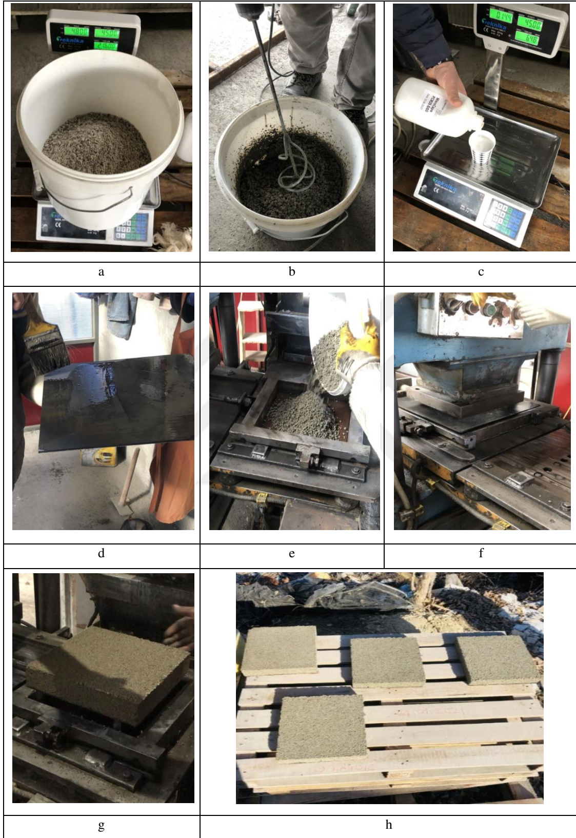
Şekil 18. (a) Pomza agregası ve çimentonun tartılması, (b) Karışımın su eklenerek karıştırılması, (c) FDM'nin tartılması, (d) Sacın yağlanması, (e) Karışımın kalıba dökülmesi, (f) Press makinesinde basınç uygulanması (g) Karışımın kalıptan çıkarılması, (h) FDM'li örnekler ile FDM'siz örneğin kurumaya bırakılması
