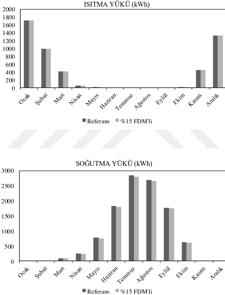
Şekil 44. Diyarbakır ilinde %15 FDM' li örnek ile referans örneğin kullanılması durumunda elde edilen aylık ısıtma ve soğutma bina enerji yüklerinin karşılaştırılması
