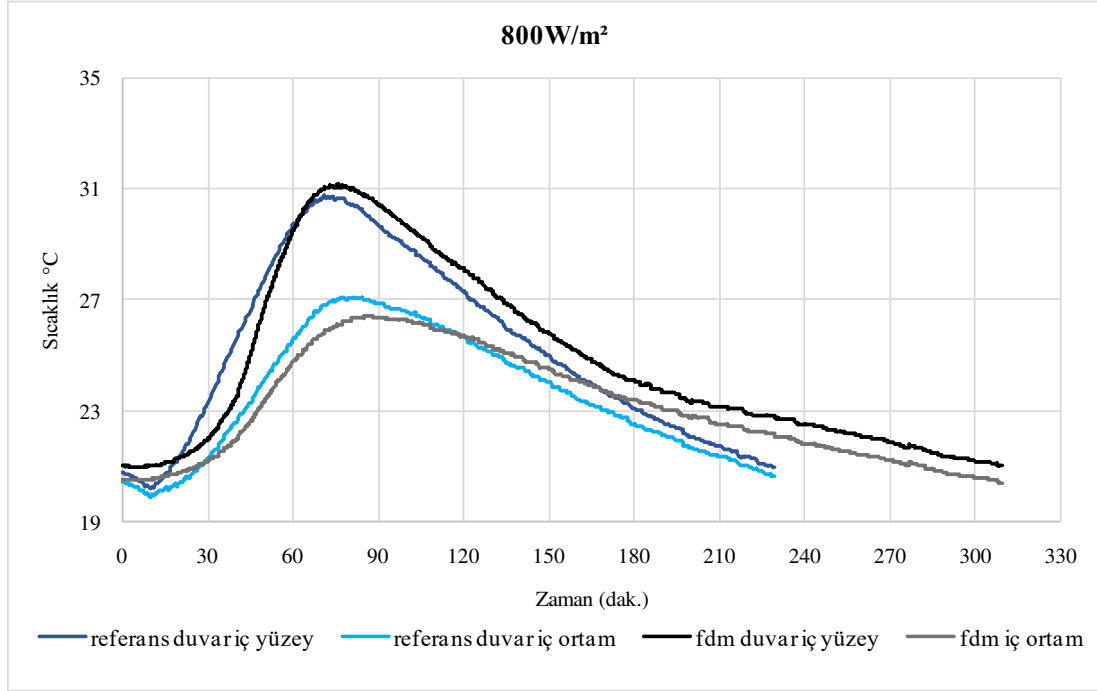
Şekil 49. 800W/m 2 'lik güneş ışıınım değeri uygulanması ile FDM'siz ve FDM'li kabinlerin duvar iç yüzey ve iç ortam sıcaklıklarındaki değışim
