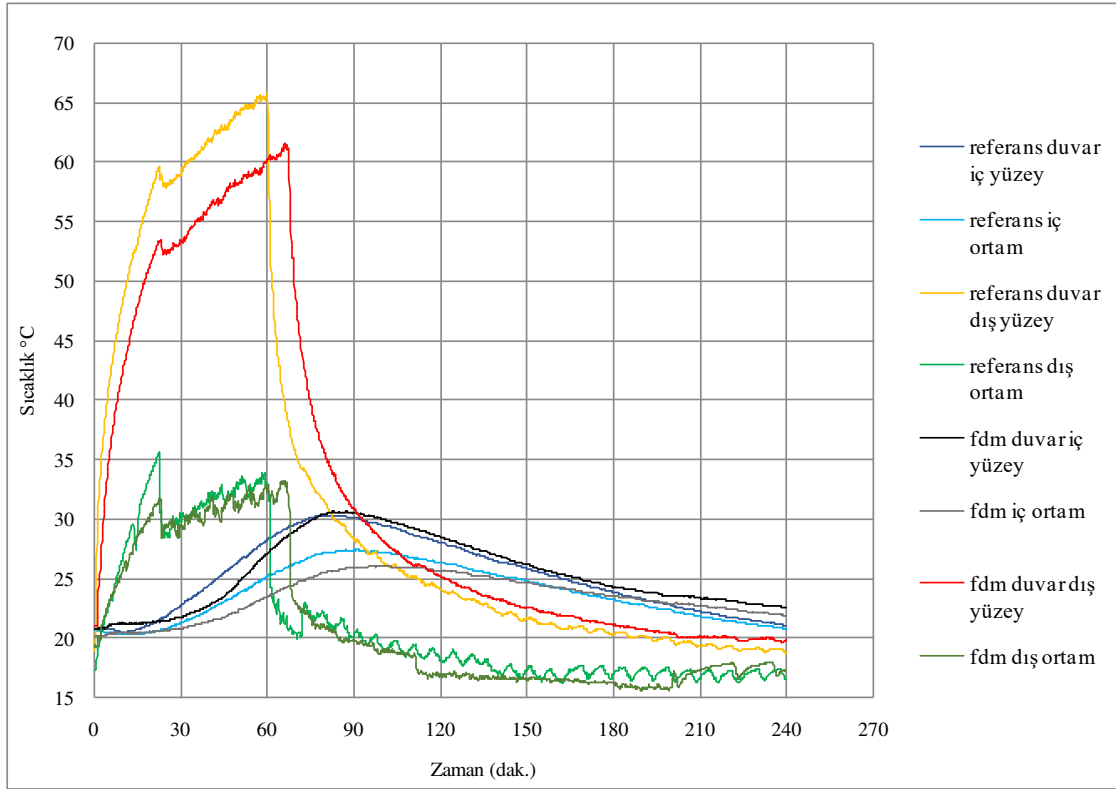
Şekil 48. 600W/m 2 'lik güneş ışınlam değeri uygulanarak yapılan uygulama bulgularının grafiksel gösterimi
