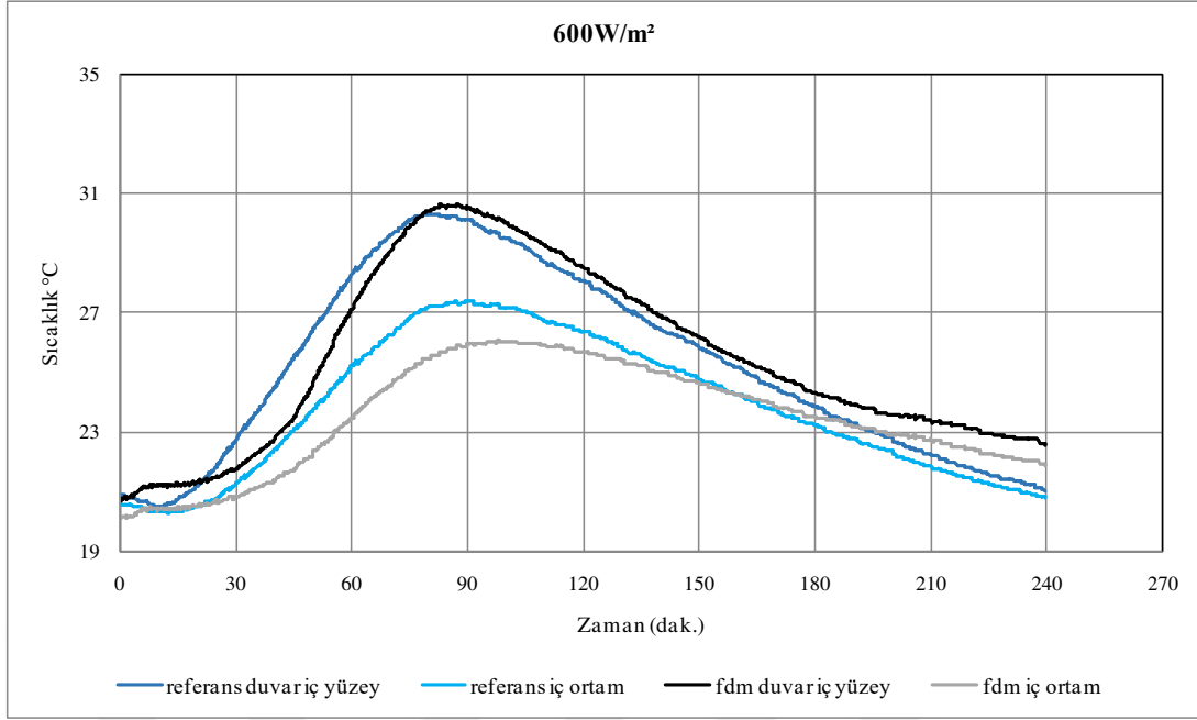
Şekil 47. 600W/m 2 'lik güneş ışınlam değeri uygulanması ile FDM'siz ve FDM'li kabinlerin duvar iç yüzey ve iç ortam sıcaklıklarındaki değişim
