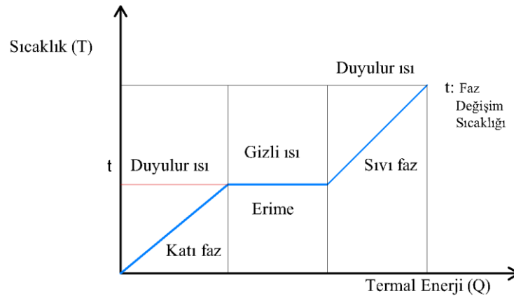
Şekil 2. Duyulur ve gizli ısı depolama [56].
