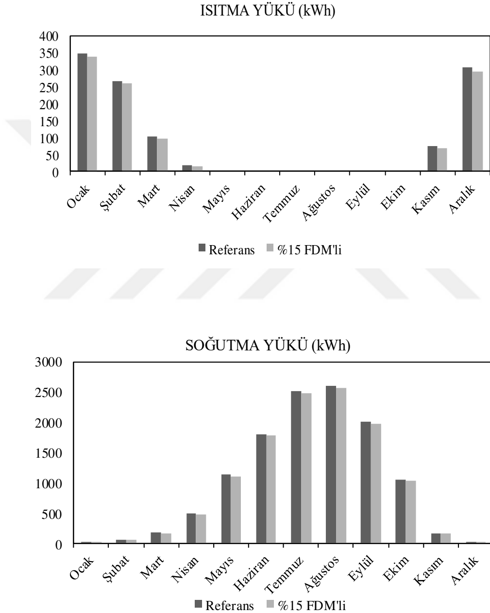
Şekil 43. Antalya ilinde %15 FDM' li örnek ile referans örneğin kullanılması durumunda elde edilen aylık ısıtma ve soğutma bina enerji yüklerinin karşılaştırılması
