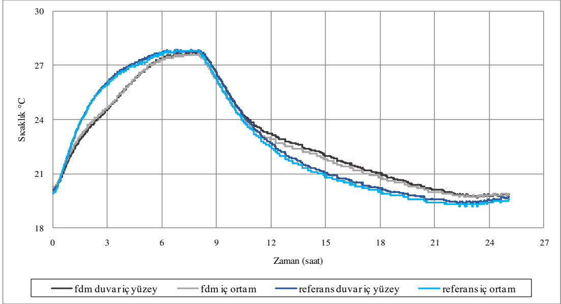
Şekil 51. Fırın içerisinde yapılan uygulamada FDM'siz ve FDM'li kabinlerin duvar iç yüzey ve iç ortam sıcaklıklarındaki değişim
