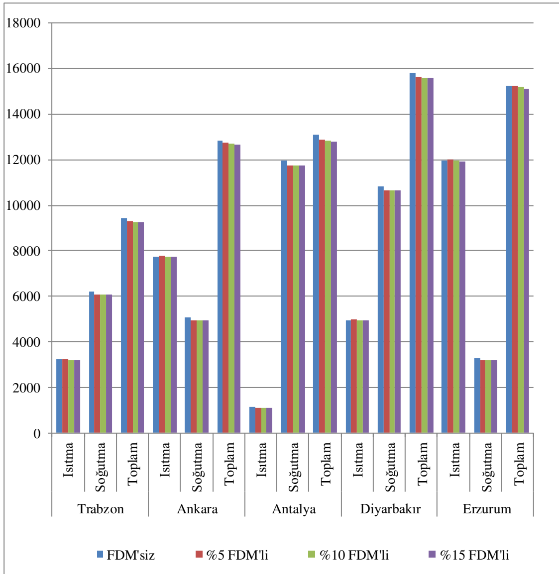
Şekil 46. FDM'siz ve %5, %10 ve %15 FDM'li örneklerin pilot illerdeki yıllık ısıtma, soğutma ve toplam enerji yüklerinin karşılaştırılması
