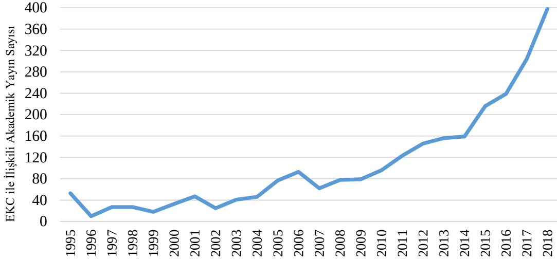
Şekil 2.5. Çevresel Kuznets Eğrisinin Akademik Popülaritesi (Kaynak: Elsevier-Sciencedirect)
