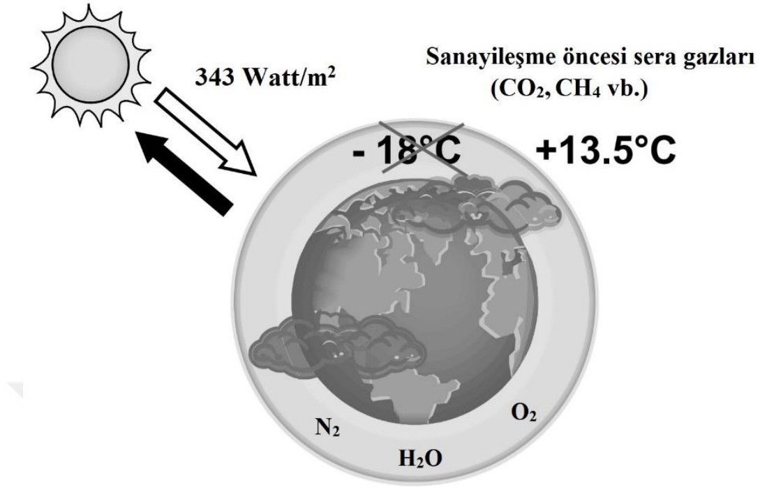
Şekil 1.10. Dünyanın Isınması ve Sera Gazları (Kaynak: Sinn, 2016)
