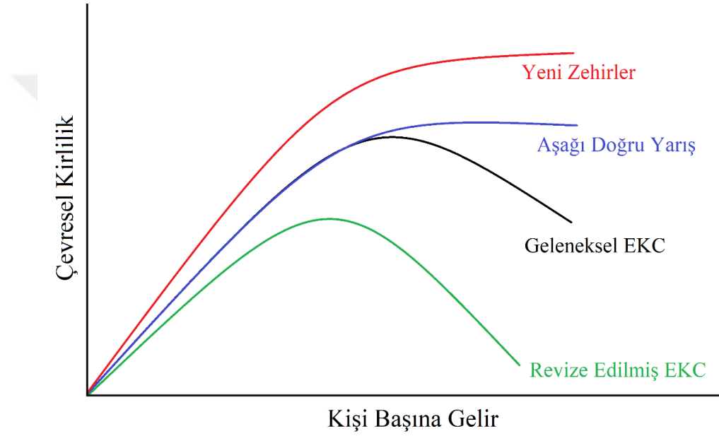
Şekil 2.2. Çevresel Kuznets Eğrisi: Alternatif Senaryolar (Kaynak: Dasgupta vd. 2002'den uyarlanmıştır)
