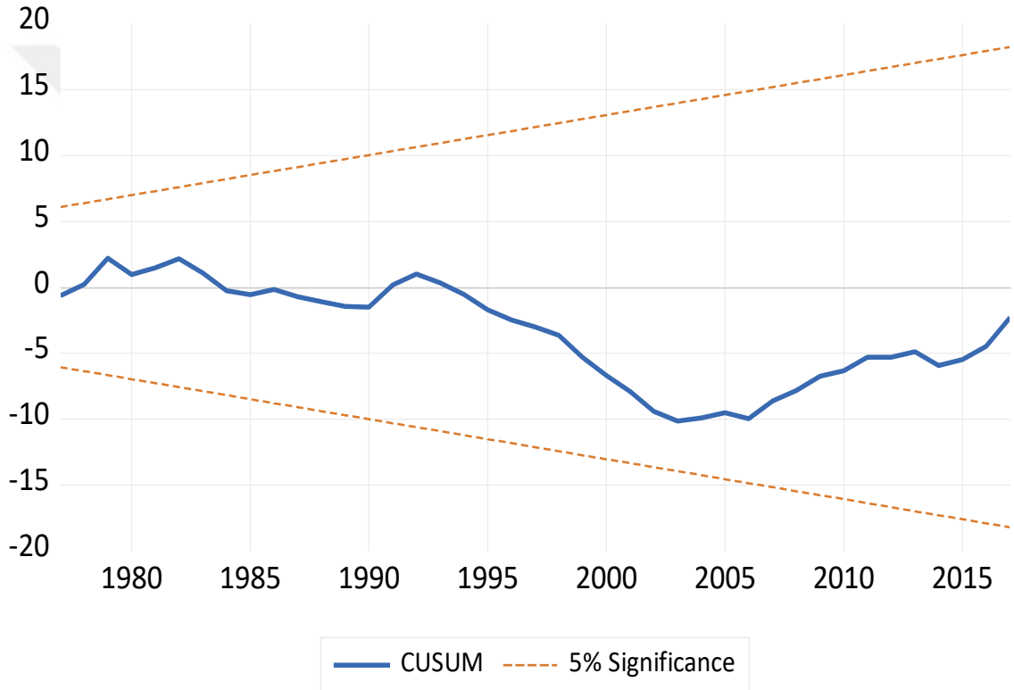
Şekil 3.3. CUSUM Test Sonucu
