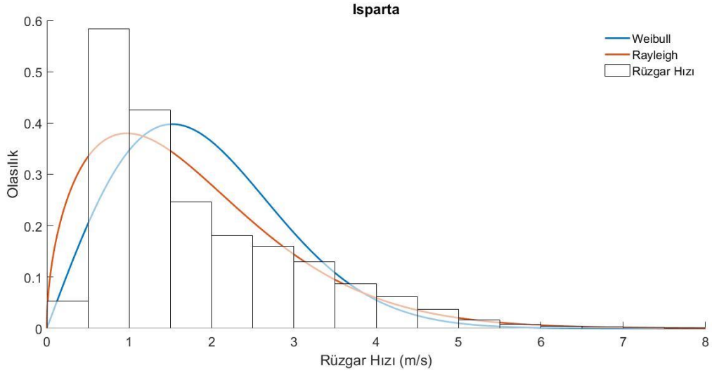
Şekil 5.9. Isparta ili için dağılım fonksiyonlarının karşılaştırılması
