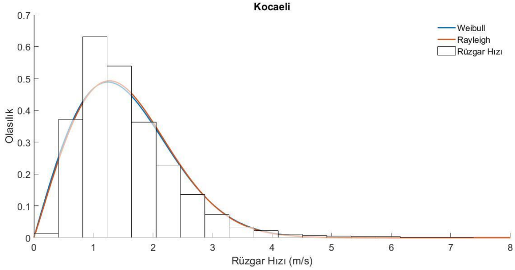
Şekil 5.2. Kocaeli ili için dağılım fonksiyonlarının karşılaştırılması
