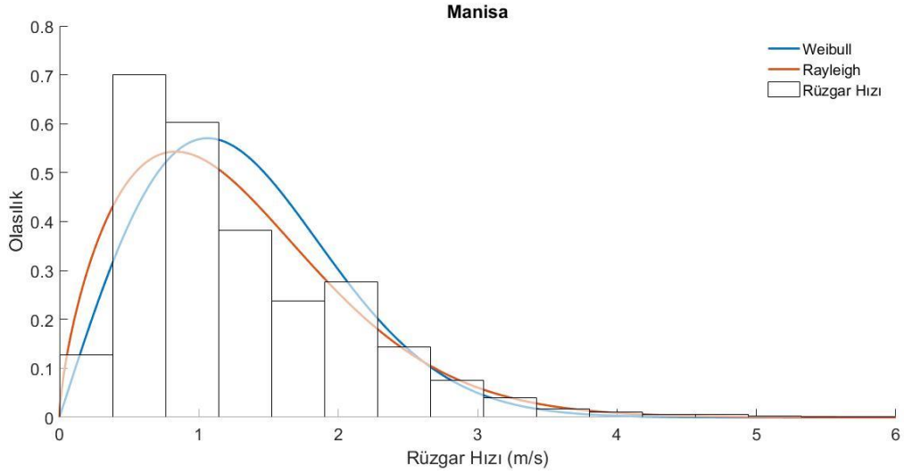
Şekil 5.5. Manisa ili için dağılım fonksiyonlarının karşılaştırılması,
