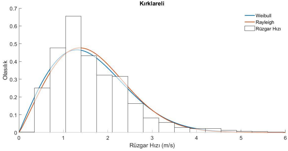
Şekil 5.3. Kırklareli ili için dağılım fonksiyonlarının karşılaştırılması
