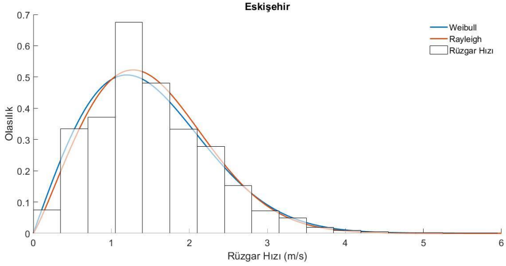
Şekil 5.10. Eskişehir ili için dağılım fonksiyonlarının karşılaştırılması
