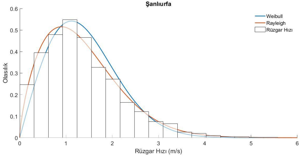
Şekil 5.20. Şanlıurfa ili için dağılım fonksiyonlarının karşılaştırılması
