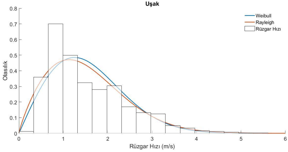
Şekil 5.6. Uşak ili için dağılım fonksiyonlarının karşılaştırılması
