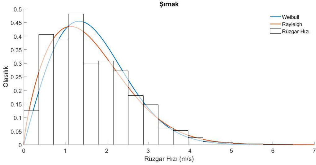
Şekil 5.21. Şırnak ili için dağılım fonksiyonlarının karşılaştırılması
