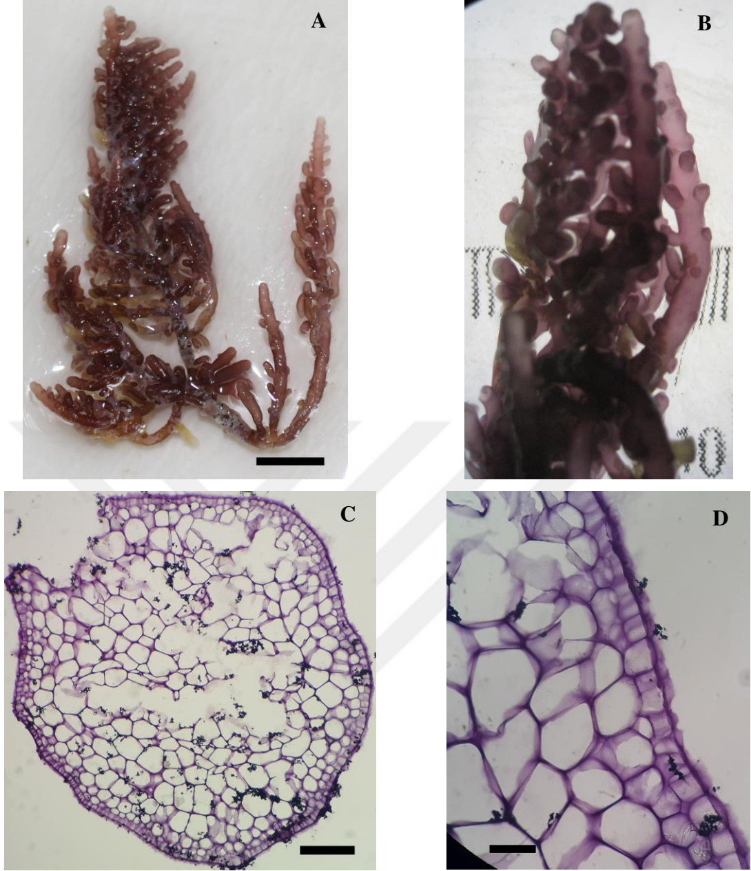
Şekil 3.8. Osmundea verlaquei genel görünüm (A; Skala=1 cm), tallusun dallanma şekli (B) ve epidermal hücrelerin düzeni (C, D; Skala= 40 \mu m).
