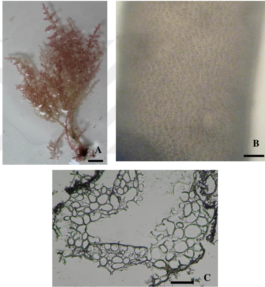
Şekil 3.1. Chondrophycus glandulifer tallus genel görünüm (A; Skala=1 cm), yüzey görüntüsünde ikincil bağlantılar (B; Skala=10 µm), tallus enine kesitte epidermal hücreler (C; Skala=20 µm).
