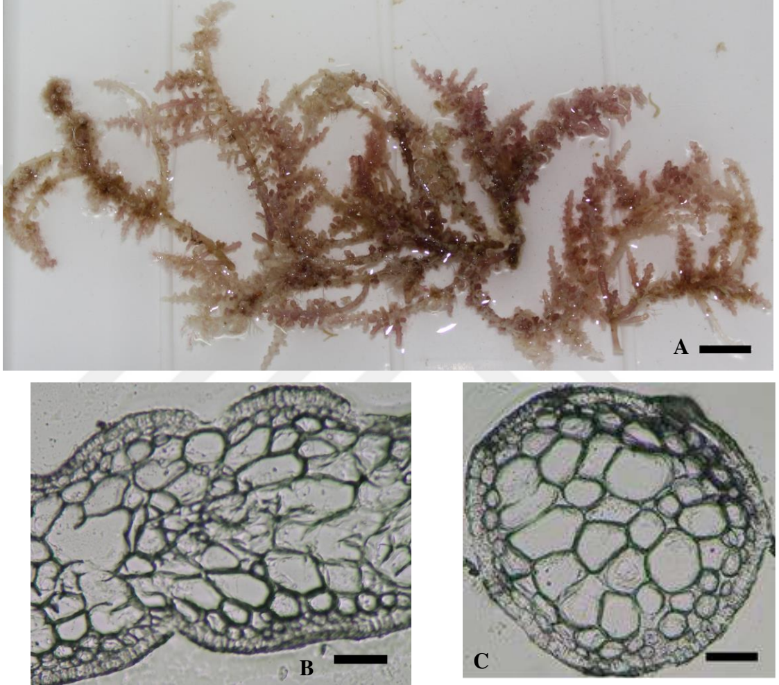
Şekil 3.6. Osmundea maggsiana genel görünüm (A; Skala=1 cm) ve enine kesit görüntüleri (B,C; Skala= 40 \mu m).
