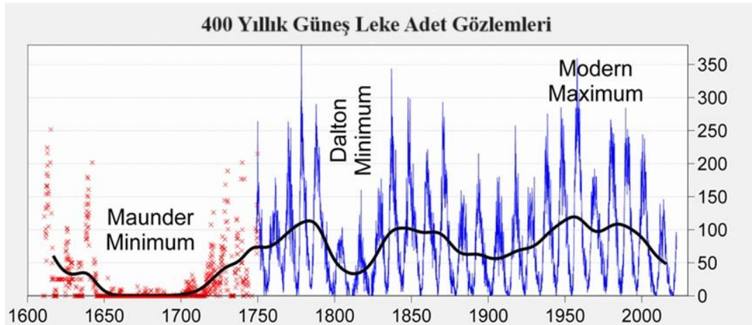
Şekil 2.4. Son 400 yıldaki Güneş lekesi sayılarının değişimi [99].
