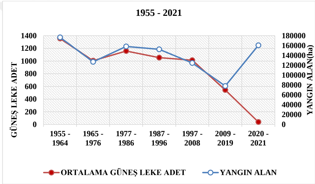
Şekil 4.1. 1955-2021 yılları arasındaki Güneş leke çevrimlerindeki Güneş lekelerinin ortalamalarının toplamaları ile bu çevrimler içindeki yıllık orman yangın alanlarının toplamalarının karşılaştırılması (Veriler için sırasıyla Tablo 3.1. ve Tablo 3.2.'ye bakınız).
