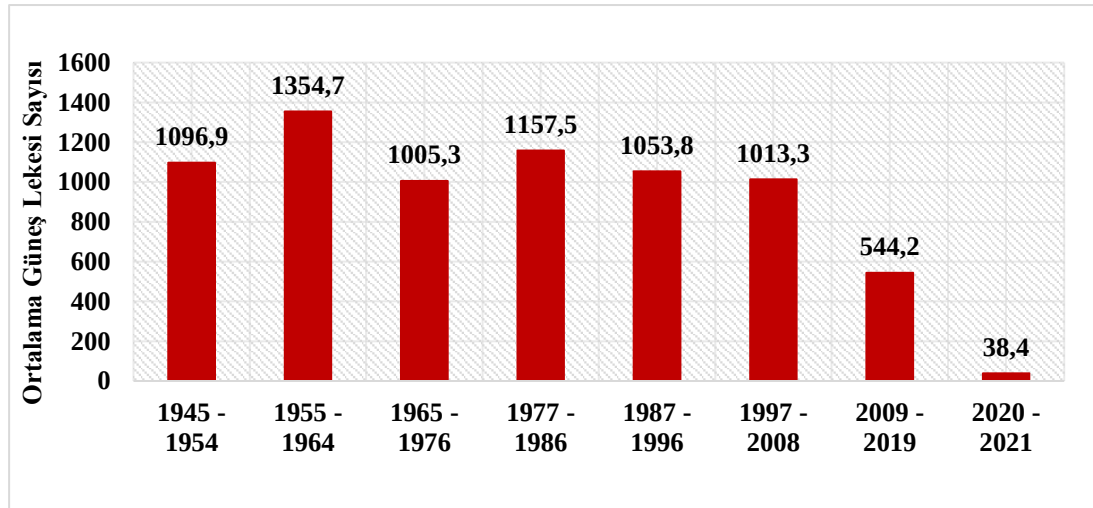
Şekil 3.2. Her bir Güneş leke çevrimi içindeki yıllık ortalama sayılarının toplamalarının zaman içindeki dağılımı. (Toplam sayılar için Tablo 3.1.'e bakınız).
