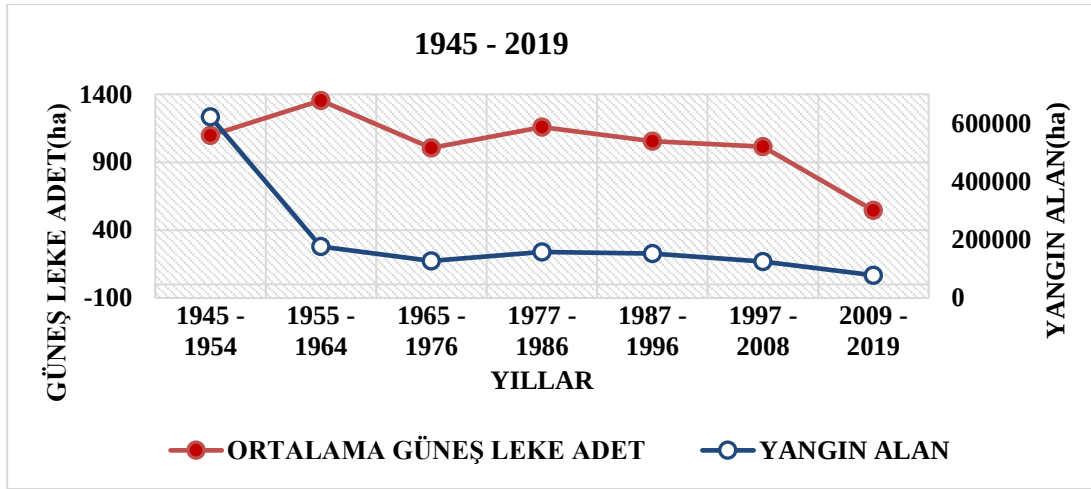
Şekil 4.2. 1945-2019 yılları arasındaki Güneş leke çevrimlerindeki Güneş lekelerinin ortalamalarının toplamaları ile bu çevrimler içindeki yıllık orman yangın alanlarının toplamalarının karşılaştırılması (Veriler için sırasıyla Tablo 3.1. ve Tablo 3.2.'ye bakınız).
