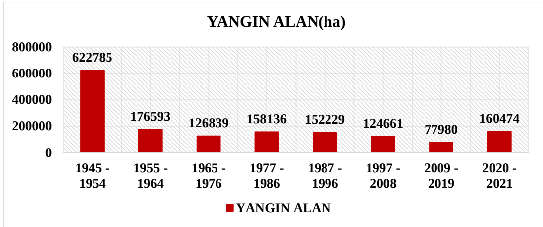
Şekil 3.6. Güneş leke çevrimi aralıklarındaki orman yangın alanlarının(ha) toplamalarının dağılımı(Veriler için Tablo 3.2.'ye bakınız).
