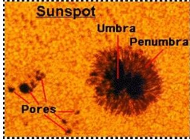
Şekil 2.3. Bir Güneş lekесinin bölümleri [75].
