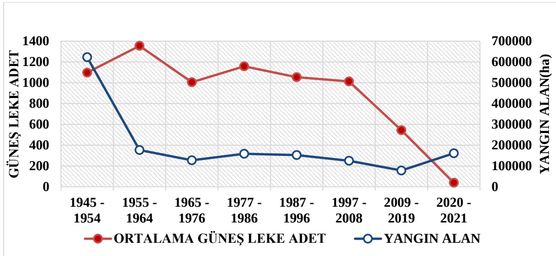
Şekil 3.9. 1945-2021 yılları arasındaki Güneş lekelerinin yıllık ortalama sayılarının Güneş leke çevrimlerindeki toplamaları ile bu çevrimler içindeki yıllık orman yangın alanlarının toplamalarının karşılaştırılması (Veriler için sırasıyla Tablo 3.1. ve Tablo 3.2.'ye bakınız).
