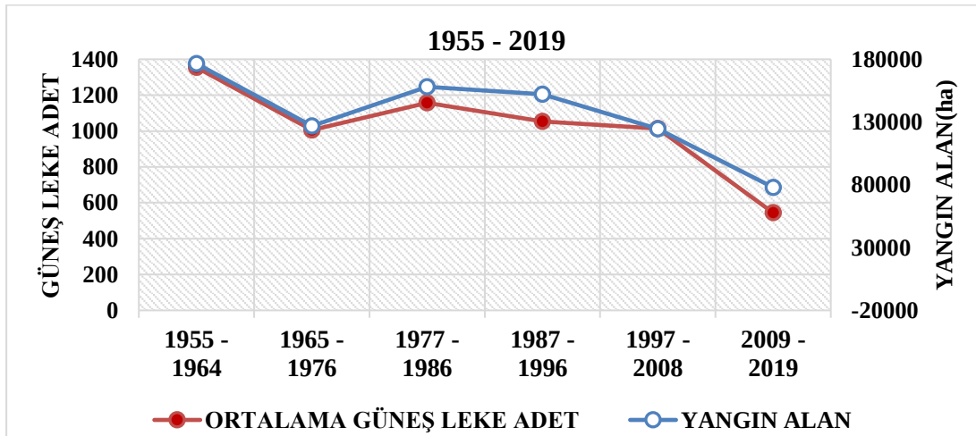
Şekil 4.3. 1955-2019 yılları arasındaki Güneş leke çevrimlerindeki Güneş lekelerinin ortalamalarının toplamaları ile bu çevrimler içindeki yıllık orman yangın alanlarının toplamalarının karşılaştırılması (Veriler için sırasıyla Tablo 3.1. ve Tablo 3.2.'ye bakınız).
