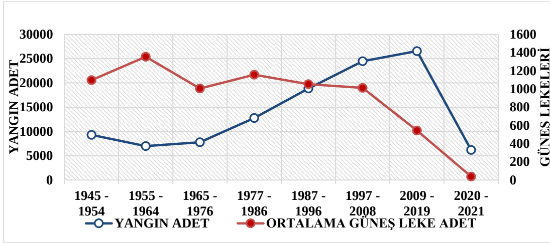
Şekil 3.8. 1945-2021 yılları arasındaki Güneş lekelerinin yıllık ortalama sayılarının Güneş leke çevrimlerindeki toplamaları ile bu çevrimler içindeki yıllık orman yangını sayısının toplamalarının karşılaştırılması (Veriler için sırasıyla Tablo 3.1. ve Tablo 3.2.'ye bakınız).
