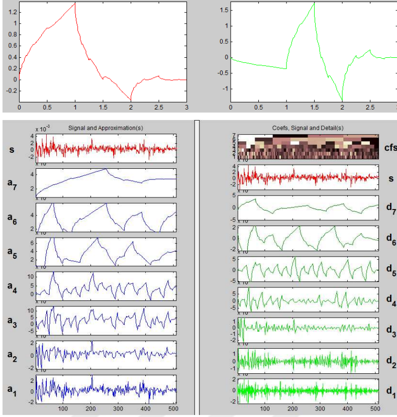
Şekil 7.10 Daubechies2-Seviye7 Ayrıştırma ve Ölçekleme Dalgacıkları RDİBS Ayrıştırması (Pointed)
