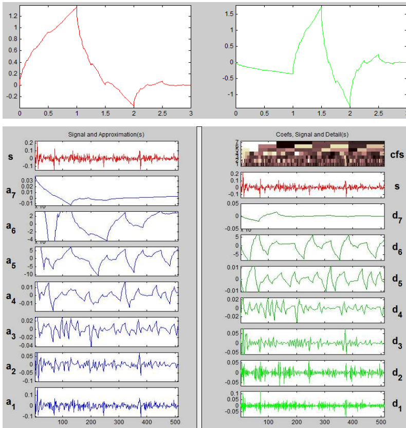
Şekil 7.9 Daubechies2-Seviye7 Ayrıştırma ve Ölçekleme Dalgacıkları RCDS Ayrıştırması (Pointed)
