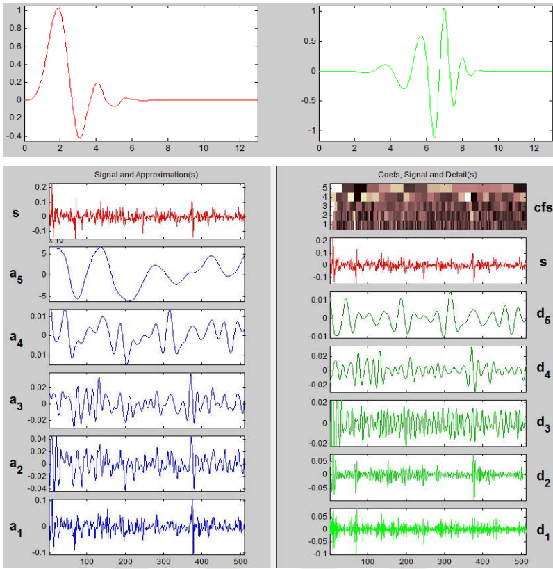
Şekil 7.13 Daubechies7-Seviye5 Ayırıştırma ve Ölçekleme Dalgacıkları RCDS Ayırıştırması (Smooth)
