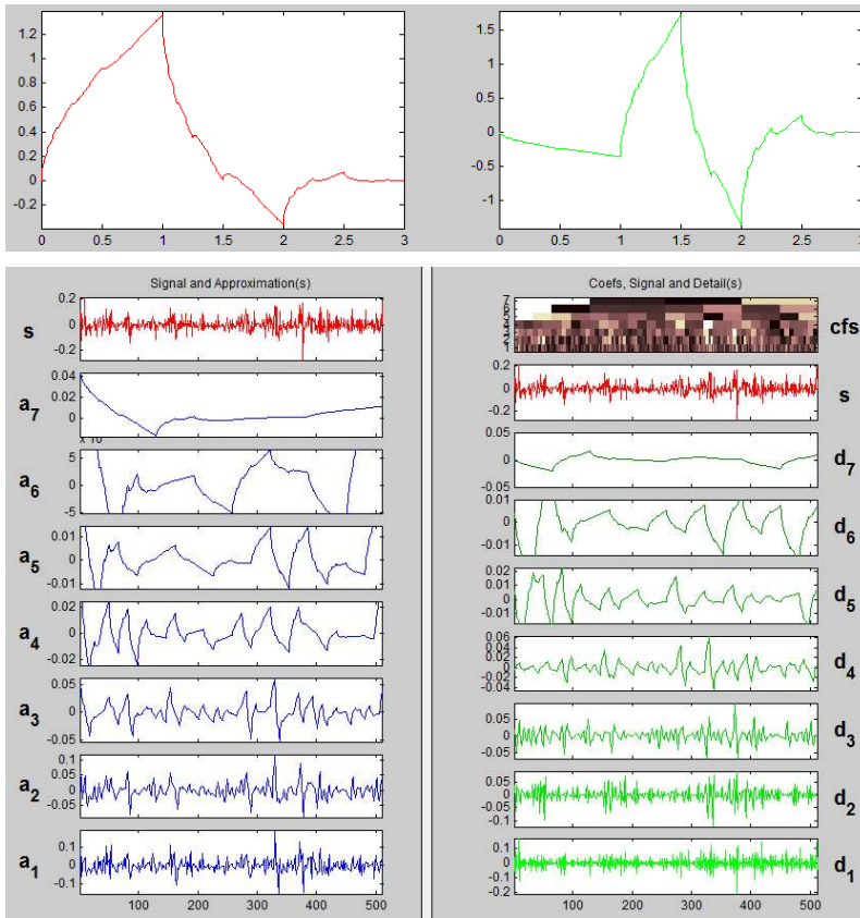
Şekil 7.11 Daubechies2-Seviye7 Ayrıştırma ve Ölçekleme Dalgacıkları RVIX Ayrıştırması (Pointed)
