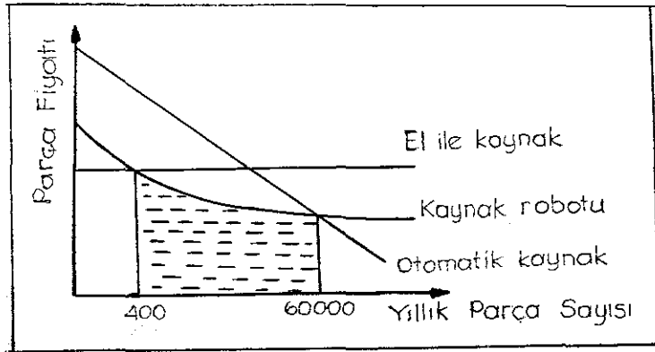
Şekil.2.14. Yıllık Parça Üretiminde Parça Başına düşen Maliyetler
