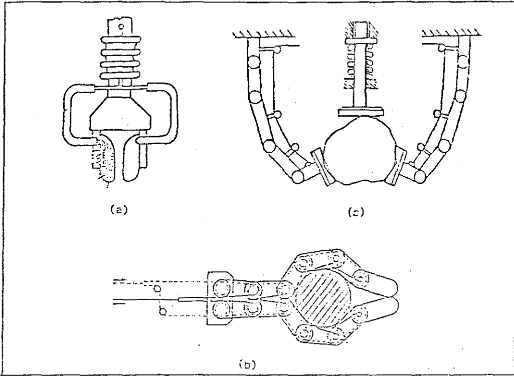
Şekil 2.8. Universal Kavrayıcılar
