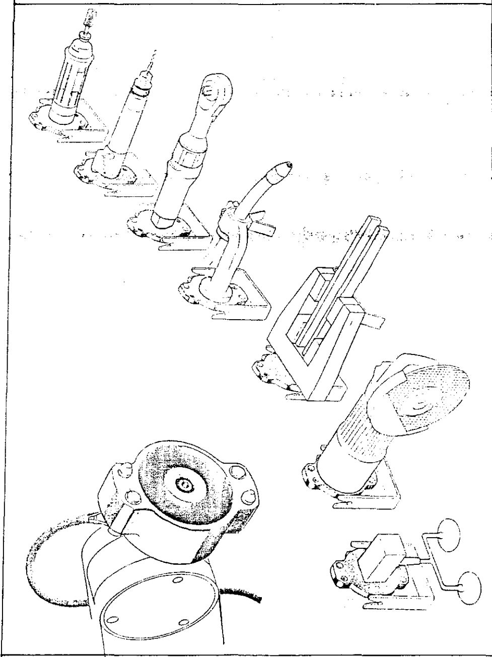
řekil 2.9. Robot Bileėinde Kullanılan Takım ve Aparatlar
