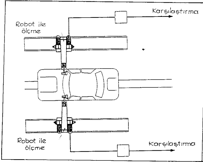
Şekil 7. Otomobil karöserlerinin kalite kontrolü.
