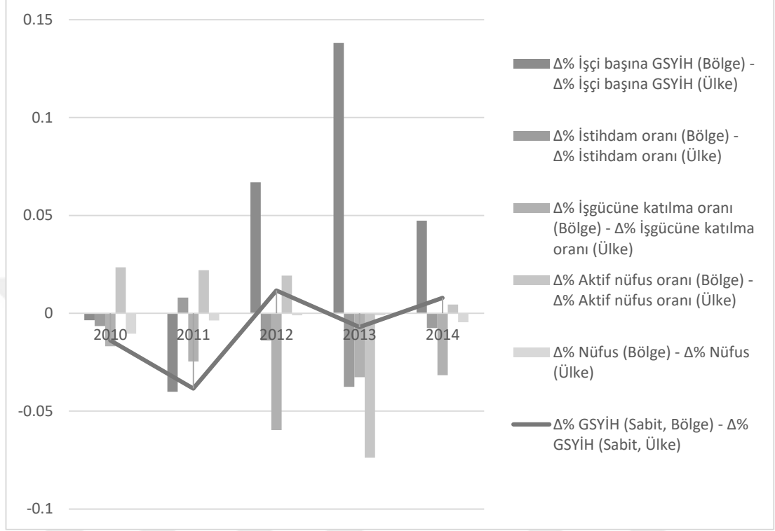
Grafik 3. 6: Gaziantep, Adıyaman, Kilis (TRC1) bölgesinin bölgesel kıyaslama sonuçları
