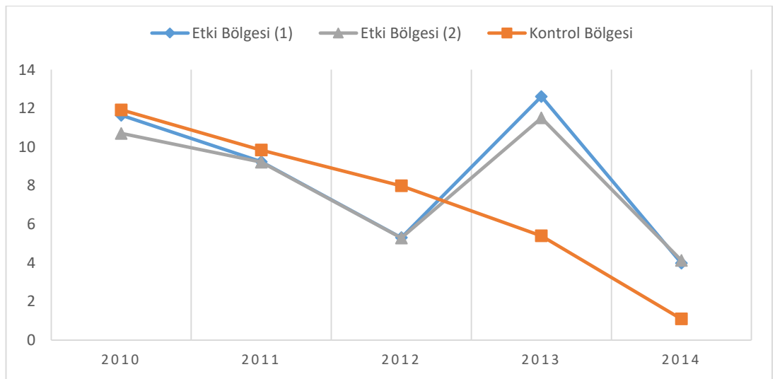
Grafik 3. 2: Etki ve kontrol grubunun göç öncesi/sonrası ortalama büyüme oranı
