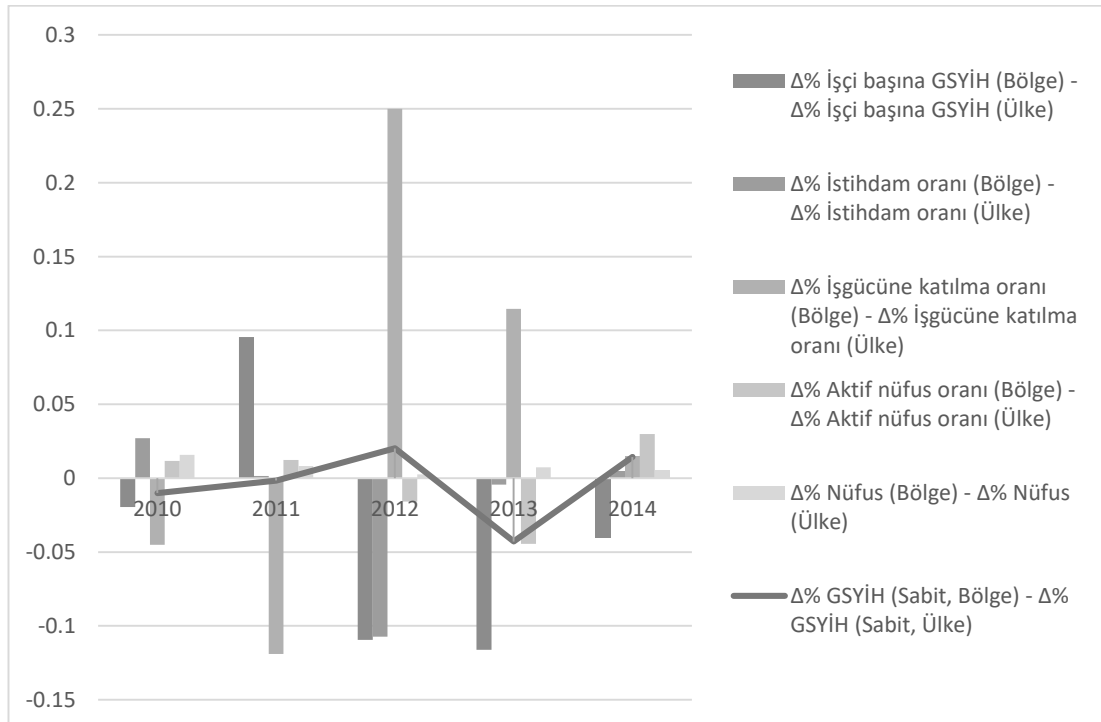
Grafik 3. 7: Şanlıurfa, Diyarbakır (TRC2) bölgesinin bölgesel kıyaslama sonuçları
