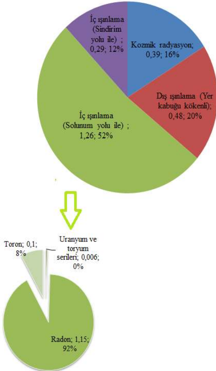
Grafik 2.1 Doğal radyoaktiviteden kaynaklanan ortalama yıllık etkin radyasyon doz dağılımı
