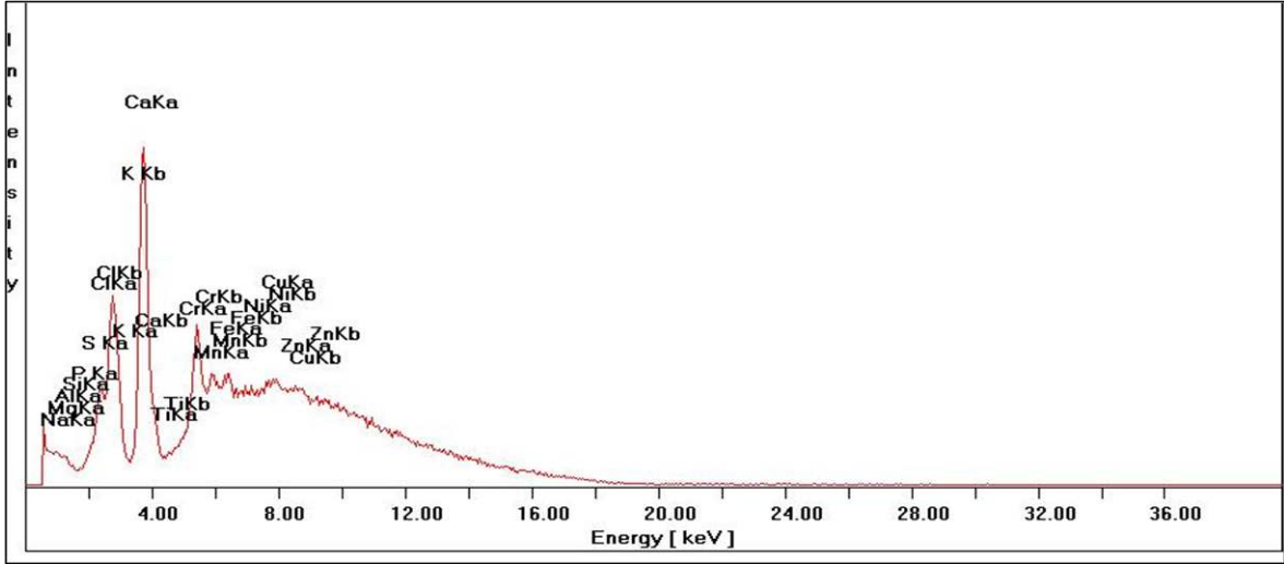
Sekil 3.6. Giljarovia tebenricosa erkek için XRF spektrometre ile ölçülmüş spektrum
