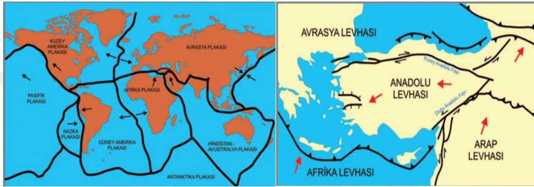
Şekil 2. Yerkabuğunu oluşturan ana levhalar, Anadolu Levhası ve hareket yönleri (Erdik, 2011)
