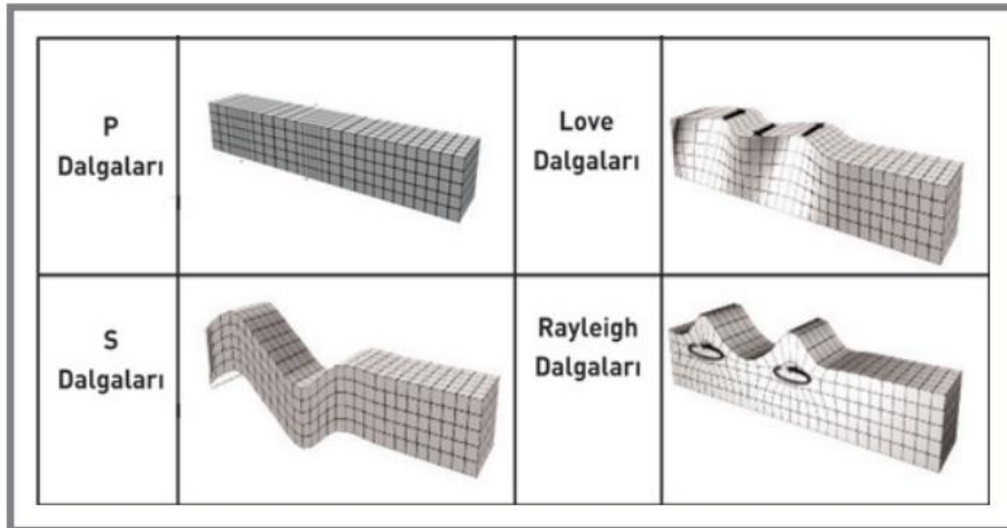
Şekil 5. Deprem dalgaları (Erdik, 2011)
