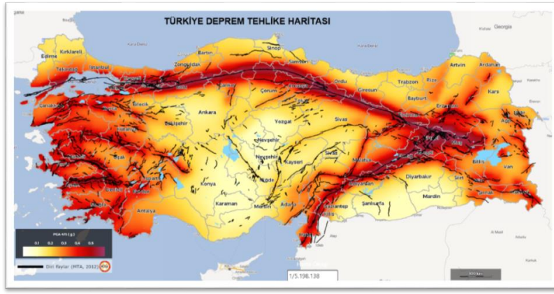
Şekil 3. Türkiye deprem tehlike haritası (AFAD, 2018)
