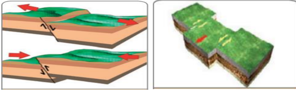
Şekil 4. Doğrultulu, normal ve ters faylanma (Erdik, 2011)
