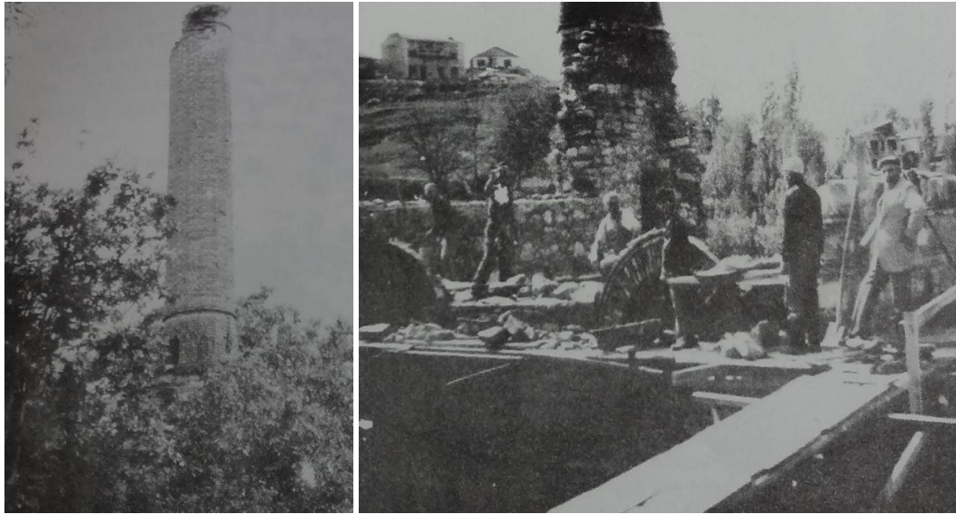
Şekil 7.89: Soldaki görselde Musa Baba Camii onarım öncesi yıkık minaresi, sağdaki görselde ise onarım için yapılan kazı çalışması görülmektedir. (Bursa Eski Eserleri Sevenler Kurumu Hizmet Albümü, 1985)
