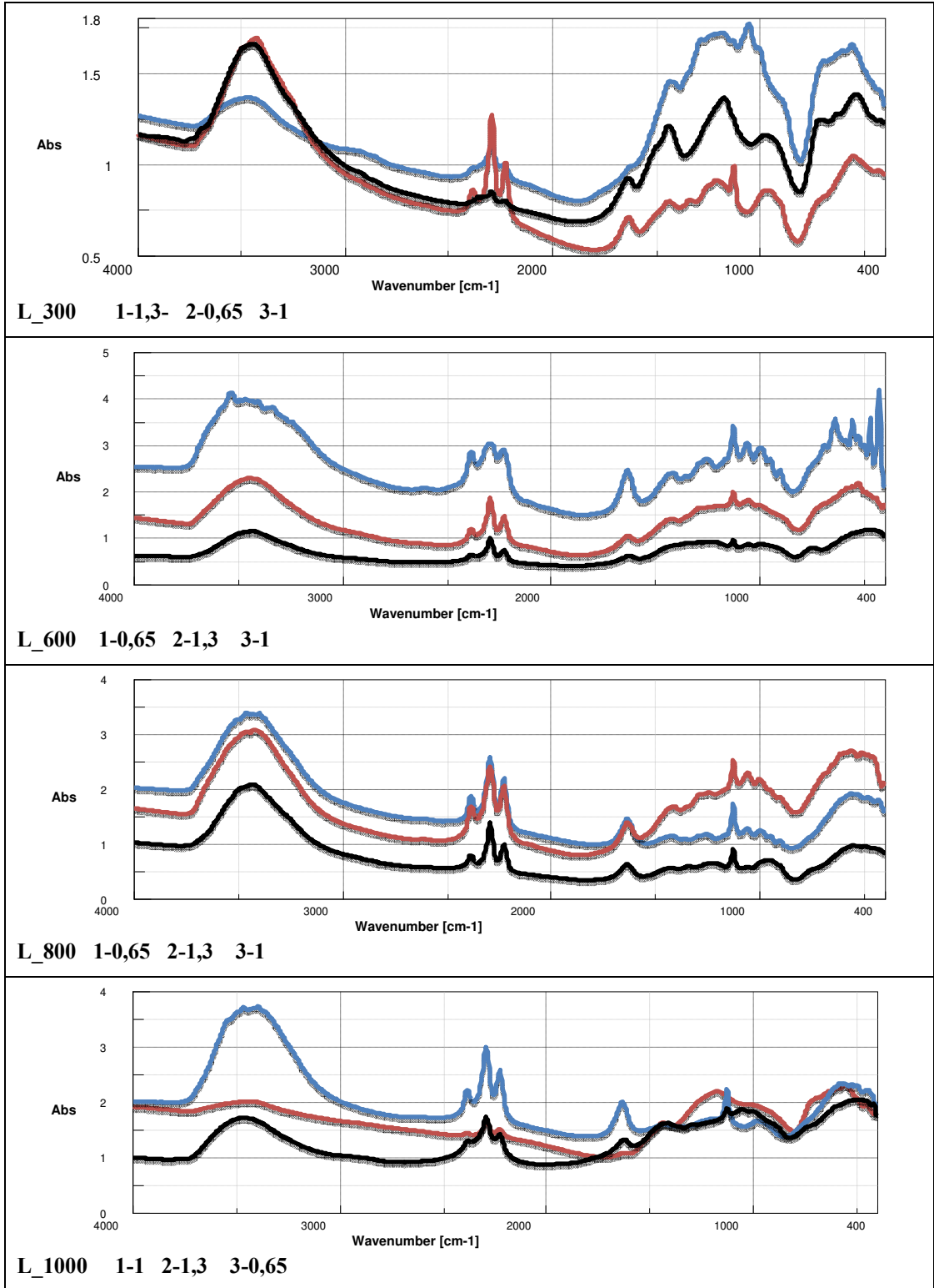
Şekil 4.39. LiBO 2 FT/IR incelemesi. a) LiBO 2 300 dakika reaksiyon sonucu FTIR incelemesi, b) LiBO 2 600 dakika reaksiyon sonucu FTIR incelemesi. c) LiBO 2 800 dakika reaksiyon sonucu FTIR incelemesi. d) LiBO 2 1000 dakika reaksiyon sonucu FTIR incelemesi
