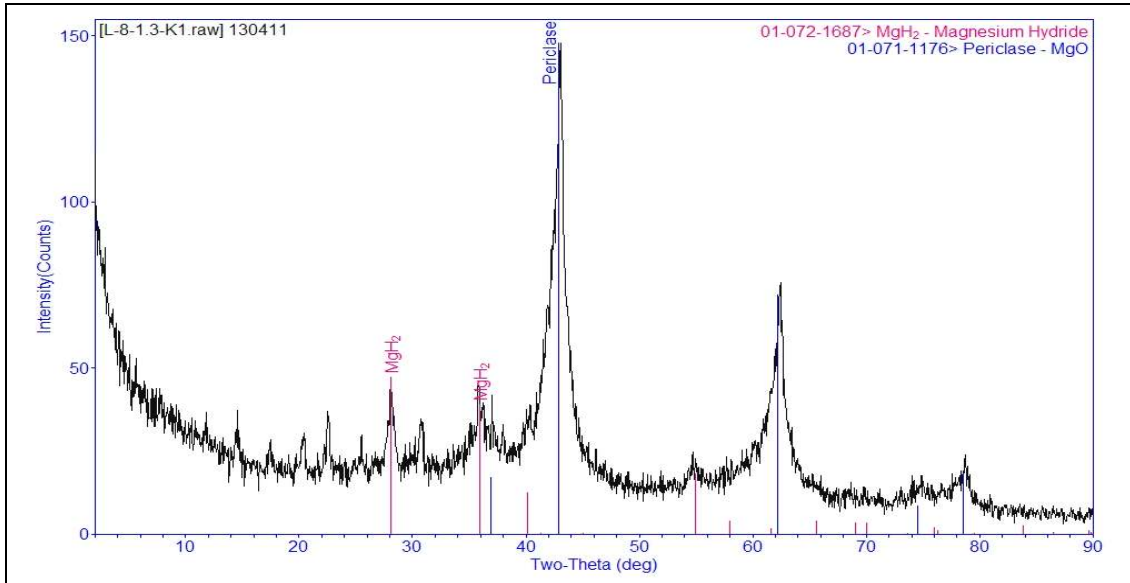
Şekil 4.46. LiBO 2 ile başlanan reaksiyonda oluşan yan ürünün XRD grafiği
