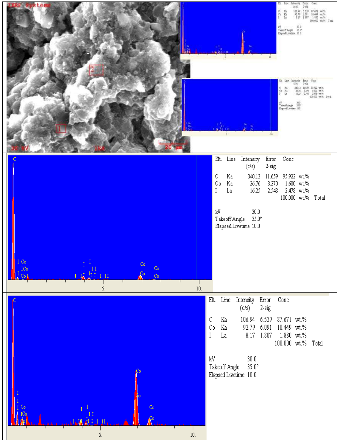
Şekil 4.16. % 40 \text{CoI}_2 katalizör 300 deneme sonrası EDS incelemeleri
