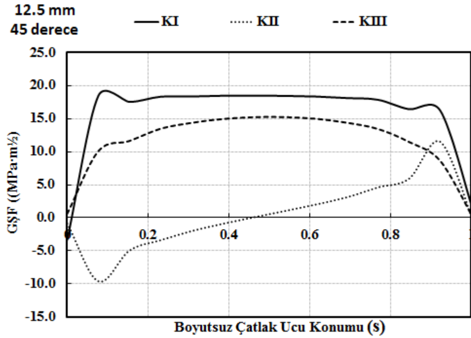
Şekil 3.28. CTT numunesinin \theta=45^\circ , P=10 kN ve t=12,5 mm için gerilme şiddet faktörleri
