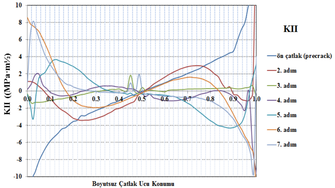
Şekil 4.30. İlerleyen çatlağın her bir adımındaki çatlak ucu boyunca KII gerilme şiddet faktörleri dağılımı.
