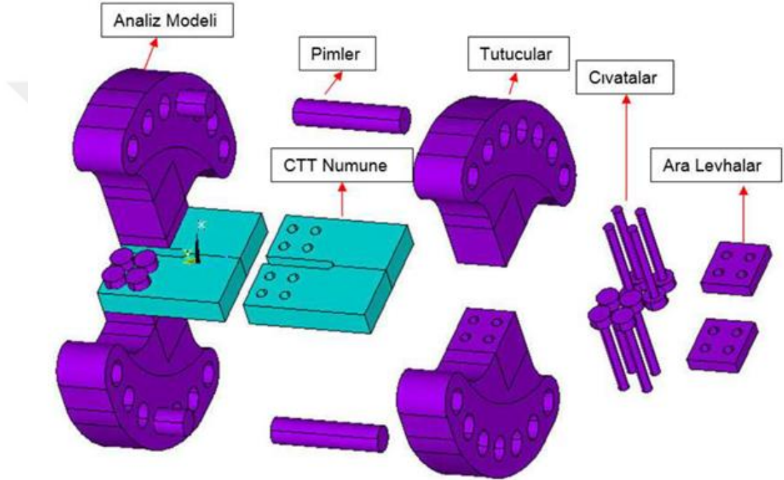
Şekil 3.5. Analiz modeli detay resmi
