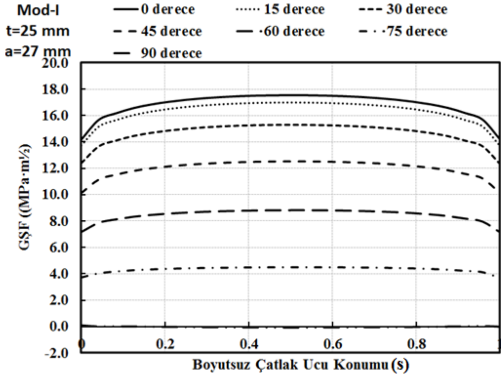
Şekil 3.39. CTT numunesinin P=10 kN, t=25 mm ve 27 mm çatlak uzunluğu için 7 farklı yükleme açısında Mod-I gerilme şiddet faktörleri
