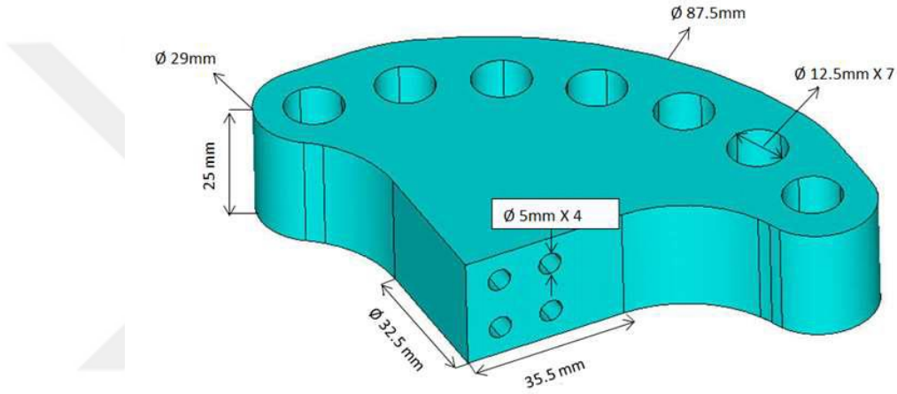
Şekil 3.2. CTT deney numune tutucusu boyutları.
