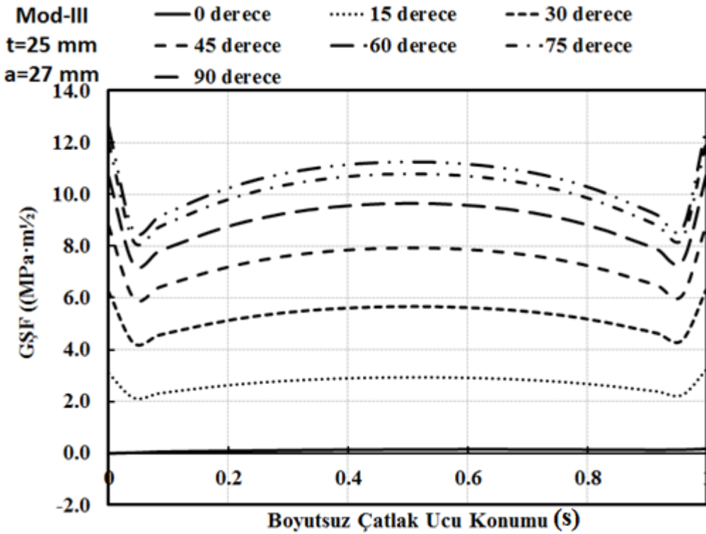
Şekil 3.41. CTT numunesinin P=10\text{ kN} , t=25\text{ mm} ve 27\text{ mm} çatlak uzunluğu için 7 farklı yükleme açısında Mod-III gerilme şiddet faktörleri
