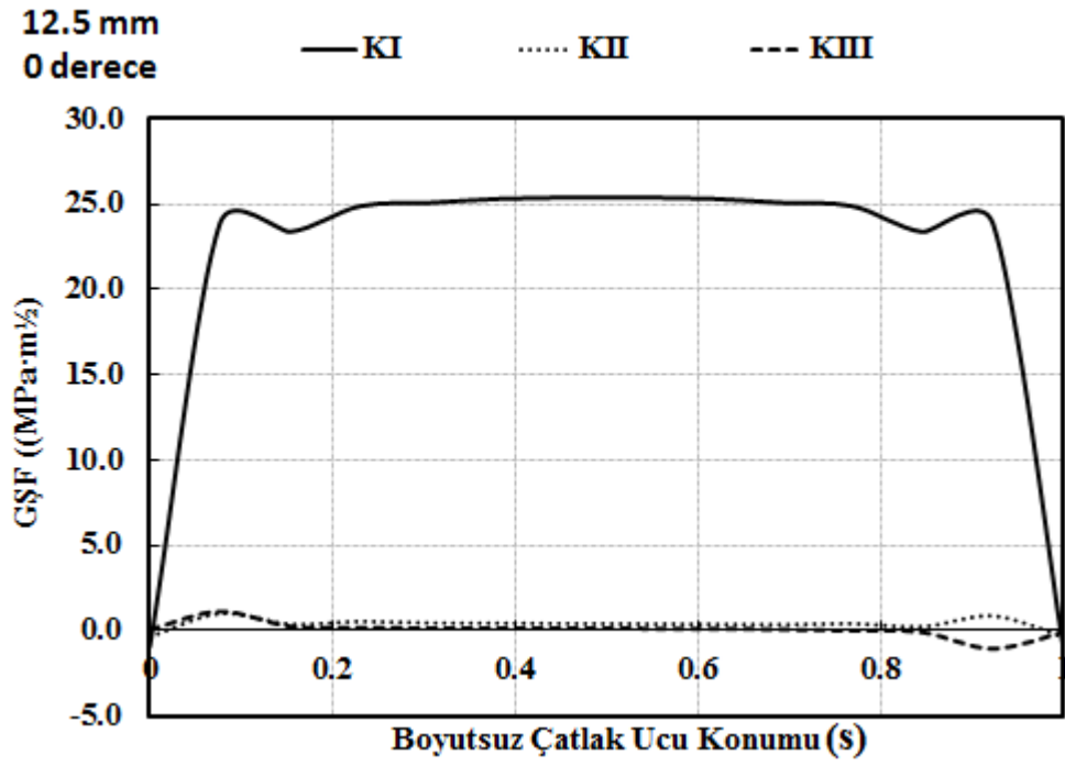
Şekil 3.27. CTT numunesinin \theta=0^\circ , P=10 kN ve t=12,5 mm için gerilme şiddet faktörleri
