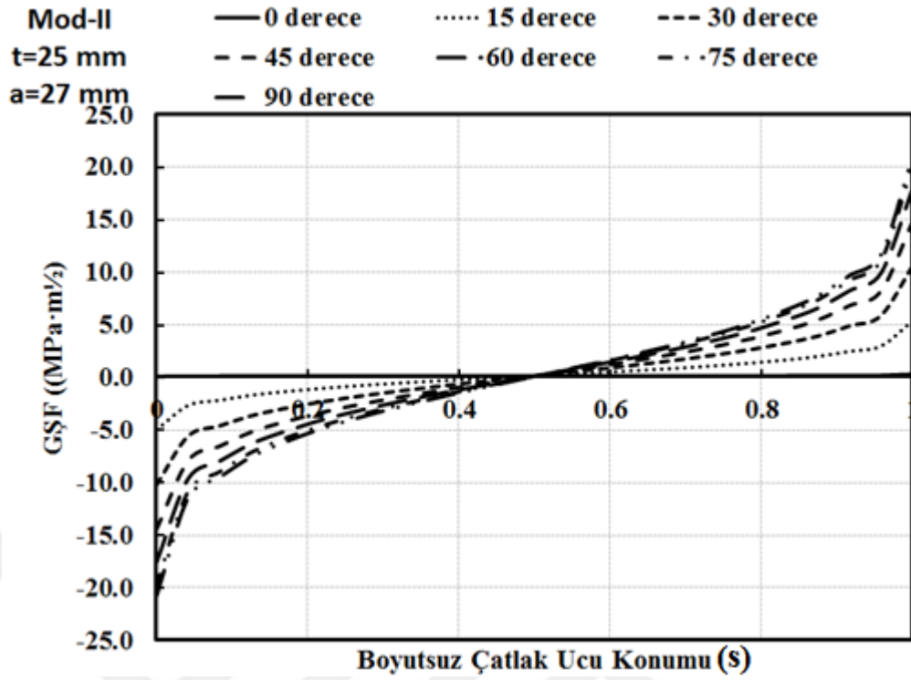
Şekil 3.40. CTT numunesinin P=10\text{ kN} , t=25\text{ mm} ve 27\text{ mm} çatlak uzunluğu için 7 farklı yükleme açısında Mod-II gerilme şiddet faktörleri
