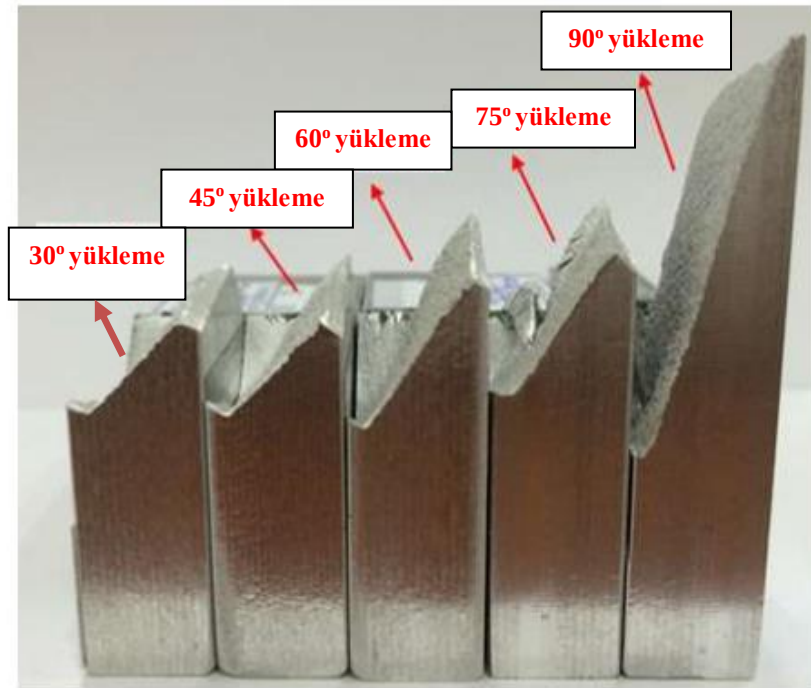
Şekil 4.21. Farklı açılarda yapılan da/dN testlerinden elde edilen kırılma yüzeyleri (sırt görünüş) [10].
