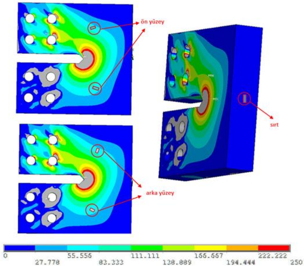
Şekil 4.6. \theta = 45^\circ Mod-I/III yüklemesinde 6 kN yüklemeye gerçekleştirilen gerilme analizi sonrası numune oluşun 1. asal gerilmeler ve strain-gagelerin yerleştirildiği yerler.
