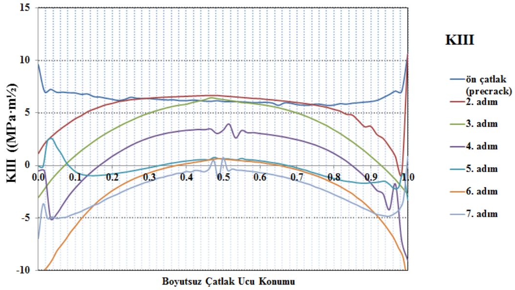
Şekil 4.31. İlerleyen çatlakın her bir adımındaki çatlak ucu boyunca KIII gerilme şiddet faktörleri dağılımı
