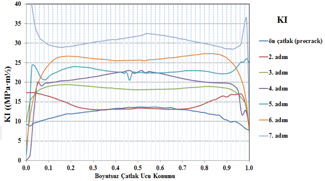
Şekil 4.29. İlerleyen çatlağın her bir adımındaki çatlak ucu boyunca KI gerilme şiddet faktörleri dağılımı.
