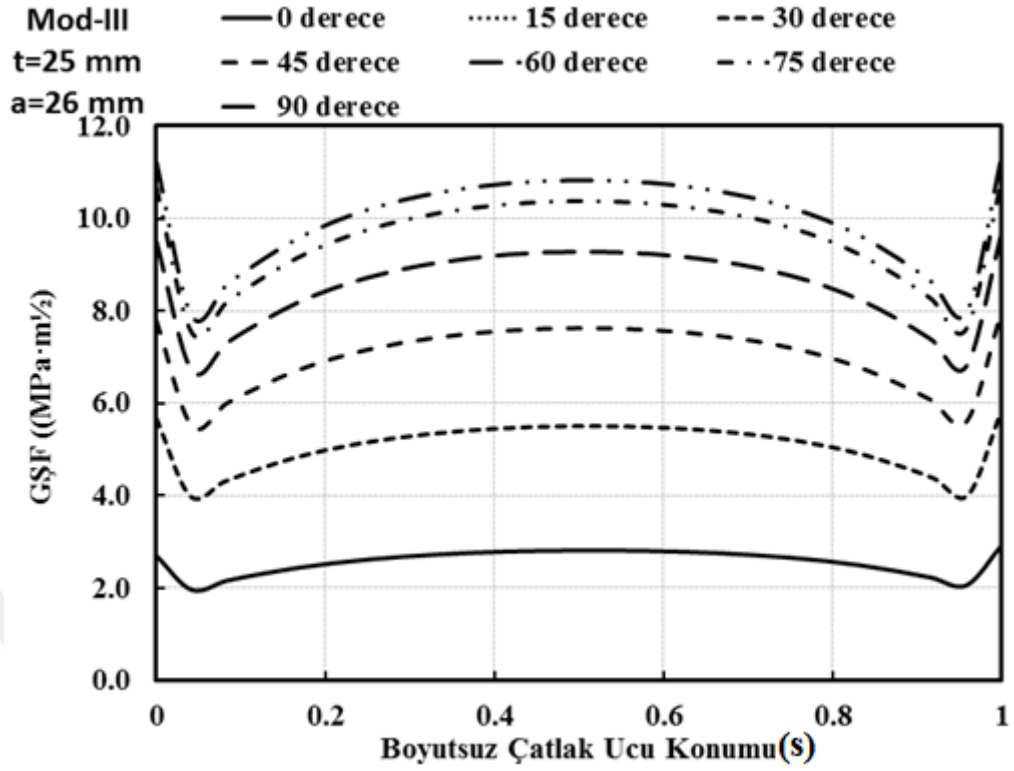
Şekil 3.38. CTT numunesinin P=10 kN, t=25 mm ve 26 mm çatlak uzunluğu için 7 farklı yükleme açısında Mod-III gerilme şiddet faktörleri
