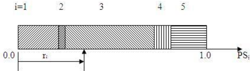
Şekil 5.5. Rulet çarkı seçim operatörünün uygulandığı [26]
