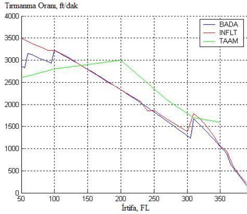
Şekil 2.7. Tırmanma oranının karşılaştırılması [2]
