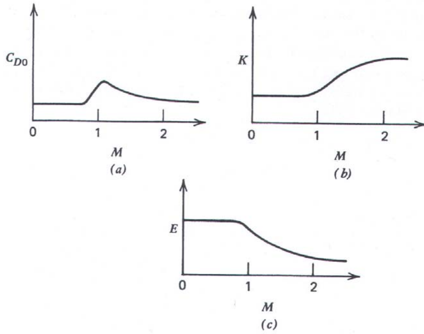
Şekil 4.5. Mach sayısının bir fonksiyonu olarak aerodinamik karakteristiklerin değişimi a) sıfır taşıma (minimum) sürüklenme katsayısı b) indüklenmiş sürüklenme parametresi c) finess [14].
