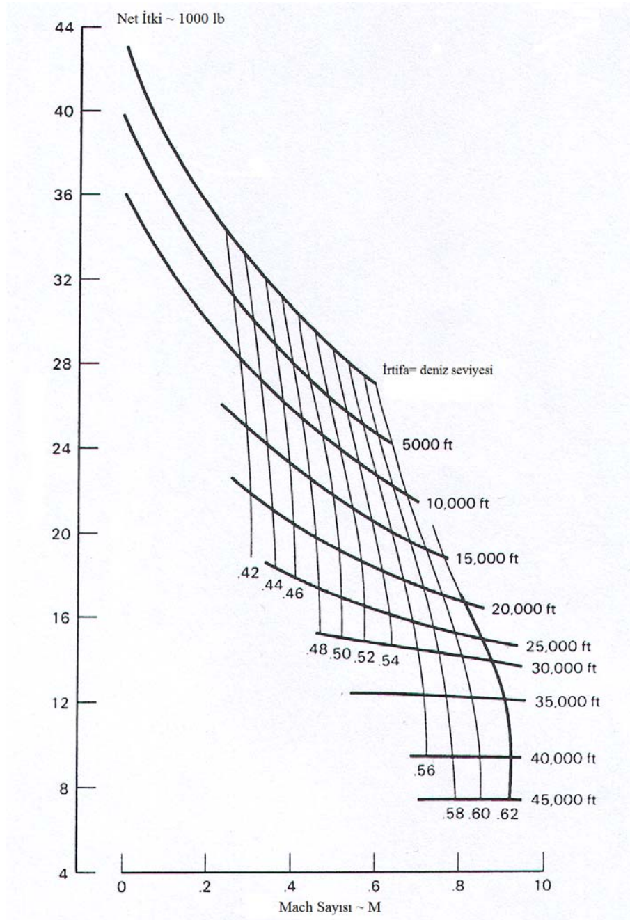
Şekil 3.10. PW 4056 turbofan motoru için maksimum seyahat itkisi [16]
