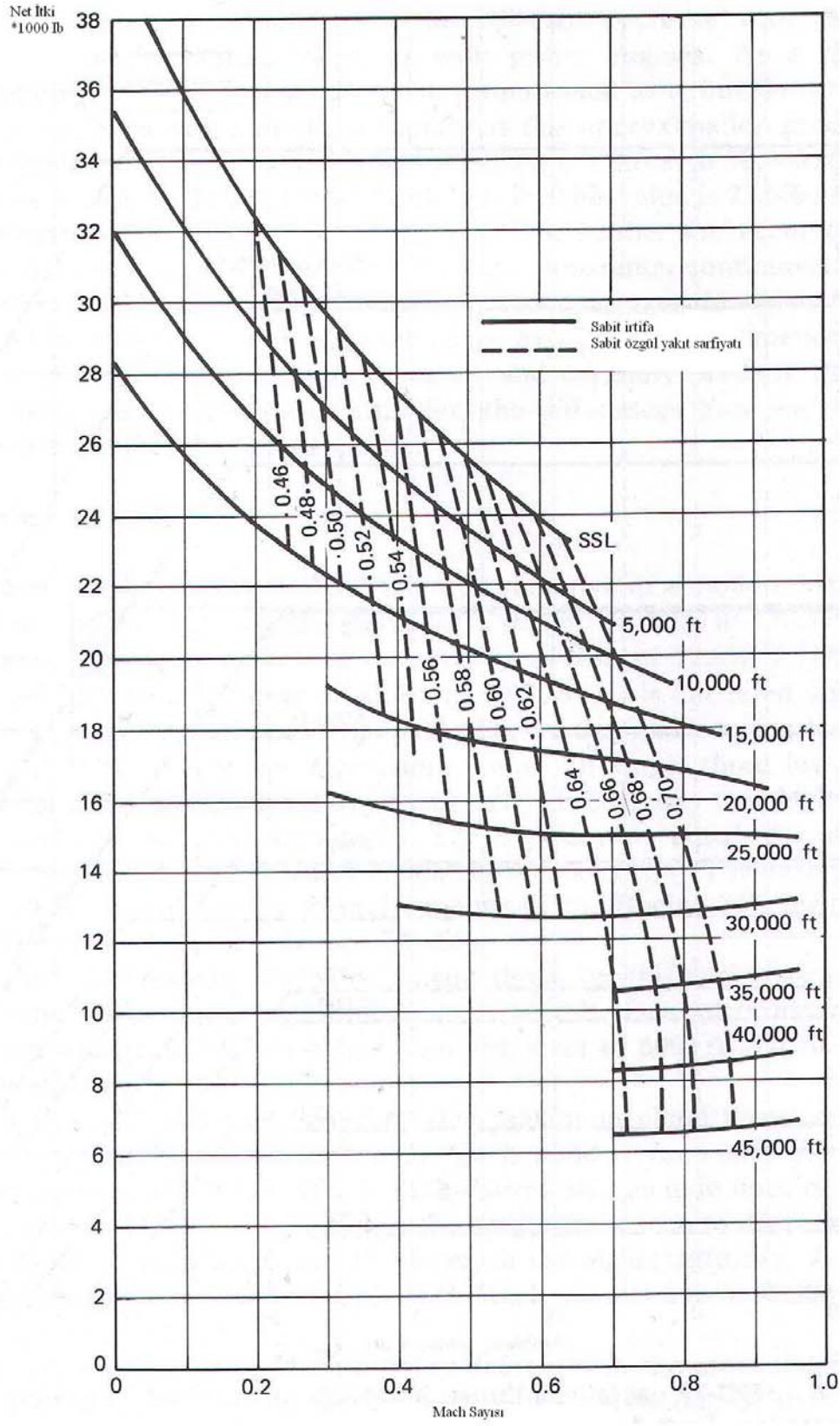
Şekil 6.1. JT9D-7A maksimum tırmanma itkisi (100% ram iyileştirmesi, bleed havası yok, güç kaybı yok) [30]
