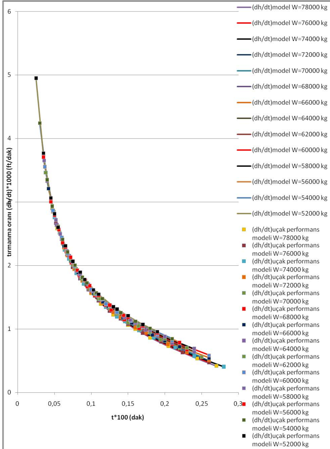
Şekil 8.9. Tırmanma oranı modeli (dh/dt)_{\text{model}} değerleri ile tırmanma oranı uçak performans modeli ((dh/dt)_{\text{uçak performans modeli}}) değerlerinin karşılaştırılması
