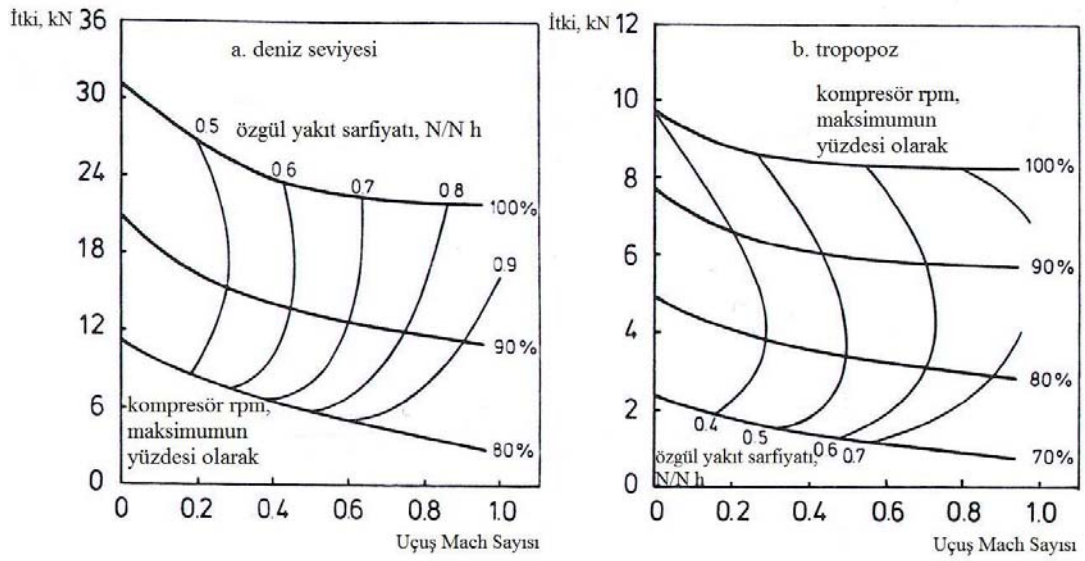
Şekil 3.7. Tipik turbofan motoru performansı [13]
