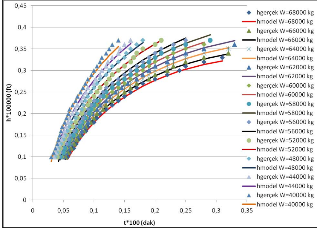
Şekil 7.1. Tırmanma sürelerine karşılık gerçek irtifa ( h_{\text{gerçek}} ) değerleri ile irtifa modeli ( h_{\text{model}} ) değerlerinin karşılaştırılması
