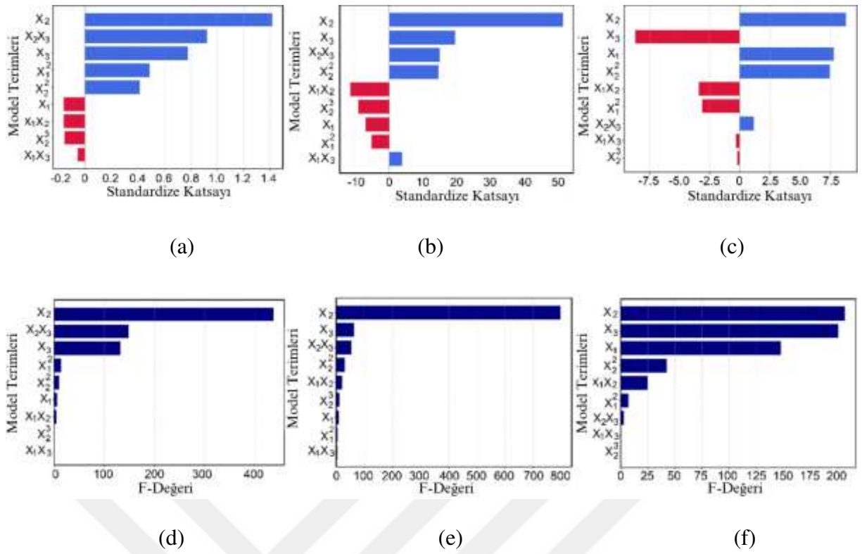
Şekil 72: Modellerin Parametre Etkileri (a) UCS Modelinin Standardize Regresyon Katsayısı Değişimi, (b) CO2 Ayak İzi Modelinin Standardize Regresyon Katsayısı Değişimi, (c) Maliyet Modelinin Standardize Regresyon Katsayısı Değişimi, (d) UCS Modelinin F-Değer Tabanlı Pareto Diyagramı
