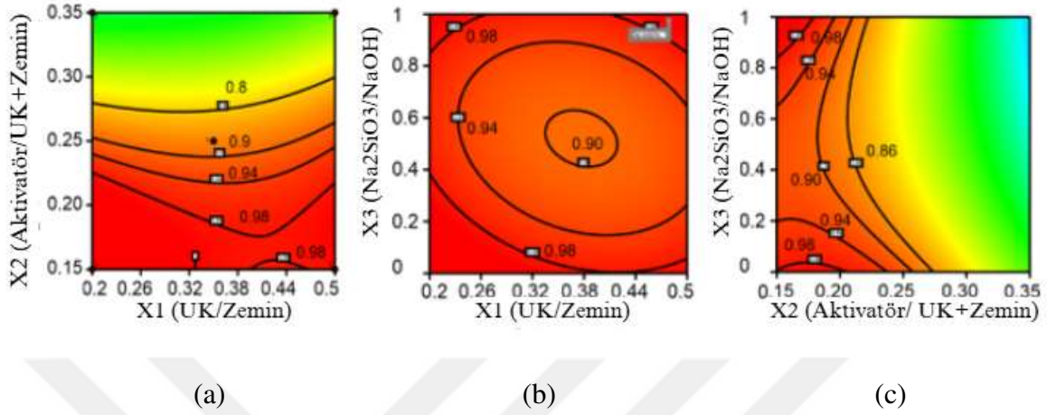
Şekil 74: CO 2 Salınımını En Aza İndirmeye Dayalı Tek Nesneli Optimizasyon Sonuçlarının Kontur Çizimi, Talebe Dayalı Etkileşim Etkilerini Göstermektedir (a) Uçucu Kül İçeriği ve Aktivatör İçeriği, (b) Uçucu Kül İçeriği ve Sodyum Silikat İçeriği, (c) Aktivatör İçeriği ve Sodyum Silikat İçeriği
