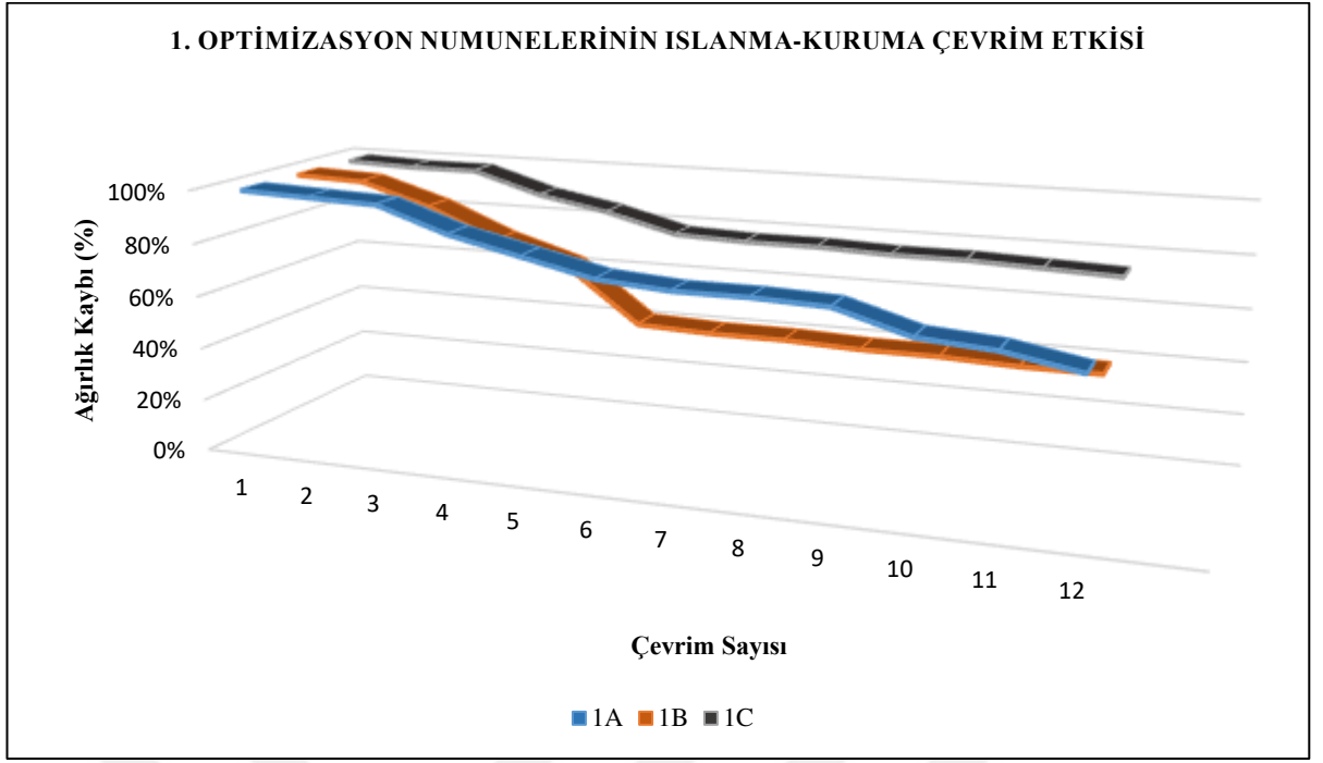
Şekil 65: 1. Optimizasyon Zemin Numunelerinin Islanma Kuruma Çevrim Etkisi
