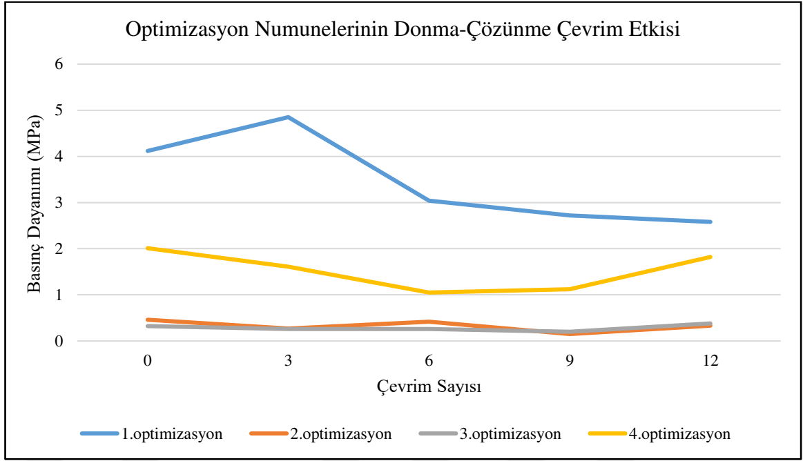
Şekil 63: Optimizasyon Numunelerinin Farklı Donma-Çözünme Çevrim Etkisi
