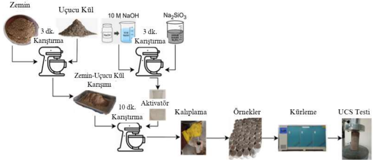
Şekil 16: Numune Hazırlama Prosedürü
