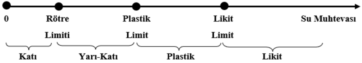
Şekil 12: Kıvam Limitlerinin Belirlenmesi
