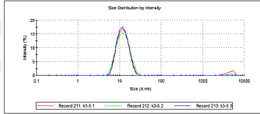
Şekil E3. (K3 serisi) 3:7 oranında kişniş uçucu yağı:Tween 20 içeren emülsiyonların stabilite çalışmaları öncesi zeta boyut analizlerinin spektrumları
