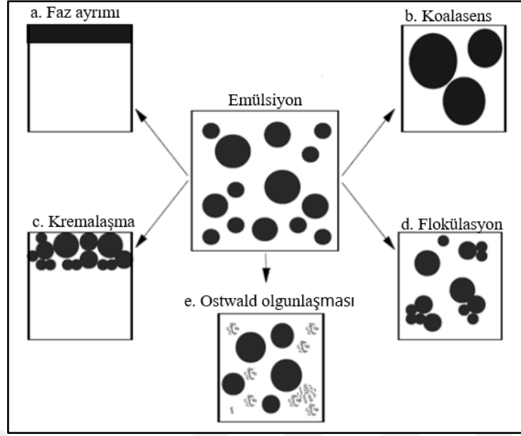
Şekil 1.5. Emülsiyonlarda destabilizasyon çeşitleri; a) Faz ayrımı, b) Koalesens, c) Kremalaşma, d) Flokülasyon, e) Ostwald olgunlaşması (Robins, 2000).
