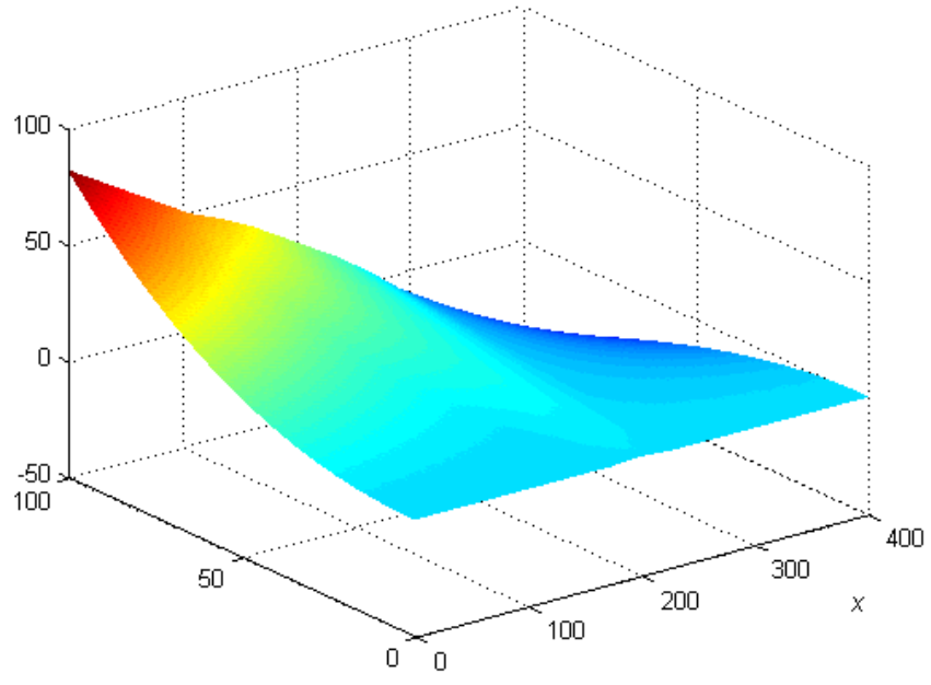
Şekil 1.1 (1.15) çözümünün grafiği
