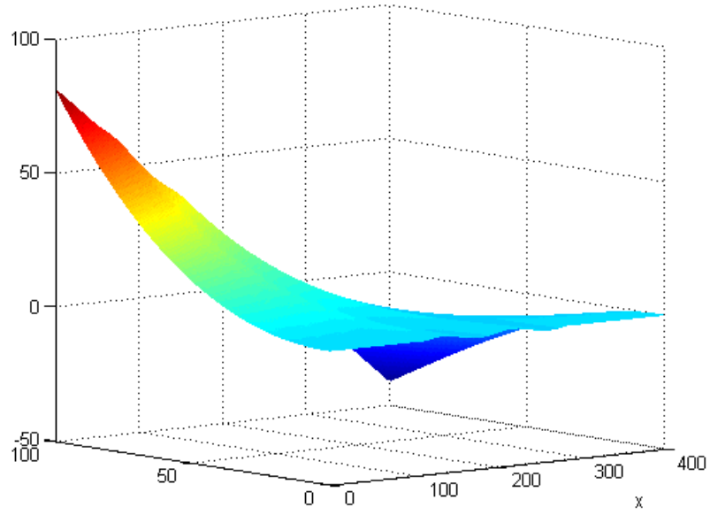
Şekil 1.2 (1.15) çözümünün grafiği
