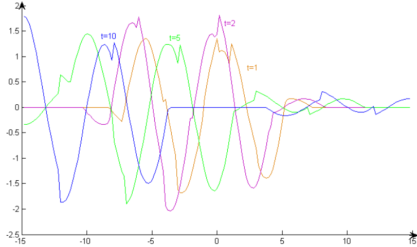
Şekil 2.12 (2.16) formülü ile elde edilen çözüm ( \phi_2(x) = c > 0 durumu)
