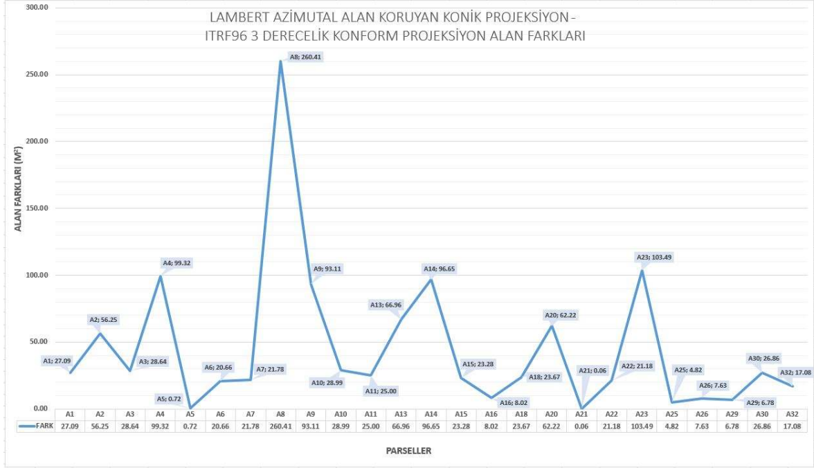
Şekil 29. Lambert Azimuthal AKK projeksiyon ve ITRF96 3 derecelik konform projeksiyon alan farkları
