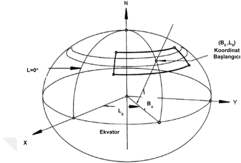
Şekil 9. Lambert Konform Konik (LKK) projeksiyonu
