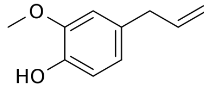
Öjenol
