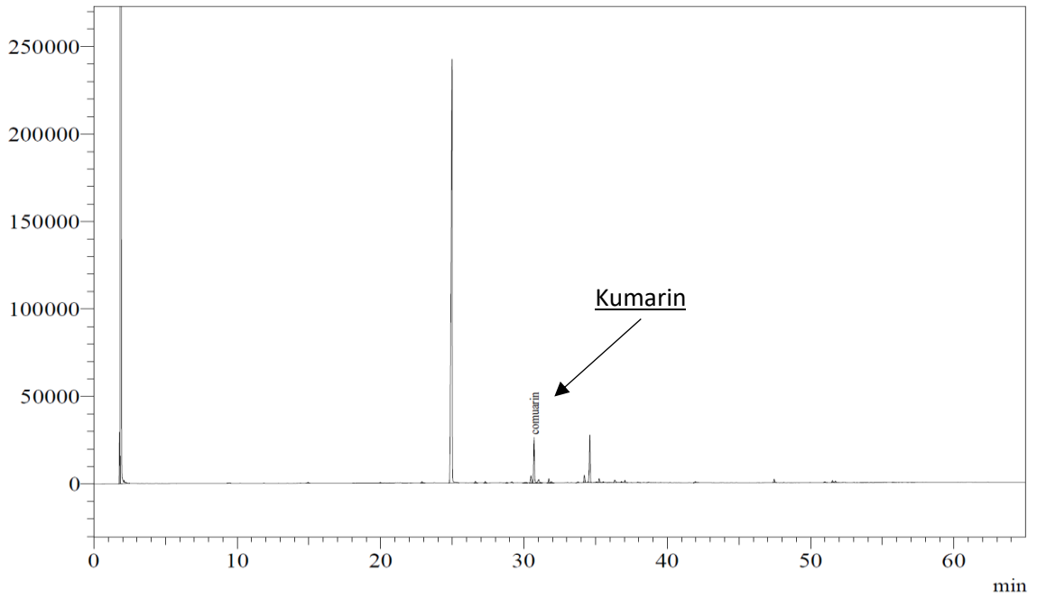
Şekil 4.2. 22 nolu tarçın numunesinden elde edilen GK-AID kromatogramı
