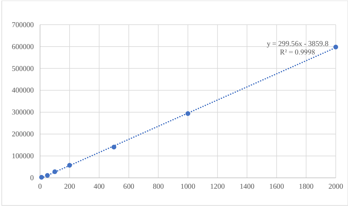
Şekil 3.3. Kalibrasyon grafiğı (GK/AİD)
