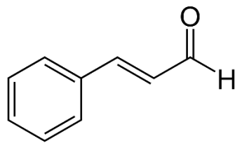
Sinnamaldehyt
