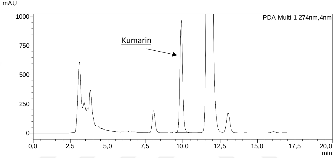
Şekil 4.1. 22 nolu tarçın numunesinden elde edilen YPSK kromatogramı
