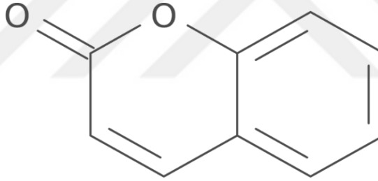
Şekil 2.2. Kumarin
