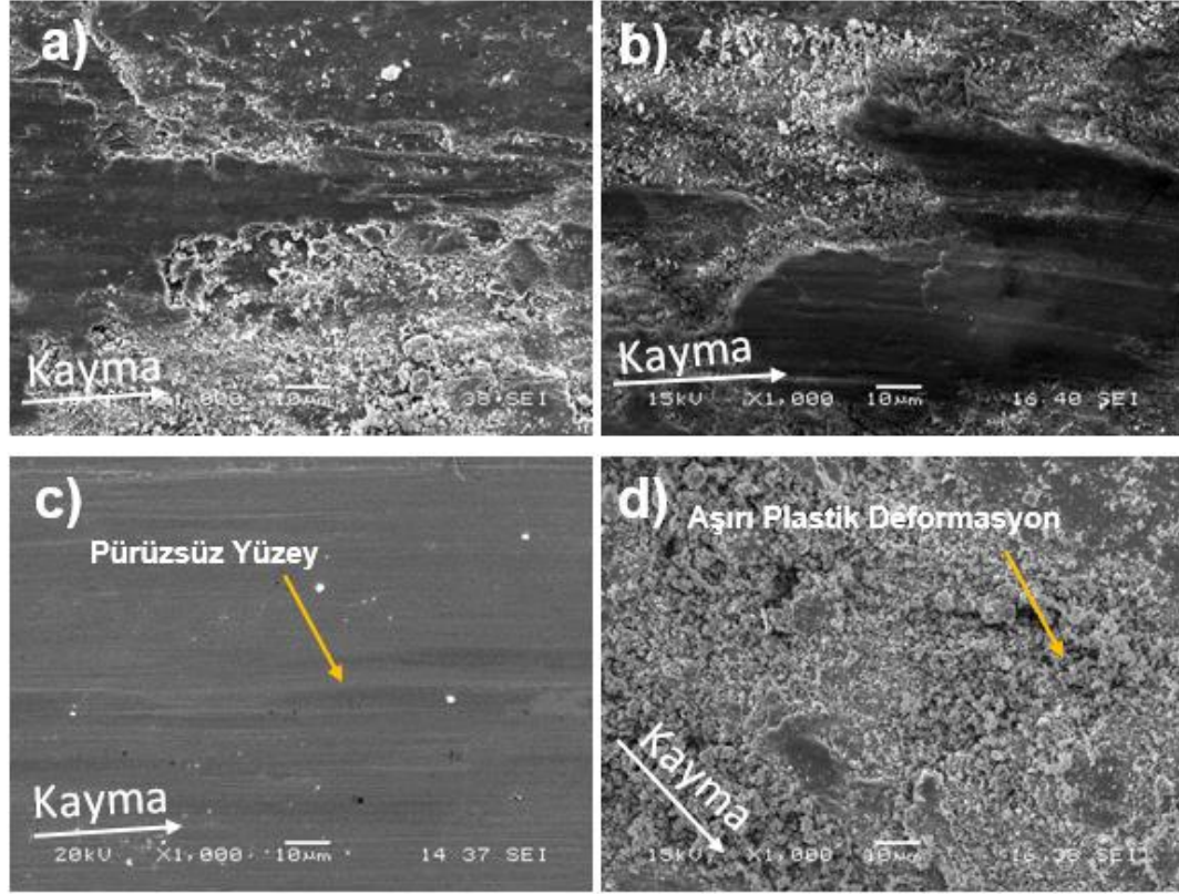
Şekil 4.12. 300 °C'de test edilen kaplamaların aşınmış yüzeyinin SEM mikrografları a) NiW5 b) NiW75W c) NiW50W d) NiW40
