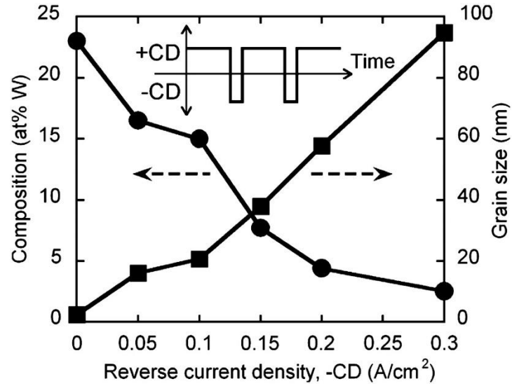
Şekil 2.6. Nanokristal Ni-W alaşımlarının kimyasal bileşimi ve tane boyutu üzerindeki ters akım etkileri. Dalga formu, 20 mS süreli ve 20 A\ dm^{-2} yoğunluktaki katodik yönde kesikli ve ardından 3 mS ters akımı içerir [130].
