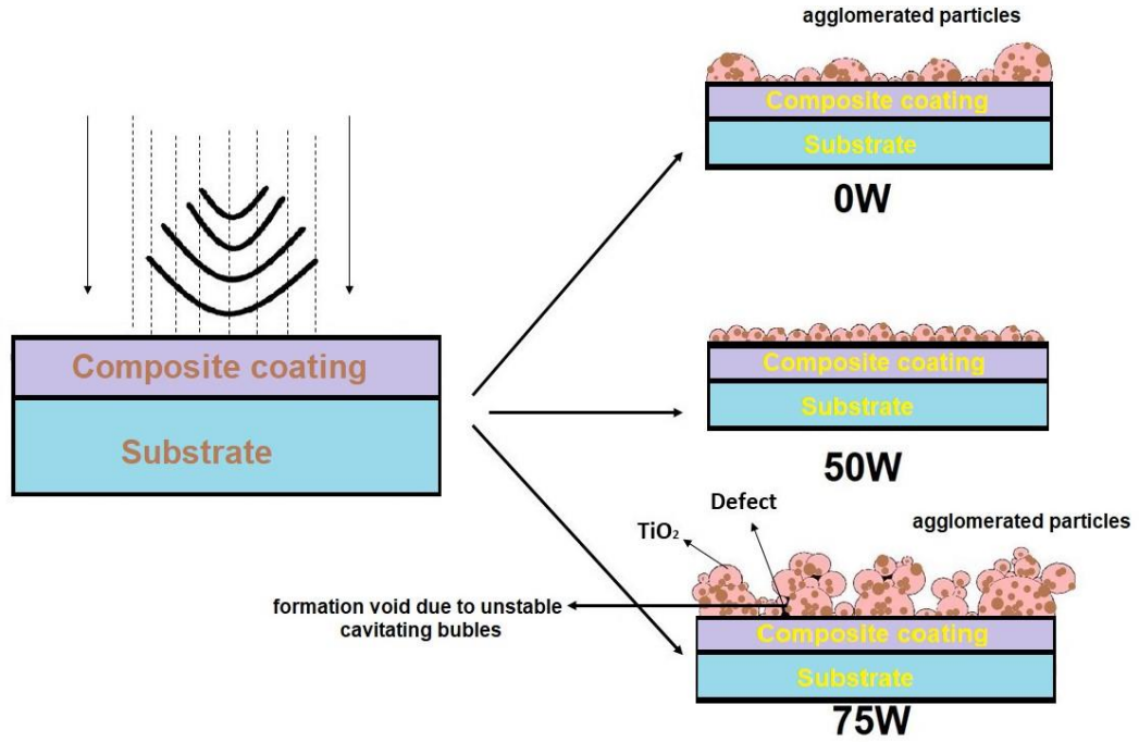
Şekil 4.3. Kaplama çözeltisinde \text{TiO}_2 parçacıklarının dağılma mekanizması
