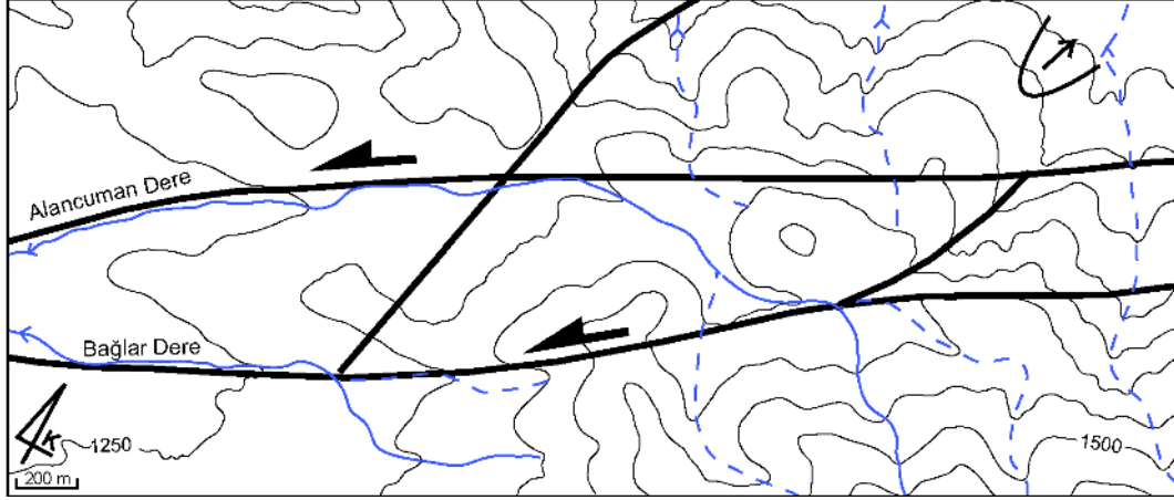
Şekil 33. Faylar boyunca gözlenen sol yanal ötelenmeler
