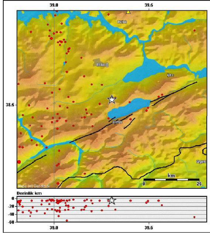
Şekil 34. Uluova Fay Zonu'nda meydana gelen 28. 12. 2005 Mollakendi depremi
