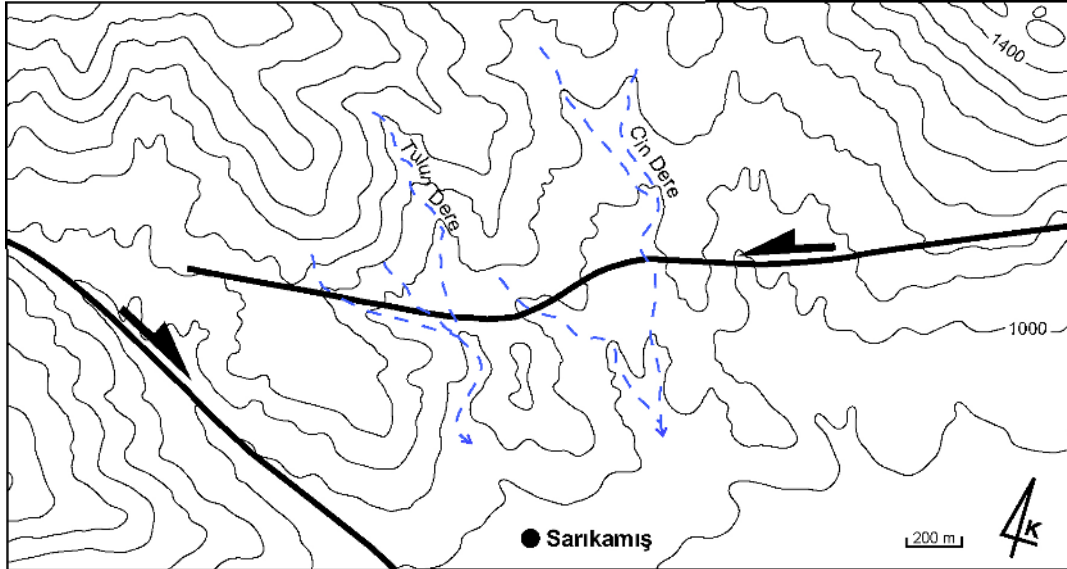
Şekil 28. Cin ve Tulun derelerde gözlenen sol yanall bükülmeler
