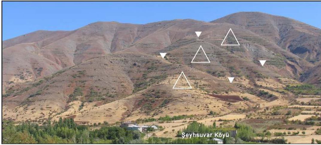
Şekil 25. Antitetik sağ yanallı doğrultu atımlı faylar boyunca gelişen üçgen yüzeyler (Şeyhsuvar D. su, Bakış GD)
