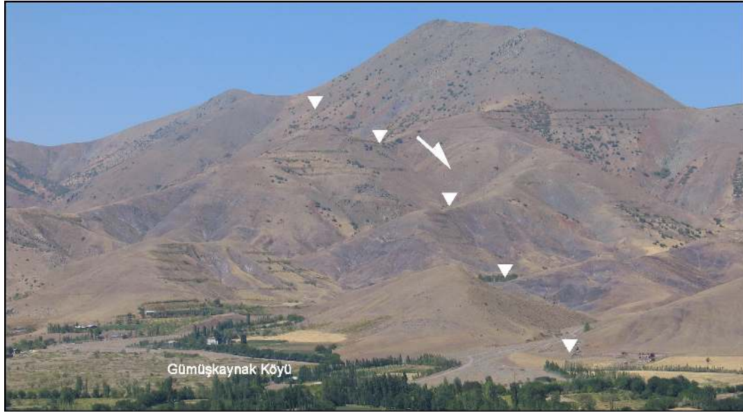
Şekil 11. Uluova Fay Zonu'na ait sağ yanal eşlenik fay örneği (Bakış K)
