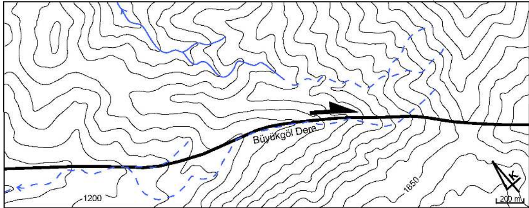
Şekil 30. Büyüköl Dere'de gözlenen sağ yanal bükülmeler
