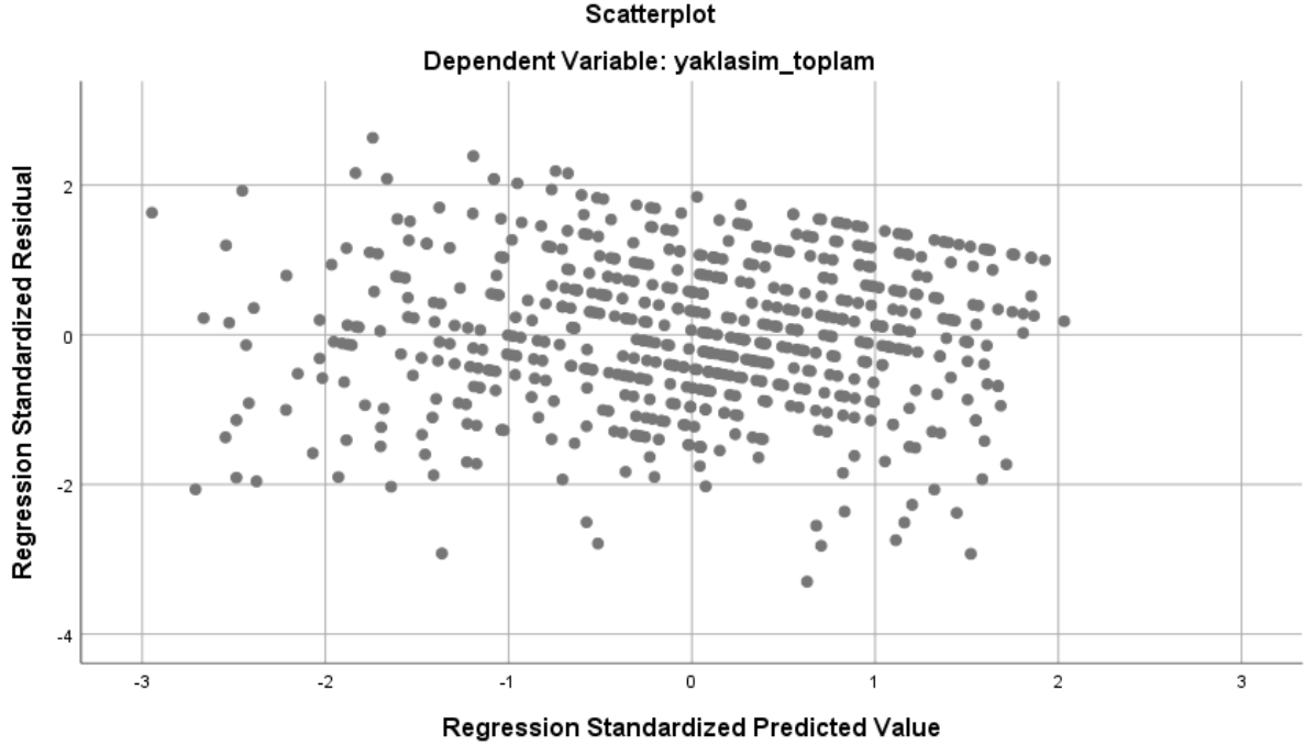
Şekil 3.6. Regresyon Modeli İçin Artıkların (Rezidüellerin) Saçıntı Grafiği (Bağımlı Değişken=Yaklaşım)
