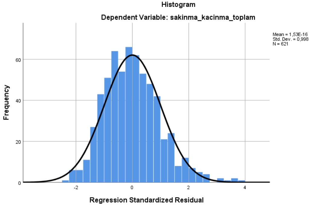
Şekil 3.10. Standardize Edilmiş Artıkların (Rezidiüellerin) Histogramı (Bağımlı Değişken=Sakınma Kaçınma)
