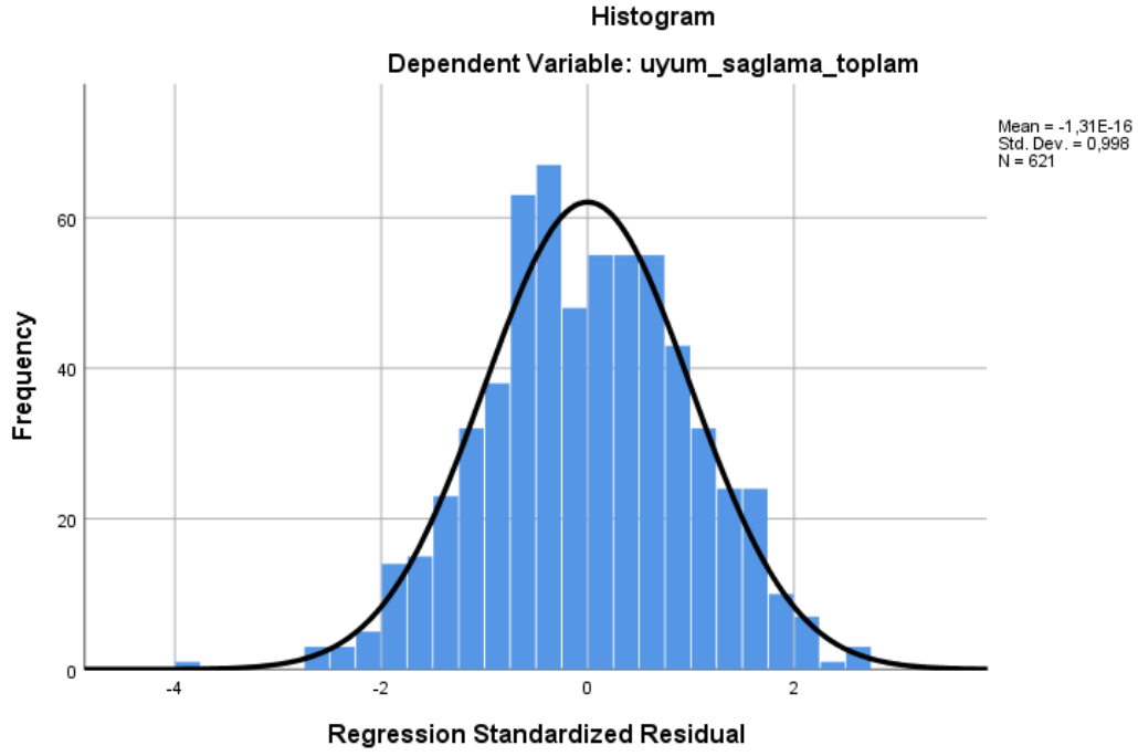
Şekil 3.7. Standardize Edilmiş Artıkların (Rezidüellerin) Histogramı (Bağımlı Değişken=Uyum Sağlama)
