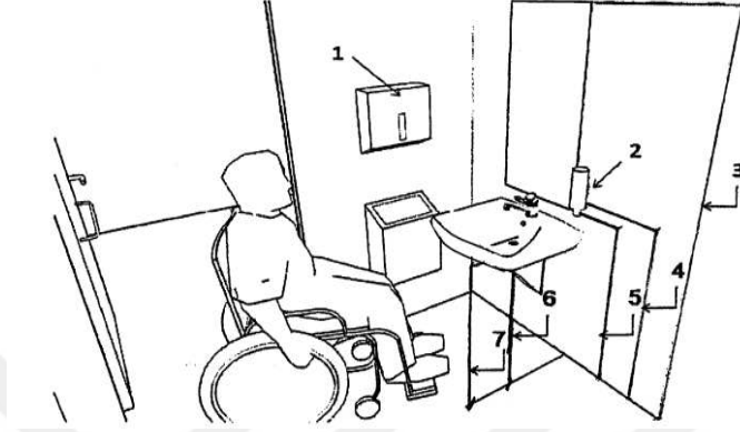
Şekil 14. Lavabo Ölçüleri
