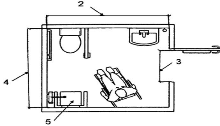
Şekil 15. Banyo Ölçüleri
