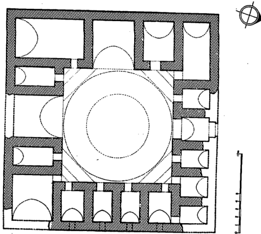
Şekil 4.22. Yağıbasan Medresesi (Çukur Medrese) Planı (Kuran, 1968)
