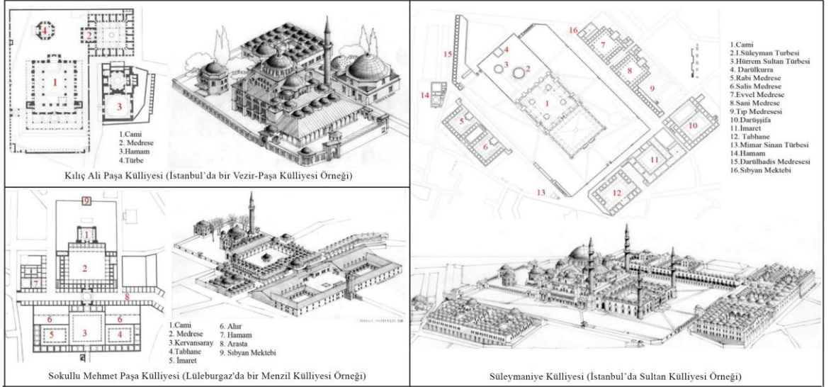
Şekil 4.20. Kılıç Ali Paşa Külliyesi, Sokullu Mehmet Paşa Külliyesi ve Süleymaniye Külliyesi plan ve görünüşleri (Necipoglu, 2005; akt. Sınnmaz, 2017)
