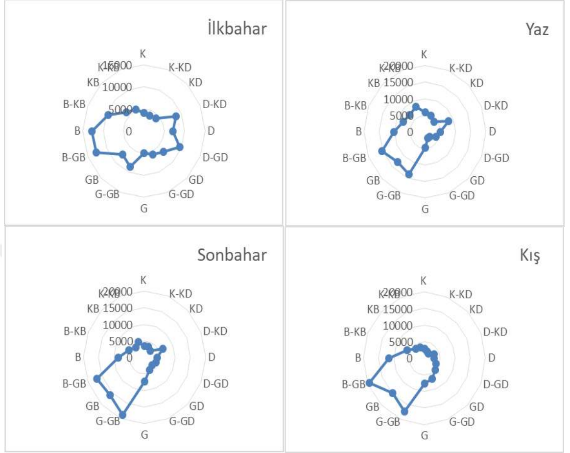
Şekil 2.2.20 :Ünye'nin mevsimlere ve yönlere göre yıllık ortalama rüzgar frekans gülü (1960-2016)
