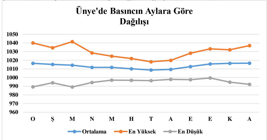
Şekil 2.2.18: Ünye'de basıncın aylara göre dağılışı
