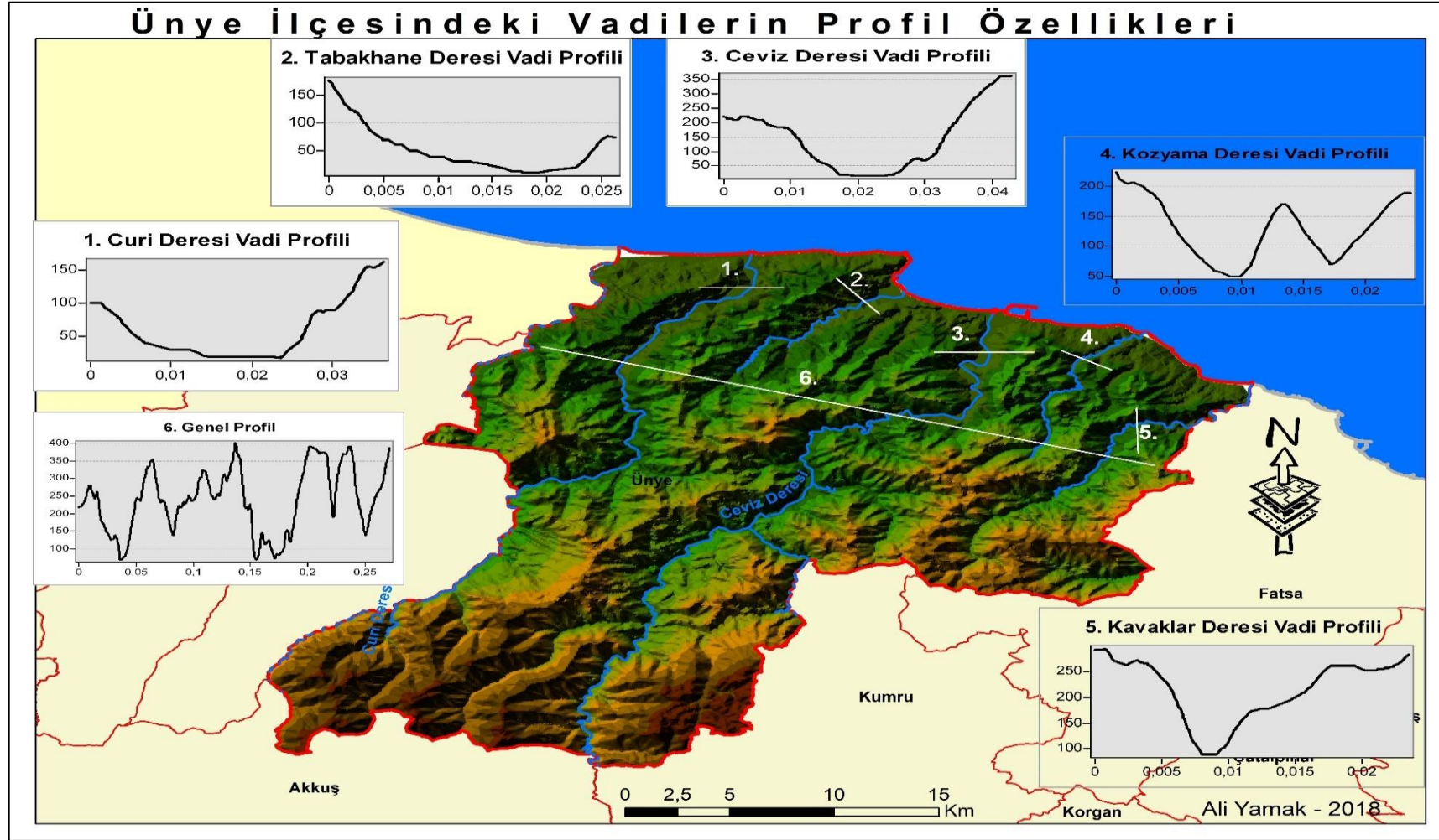
Şekil 2.2.9: Ünye ilçesindeki vadilerin profil özellikleri
