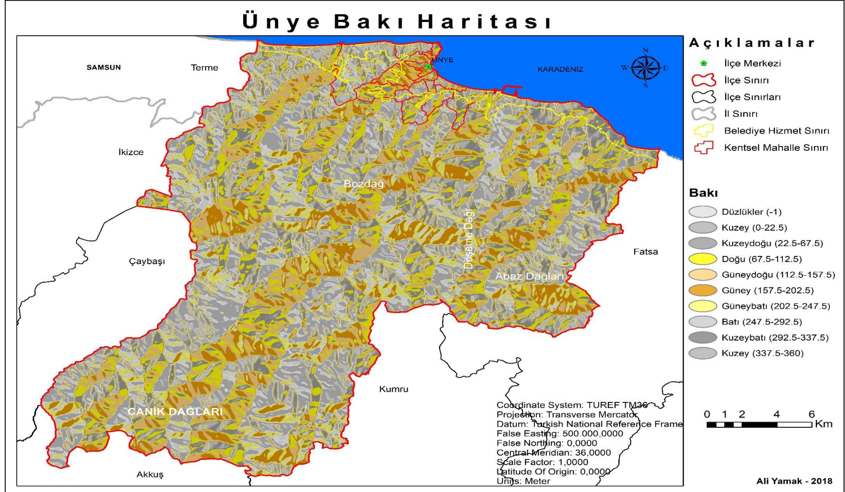
Şekil 2.2.13: Ünye'nin bakı durum haritası
