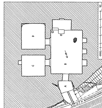
Şekil 11: Sangar Plan (Kleiss, 1968: 8).
