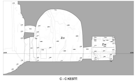
Şekil 9: Tuşpa-İç Kale ve Neft Kuyu Kaya Mezar Kesiti. (Sevin, 2012).
